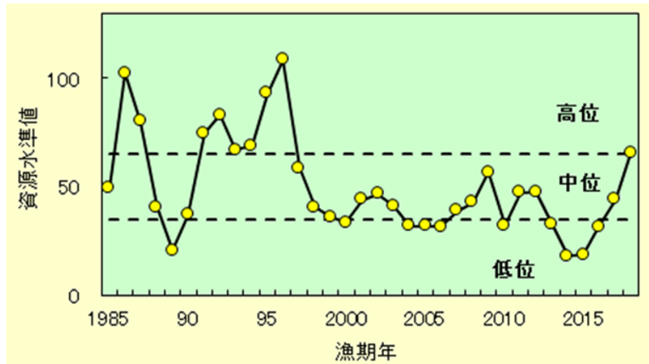
図2.1 根室海峡のマダラの資源水準値
