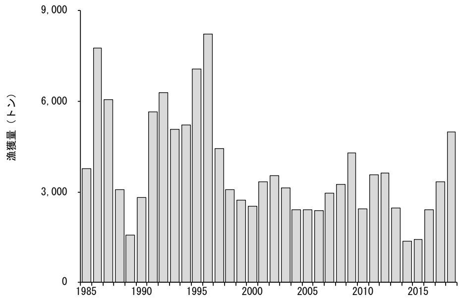
図1.2.2 根室海峡におけるマダラの漁獲量
