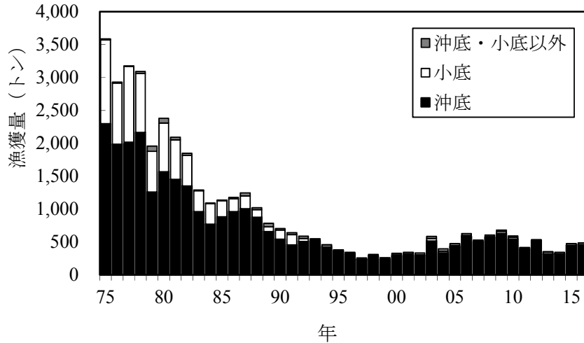
図5. 太平洋北部におけるキチジ漁獲量の推移
