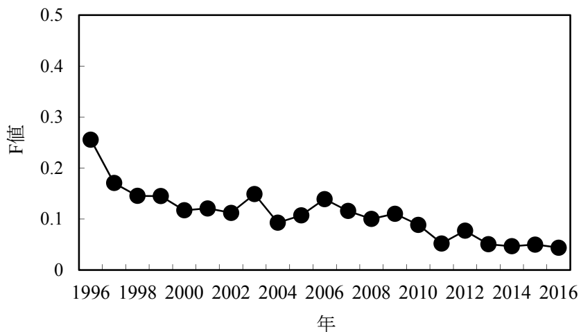
図12. F値の経年推移
