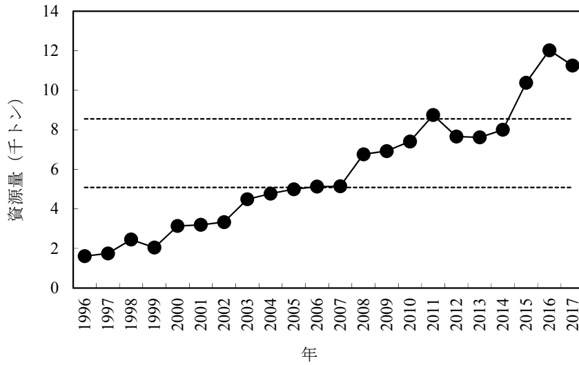
図16. キチジの資源量（1月時点）の推移 破線は水準の境界を示す。
