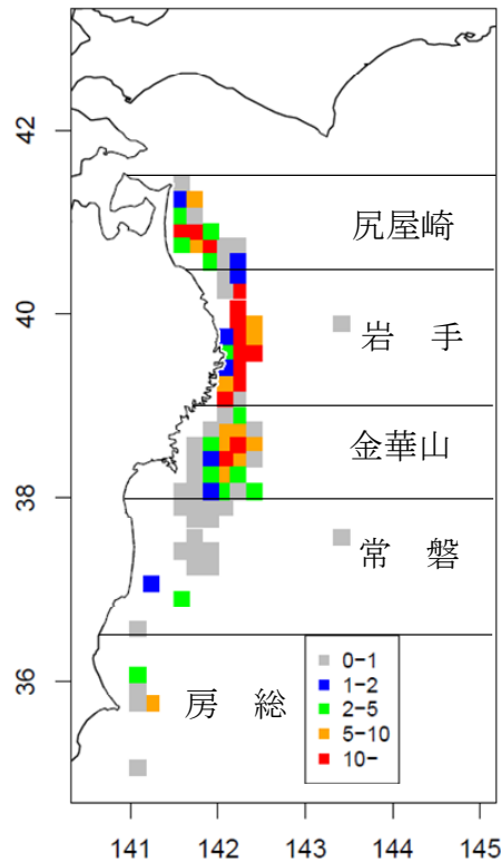
図4. 2015年の沖底によるキチジの漁場分布図 単位はトン。
