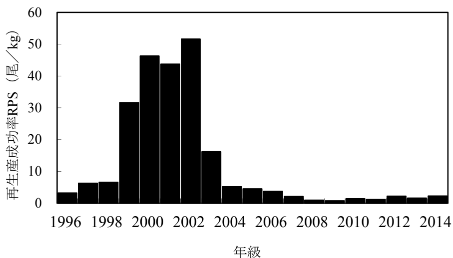
図13. 再生産成功率 (RPS) の推移 雌親魚1kgあたりの2歳魚尾数として計算。
