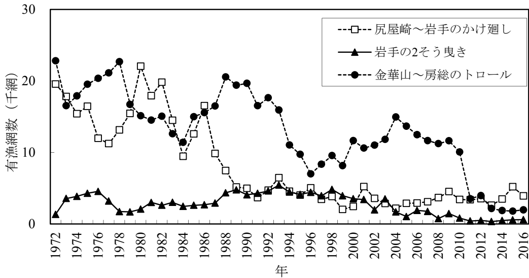
図6. 沖底による漁獲努力量の経年変化 2016年の値は暫定値。
