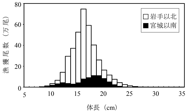
図9. 2016年の漁獲物の体長組成
