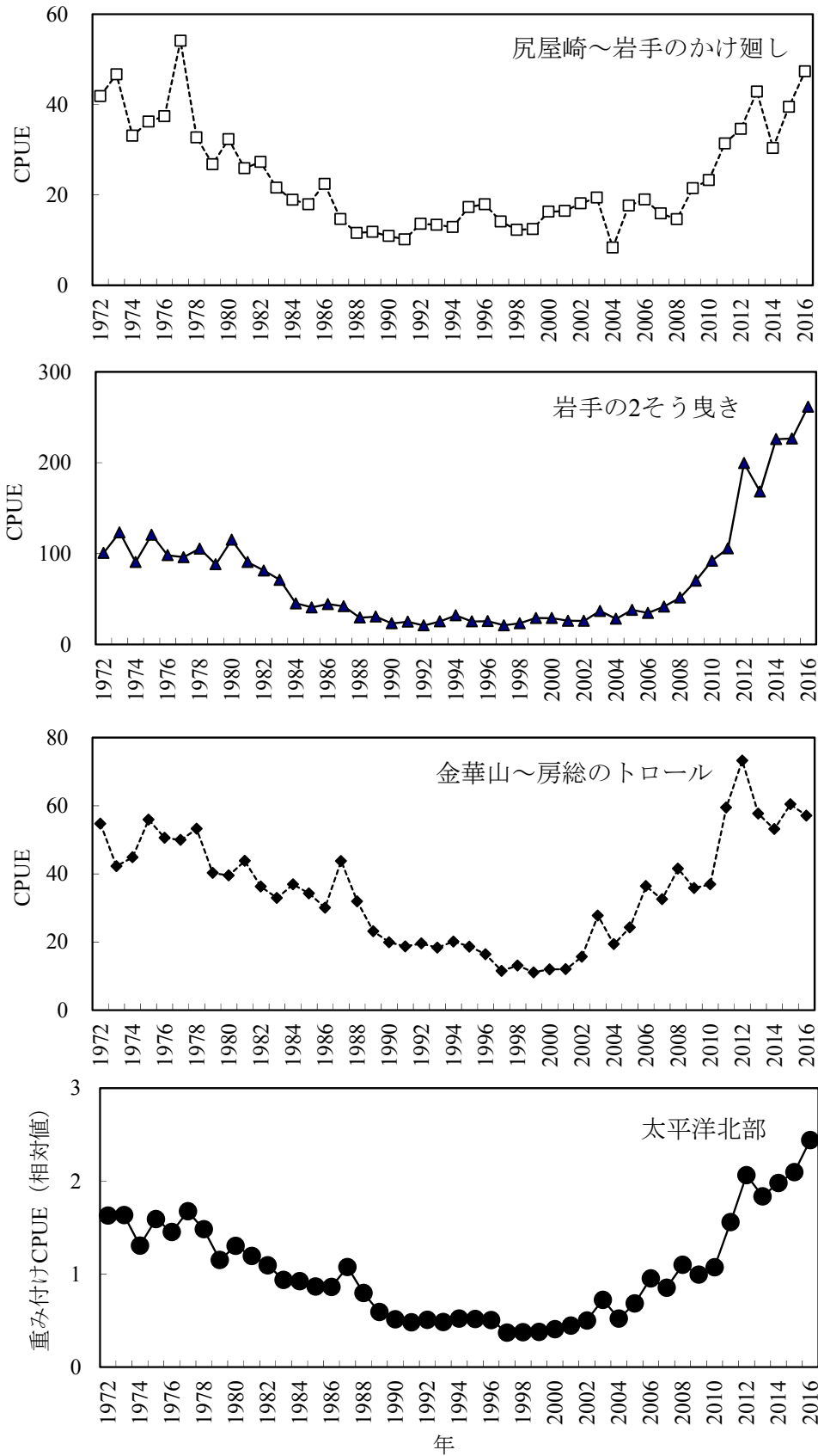
図8. 沖底によるCPUE (kg/網) および重み付けCPUE (相対値) の経年変化 2016年の値は暫定値。
