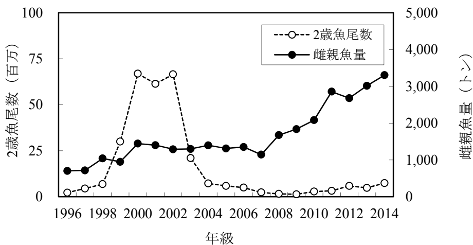
図14. 雌親魚量と加入量の推移
