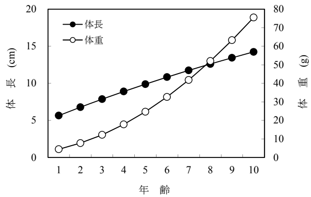
図2. 太平洋北部におけるキチジの成長
