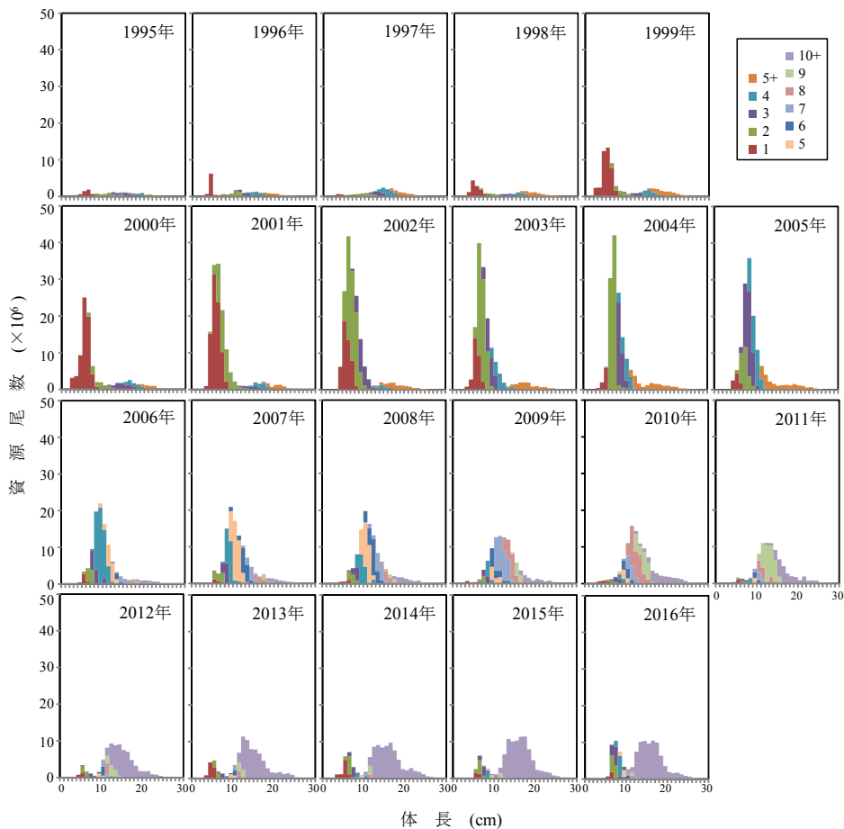
補足図3-2. Logistic式から得られた採集効率を用いた場合の資源の年齢別体長組成(10～11月時点)
