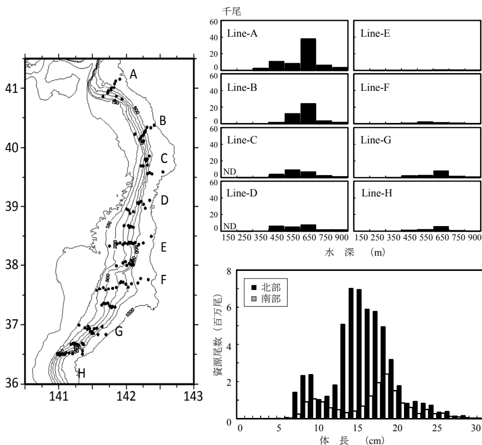
補足図3-1. 2016年10~11月の資源量調査における曳網地点(左)、キチジの分布密度(右上、曳網1km 2 あたり採集尾数で示す)および東北部・南部における体長組成(右下) ここでは、採集効率=1で一定とした。
