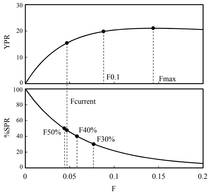
図17. 様々なFとYPR曲線および%SPR曲線との関係
