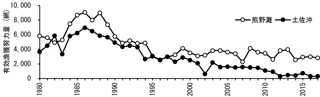
図4. 熊野灘と土佐沖における1そうびき沖底の有効漁獲努力量の経年変化
