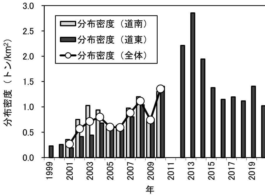
図4. 着底トロール調査によるキチジの分布密度推定値の推移
