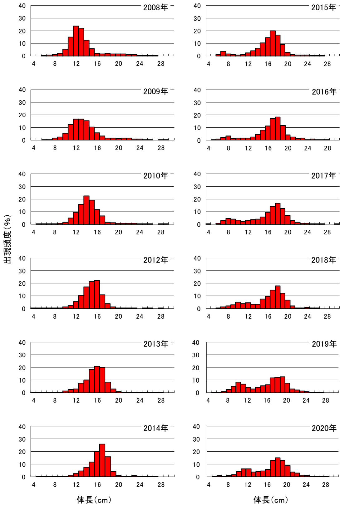
図 6. 着底トロール調査で採集されたキチジの体長組成 (2011 年は欠測)
