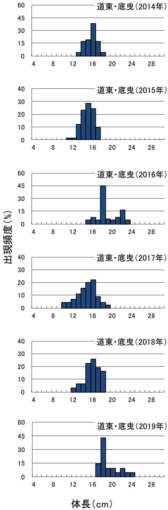
図 5. 道東海域におけるキチジ漁獲物の体長組成 (底曳は沖底とえびこぎ網を含む)
