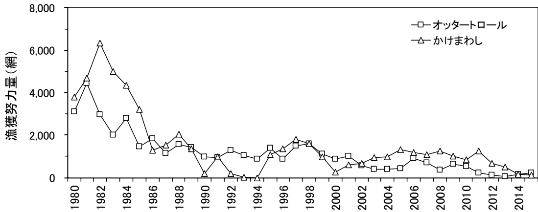
図4. イカナゴ類宗谷海峡に対する沖底の漁獲努力量 (有漁網数)
