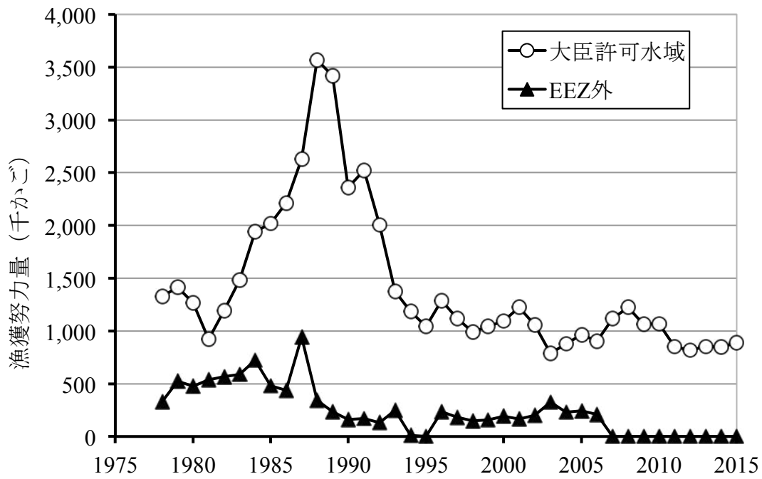
図5. 大臣許可水域及びEEZ外における漁獲努力量（かご数）の経年変化
