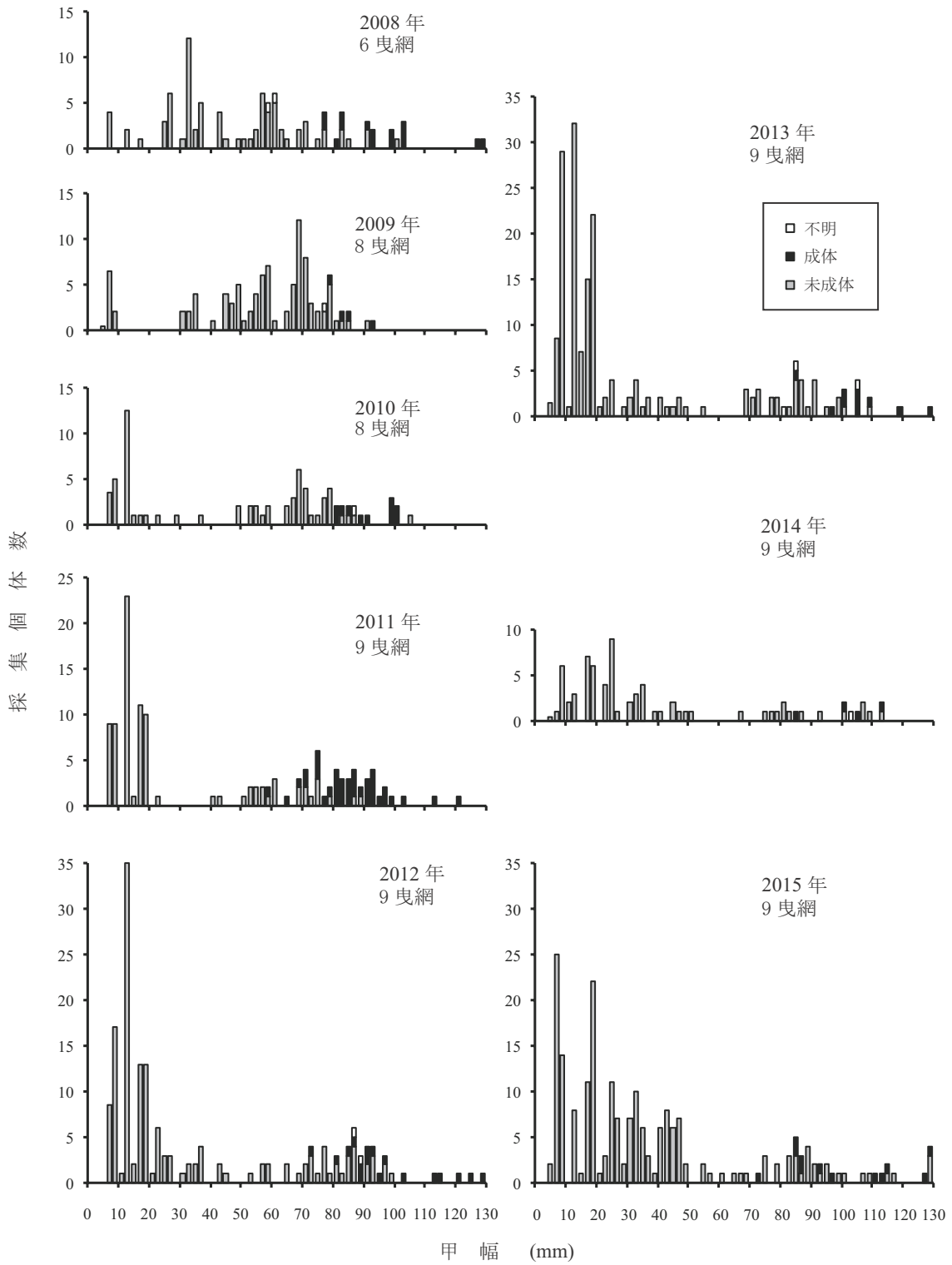
図 10. 2008～2015 年 8 月に富山湾内で、桁網により採集されたベニズワイガニ雄の甲幅組成
