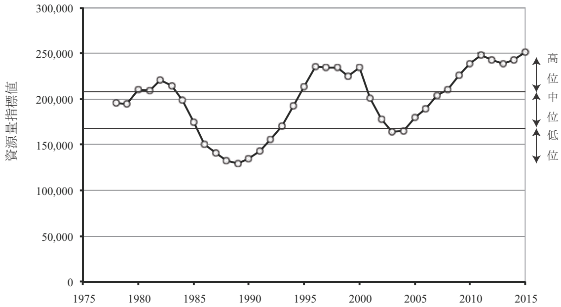
図 7 知事許可水域における資源量指標値の経年変化 資源量指標値の最高値と最低値の間を三等分して、上から高位、中位、低位とし、それぞれの境界を示した。高位／中位、中位／低位の境界値はそれぞれ 208,692 と 169,037 である。
