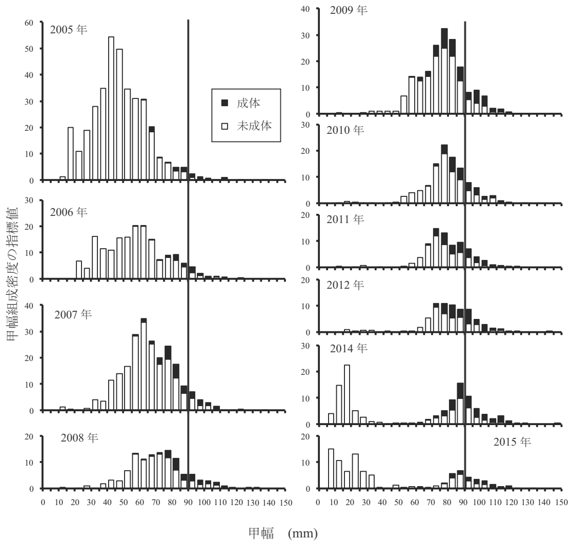
図 9. 2005～2015 年（2013 年は未実施）夏季に隠岐島西方海域で採集されたベニズワイガニ雄の甲幅組成密度の指標値（各調査定点での 1,000m 2 曳あたり密度組成の累計として計算）
