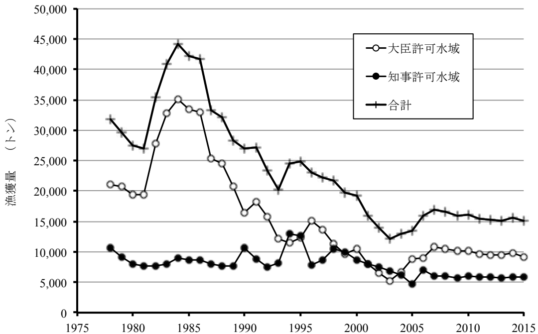
図 4. ベニズワイガニ日本海系群の許可水域別漁獲量
