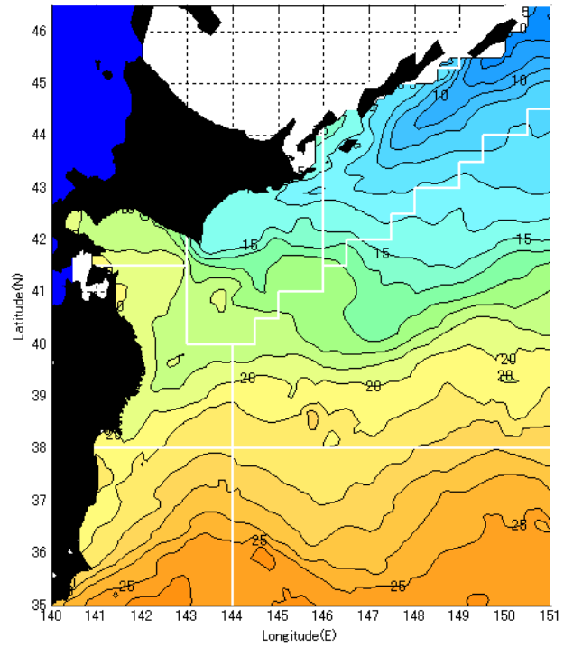
10月上旬予測水温分布図
