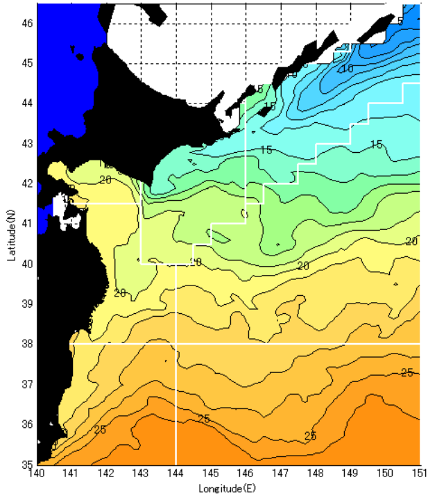
9月下旬予測水温分布図
