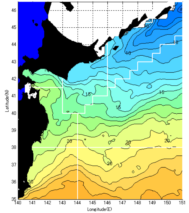
10月下旬予測水温分布図
