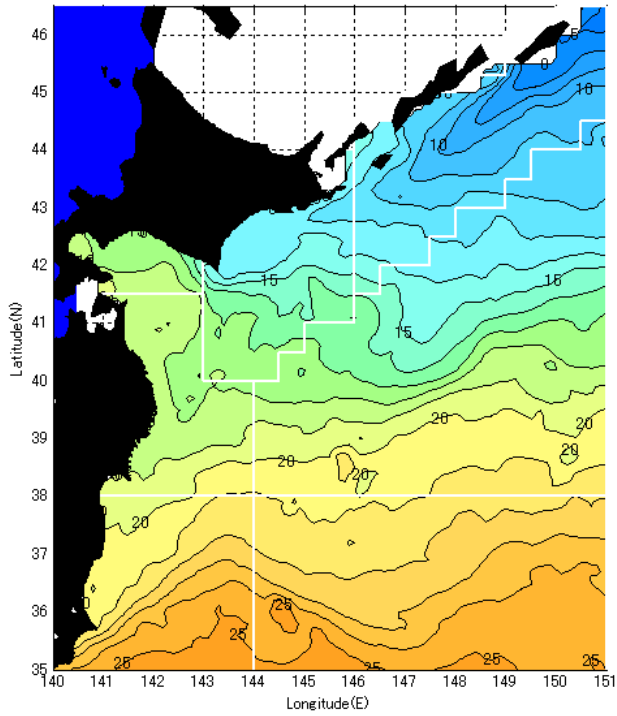
10月中旬予測水温分布図
