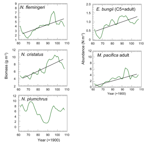
図 2. 春季 (4-5 月) の親潮域における大型カイアシ類 5 種の現存量の経年変動。緑線は 5 年の移動平均を示す。
