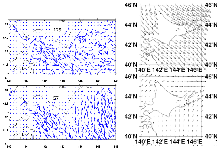
図 1. QuickSCAT Level2B による 2 月の平均風速（上：2006 年、下：2000 年；図中の数字は FEZI を示し 1999～2009 年でそれぞれ最大と最小となった（左）。2003 年の 3 月（上）と 4 月（下）の平均風向・風速（右）。2003 年は 1 月～3 月まで北西風が卓越し、4 月は南南西の風になった。2004 年は示さないが、4 月まで西風成分が卓越した。
