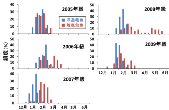
図 1. 浮遊稚魚 (青) と着底幼魚 (赤) のふ化日組成。
