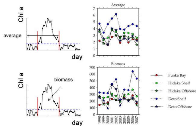
図3 海域別の春季ブルーム評価のための新しい指標
