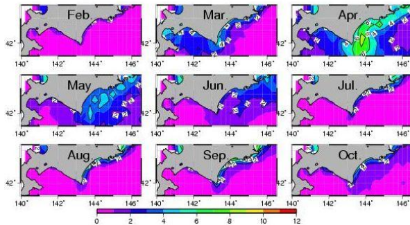
図1 衛星データから求められた、海面クロロフィル濃度の月別平均場
