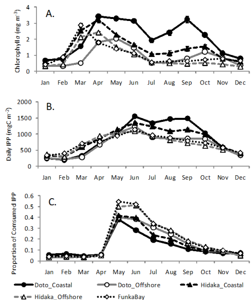
図4 各海域におけるクロロフィル a 濃度 (A)、日基礎生産量(B)、および日基礎生産量に対する動物プランクトンによる摂餌・分解量の割合 (C) の季節変化
