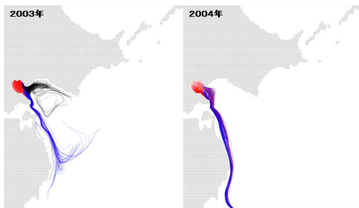
図 2. 粒子のうち噴火湾内に入った粒子の 4 月 1 日から 30 日後までの軌跡を示す。黒は日高湾陸棚、青は噴火湾口部、赤は噴火湾内に置いた粒子。2003 年では粒子は日高湾沿岸にそって室蘭側から噴火湾に流入する。2004 年では噴火湾外から湾内へ流入する粒子はない。
