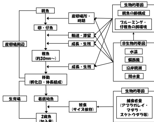
図1. 加入量変動に関するコンセプトモデル
