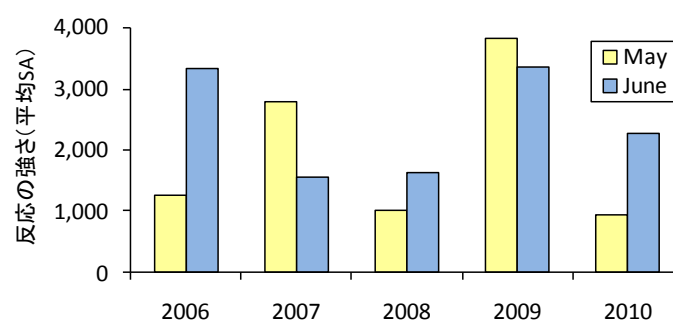
図2. 噴火湾内における海域平均の魚探反応 ( S_A ) の強さ（栽培水試）
