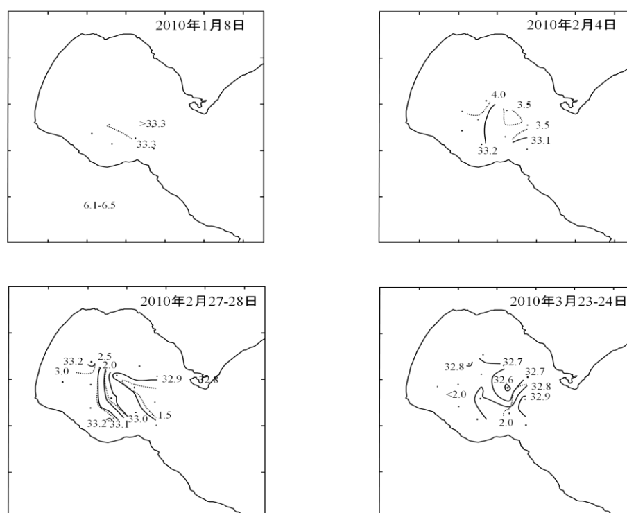
図1. 2010年冬季の噴火湾における海洋環境（北大調査）
