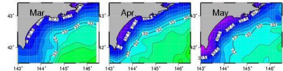
図2 10m深における塩分の月別平均場
