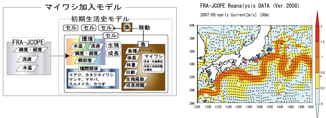
図 1. マイワシ加入モデルの概要 今回のシミュレーションでは、餌密度、種間関係にある各魚種の資源量は定数（平均値等）を用いた。
