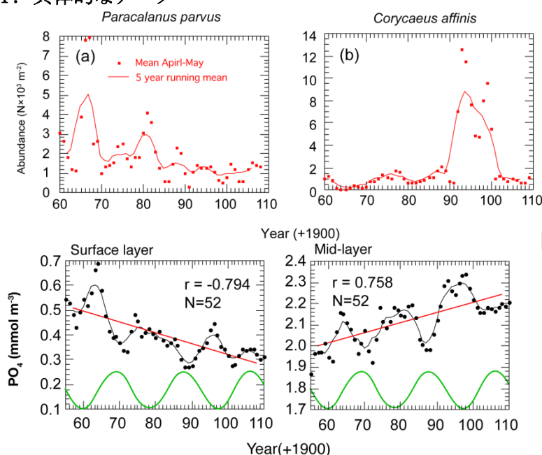
図 1 混合域における Paracalanus parvus (a) と Corycaeus affinis (b) 現存量の春～夏の年平均值 (4-5 月) の経年変動。
