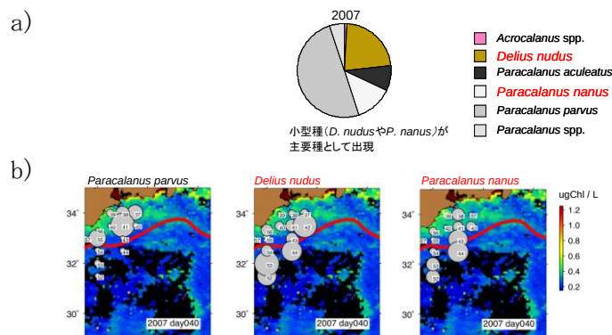
図1. 2007年2月の黒潮南方域におけるカイアシ類組成 a) と主要3種の水平分布 b)。
