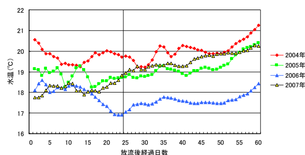
図 2. 2004~2007 年における、4 月に孵化した卵の経験水温の比較。
