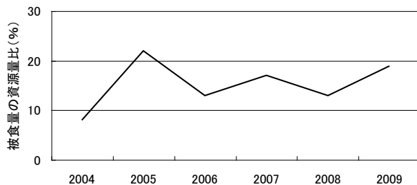
図 3. カタクチイワシ 0 歳魚の被食量の資源量に 対する比率
