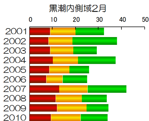
図2 黒潮内側域における2月のかいあし類現存量( \text{mm}^3/\text{m}^3 )の経年変化。
