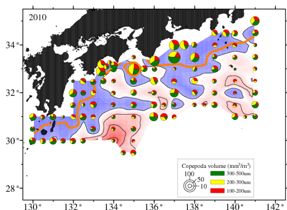
図1 2010年2月かいあし類体積と混合層深度の分布(混合層は \Delta T=0.2^{\circ}\text{C} で定義した)。橙色線は水深200mにおける 16^{\circ}\text{C} 等温線を示す。
