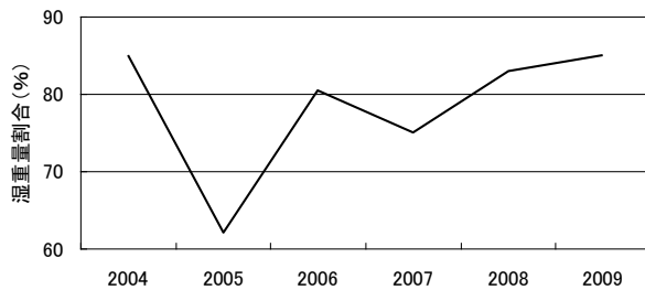
図 1. 胃内容物全湿重量のうち カタクチイワシが占める割合
