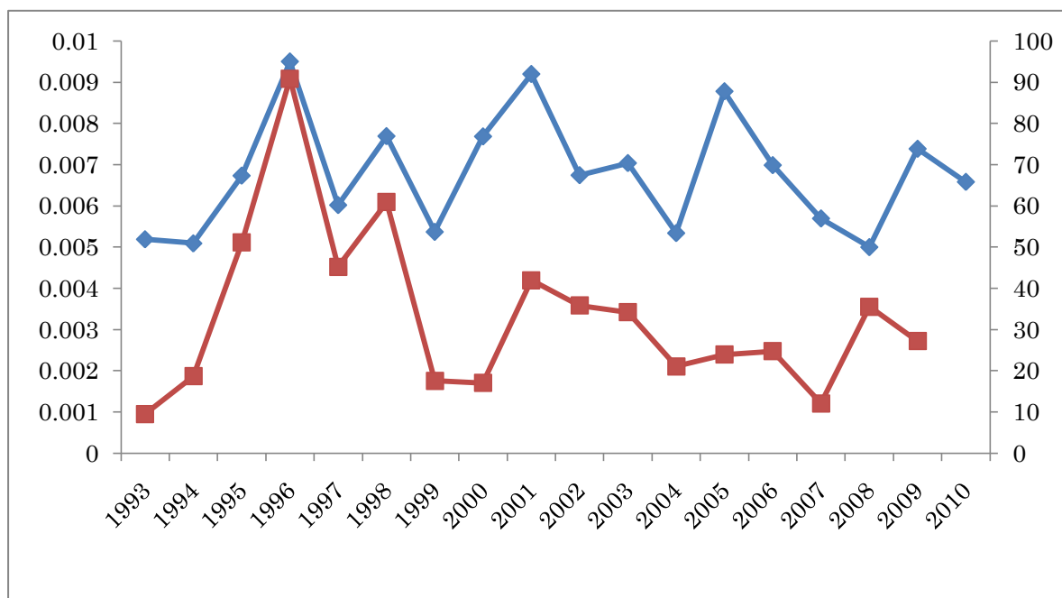
図 3. シミュレーションによるマイワシの生残率（青線）と実測値（赤線）
