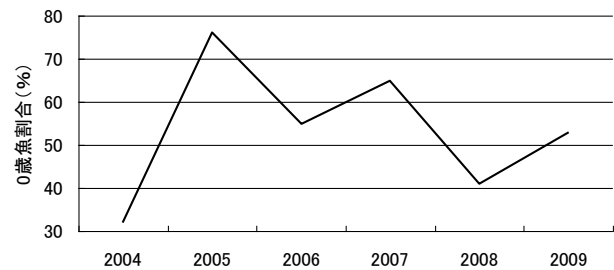
図 2. 胃内容物としてのカタクチイワシのうち 0歳魚が占める割合 (湿重量)
