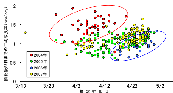
図 1. マサバの 2004~2007 年級群の孵化日別に対する 25 日齢までの成長速度の分布。
