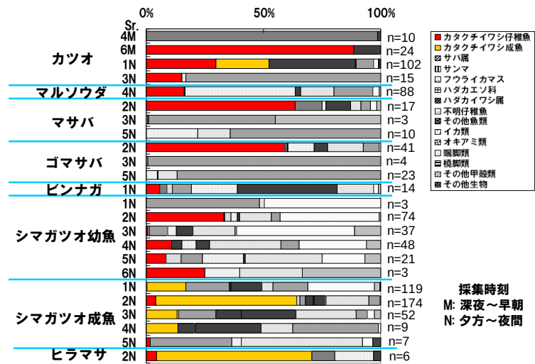
図 1: 2005-2006 年 5-6 月に黒潮親潮移行域で流し網(開運丸)により採集された主要な魚食性魚類の胃内容物の重量比。
