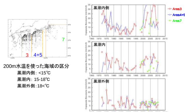
図2. 卓上型ビデオプランクトンレコーダー(B-VPR)を用いた黒潮および黒潮属流域のカイアシ類密度の経年変動。
