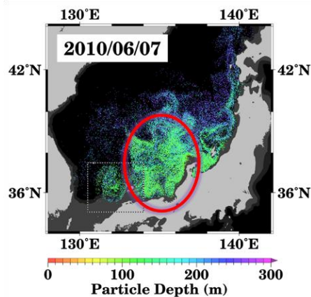
図 4 JADE データを用いたズワイガニ属幼生分布の再現結果。若狭湾沖（大和海盆）に大量の幼生が滞留する状況を再現。
