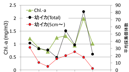
図 3. 2003 年～2010 年の衛星画像（MODIS）による Chl. -a の分布（左図）と、沖合域（北緯 37-39 度、東経 132-137 度）における平均 Chl. -a 密度と幼スルメイカの採集個体数の経年変化
