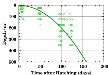
図 3 分布調査データから推定したズワイ幼生期の沈降曲線（孵出海域を浜田沖、孵出時期を 2～3 月と仮定）。
