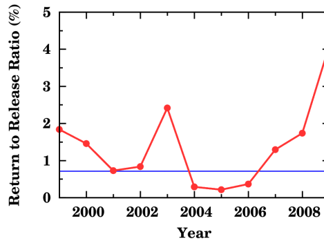
図5 JADE 計算により推定された幼生帰還率の年々変動（99～09年）。赤：各年の帰還率、青：11年平均流速場による帰還率。気候値的な流れでは高い帰還率は望めないが、年ごとに化する流況に応じて帰還率が非常に高くなる年が生じる。
