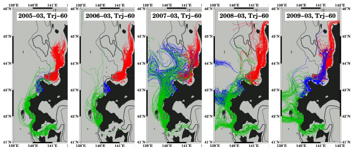
図 2. 2005～2009 年のスケトウダラ 3 月ふ化群卵仔魚の JADE による輸送シミュレーション。産卵場の設定は、緑：檜山、青：岩内、赤：石狩。
