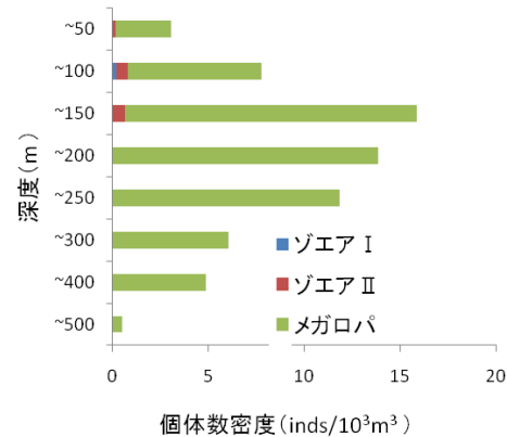
図 2 ズワイガニ属幼生の鉛直分布（H22 年 6 月）。
