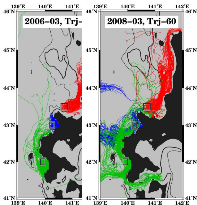
図 3. 2006 年および 2008 年の 3 月ふ化群を想定した卵仔魚の輸送シミュレーション結果. 各色はスタートの産卵場の違いを示す (緑: 檜山、青: 岩内、赤: 石狩).
