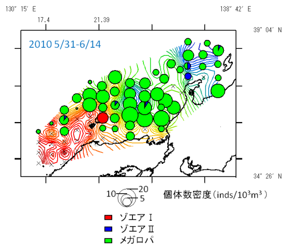
図 1 ズワイガニ属幼生の水平分布（H22 年 6 月）。
