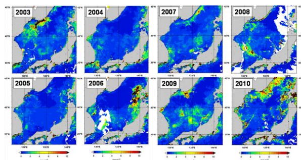
図 3. 2003 年～2010 年の衛星画像（MODIS）による Chl. -a の分布（左図）と、沖合域（北緯 37-39 度、東経 132-137 度）における平均 Chl. -a 密度と幼スルメイカの採集個体数の経年変化
