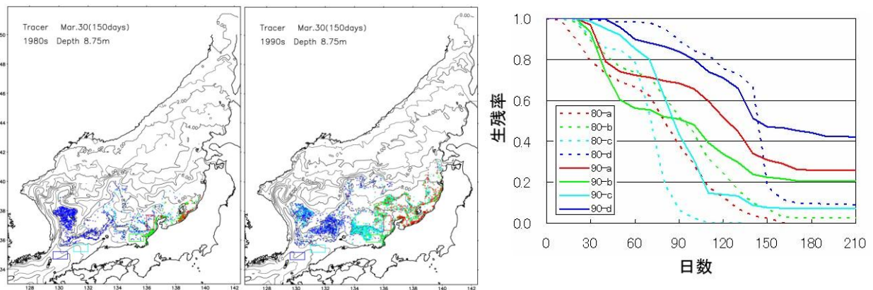
図 1. スルメイカの中長期海洋モデルを用いたシミュレーションによる 1980 年代と 1990 年代の生残率の変化シミュレーション結果(平成 20 年度成果報告書より)
