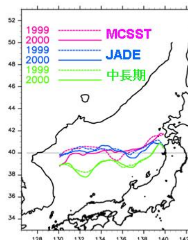
図2. 海面水温勾配から見積もった極前線の年平均位置の推移.
