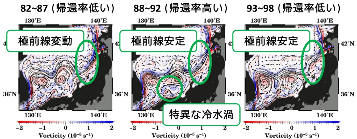
図 3. 中長期海洋モデルによるズワイガニ幼生の帰還率（設定した産卵場＝山陰沿岸付近の大陸棚斜面へ輸送される割合）の変化と対馬暖流の流動の関係。
