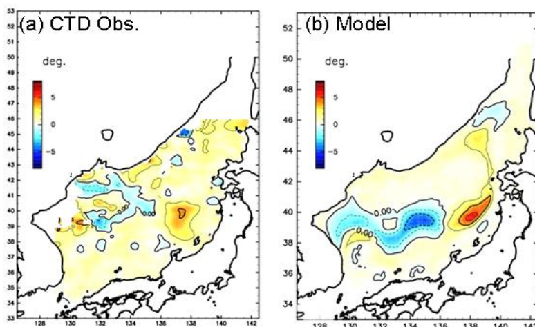
図1. (a) CTD 観測で得られた 50m 深水温を使用して見積もった 1990 年代(1993-1998)から 1980 年代(1982-1987)を差し引いた水温偏差. (b) (a)と同様. ただし, 中長期モデルで再現された 42.5m 深水温を使用.
