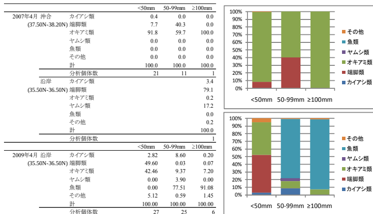
図 1. 新規加入量調査（2007 年および 2009 年 4 月）で採集した幼スルメイカの消化管内容物（重量組成%）。
