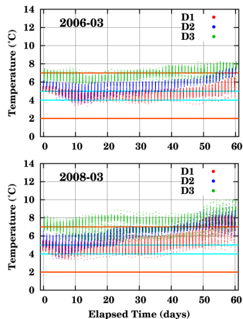
図 4. 輸送シミュレーションで得られた卵仔魚の経験水温分布. 各色はスタートの産卵場の違いを示す (緑: 檜山、青: 岩内、赤: 石狩). また、赤線は生存の適水温帯 (2~7°C)、青線は最適水温帯 (4~5°C) をそれぞれ示す.
