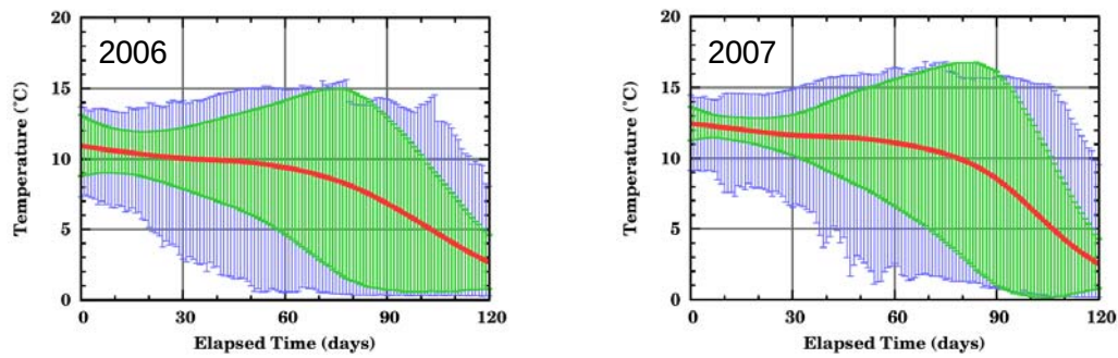
図1: 改良した生物輸送モデルを用いたズワイガニ幼生の輸送・着底シミュレーション（試行）により得られた経験水温の例。追跡開始からの日数で整理して示す。赤線は着底していない粒子すべての経験水温を平均したもの、緑線は平均値のまわりに標準偏差を、青線は同じく最大値・最小値の範囲を示す。左は2006年（寒冬）の、右は2007年（暖冬）の例。
