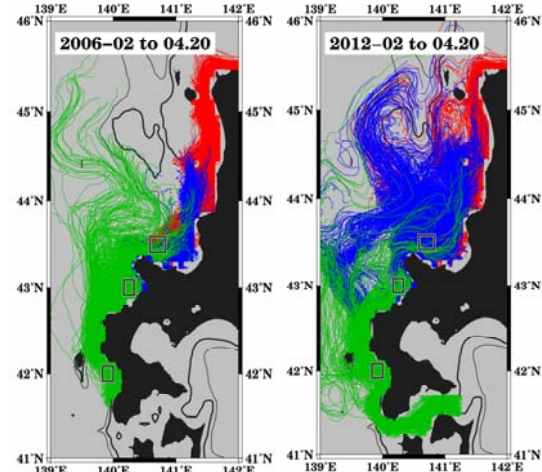
図2. 改良版JADEで推定した2006年および2012年の輸送特性.
