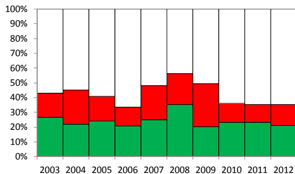
図1 2003年～2012年の4月20日の日本海の表面水温における各水温域の面積比率の変化 (左図)
