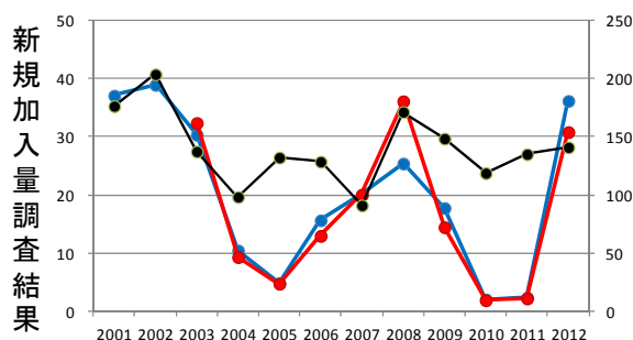
図2 4月のスルメイカ新規加入量調査結果とスルメイカ秋季発生系群の推定資源量
