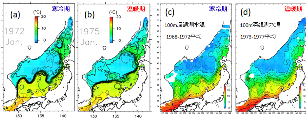
図 1. (a) 中長期モデルで計算された 1972 年 1 月の月平均水温場。(b) (a) と同じだが、1975 年 1 月のもの。(c) 日本海各層水温データセットから見積もった 100m 深水温の 1968～1972 年における平均場。(d) (c) と同じだが、1973～1977 年平均のもの。
