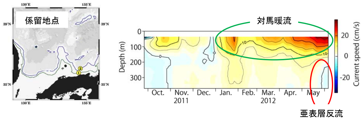
図2: 係留系設置地点と観測結果（第1報）。浜坂沖保護礁内には流速計1基(ADCP)を用いた楕円型ブイシステム(左図)を、但馬沖には流速計2基(ADCPとAANDERAA)を用いた系(左図2)を設置している。但馬沖ADCPが計測した東西方向流速の時系列(右図)をみると、対馬暖流の下方に形成初期の亜表層反流と思われる現象が捉えられていた（2012年5月下旬）。
