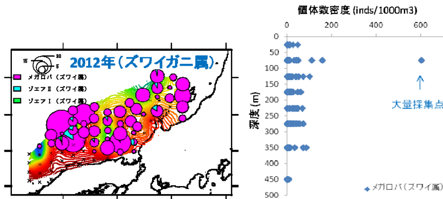
図 2 2012 年 6 月のズワイガニ属幼生の水平および鉛直分布
