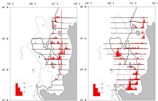
図1. 5月のすけとうだら音響調査で計測された0歳魚の分布密度(尾/m 2 ).
