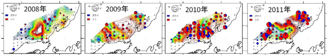
図 1 毎年のズワイガニ属メガロパ分布（2008～2011 年の 6 月）
