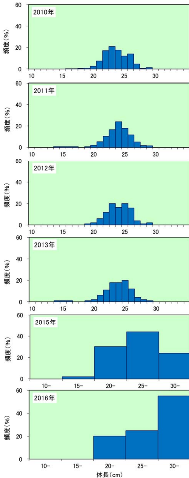
図5. オホーツク海におけるキチジ漁獲物体長組成 (2010～2013年：延縄漁業の漁獲物、網走水産試験場 2014、 2015～2016年：延縄漁業・刺し網漁業の漁獲物、体長階級幅は5cm)
