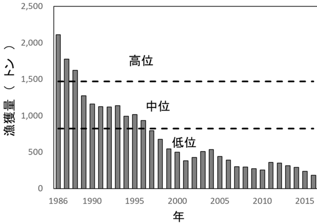
図 6. キチジオホーツク海系群の漁獲量の推移と資源水準の判断 2016 年は暫定値 (漁獲量の最高値～最低値を 3 等分した、図中の点線は資源水準の境界を示す)
