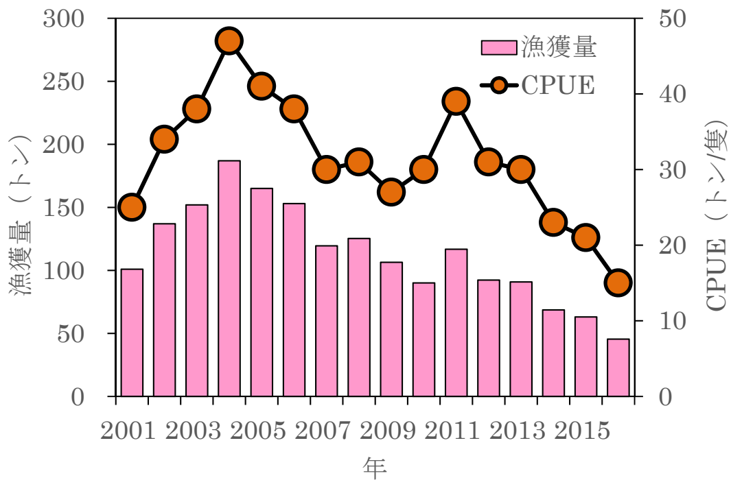
図4. オホーツク海における延縄漁業の漁獲量とCPUE（資源量指標値）の推移（網走水産試験場 2018）
