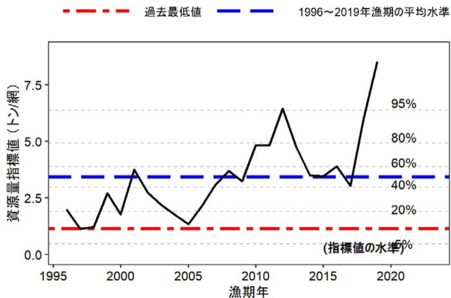
補足図 3-1. 資源量指標値の推移と水準
