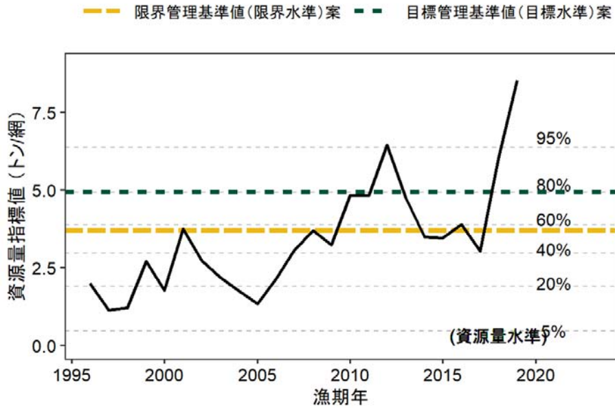
補足図 4-1. 漁獲管理規則案
