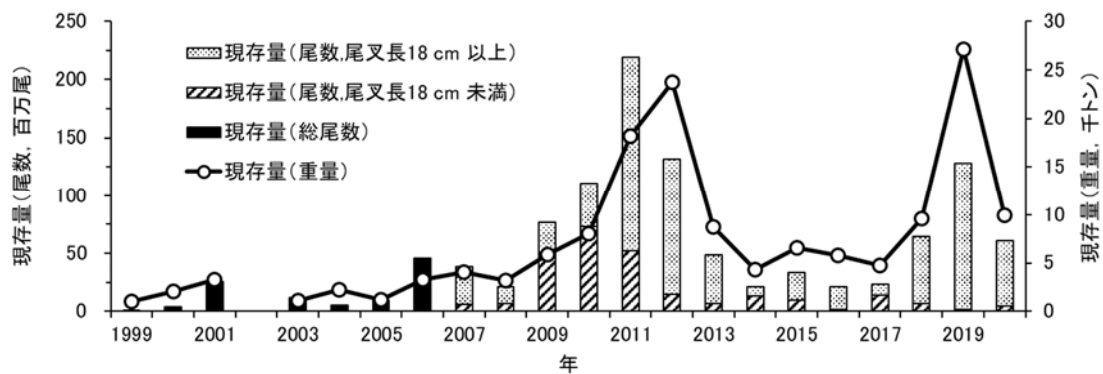
図 4-4. オホーツク海底魚資源調査から推定されたスケトウダラの現存量 2002 年は調査未実施のためデータ無し
