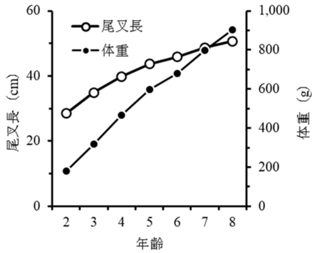
図 2-3. 沖底漁獲物の平均尾叉長と平均体重 (2009~2019 年の 4~7 月)
