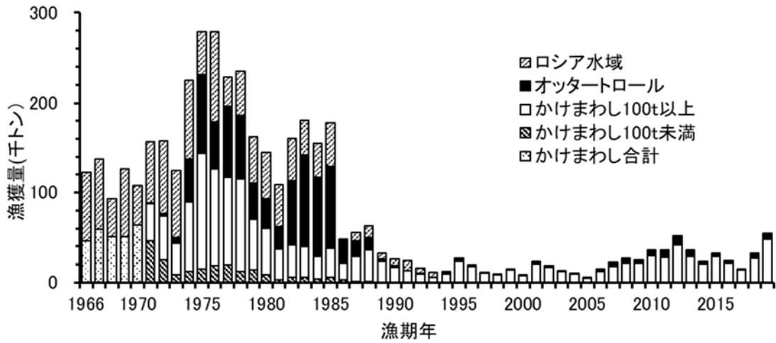
図 3-1. 沖合底びき網漁業による漁獲量の推移
