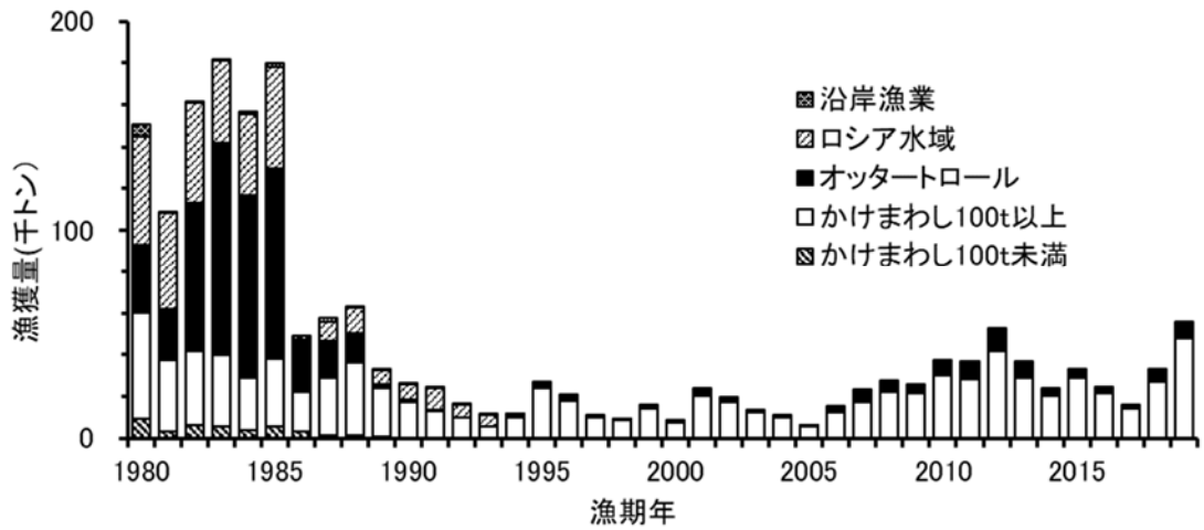
図 3-2. 日本水域における漁獲量の推移
