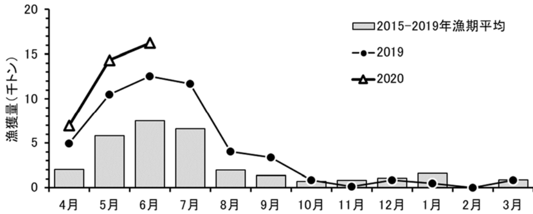
図 3-3. 沖底月別漁獲量、2019 年漁期値は暫定値、2020 年漁期値は速報値である。
