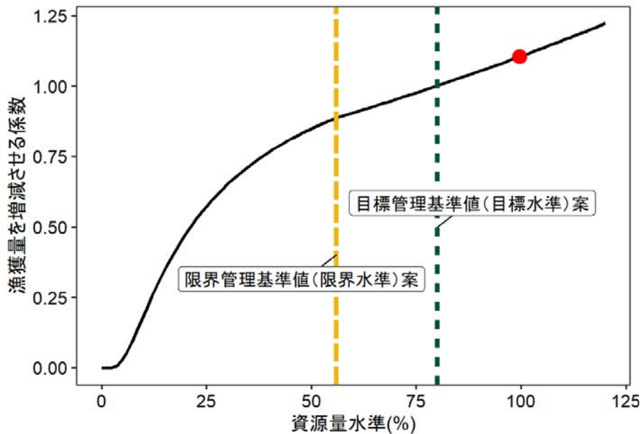
補足図 4-2. 資源量指標値の水準
