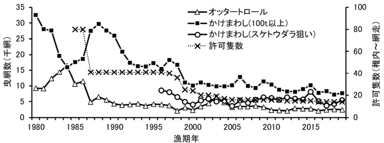
図 3-5. 沖合底びき網漁業の努力量（曳網数）の動向
