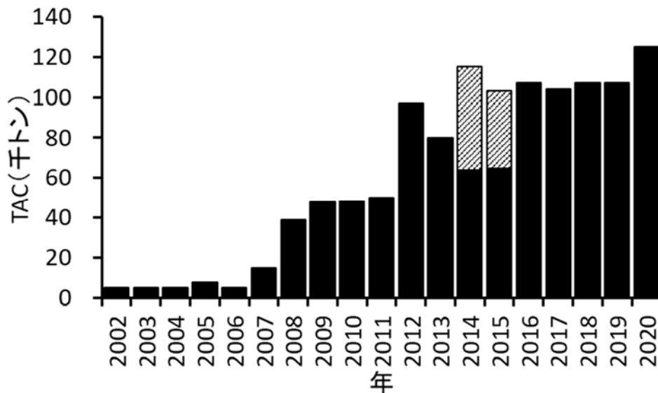
図 3-4. ロシア連邦が設定している漁業海区名「東サハリン」における TAC 斜線は期中改定による増加分を示す。
