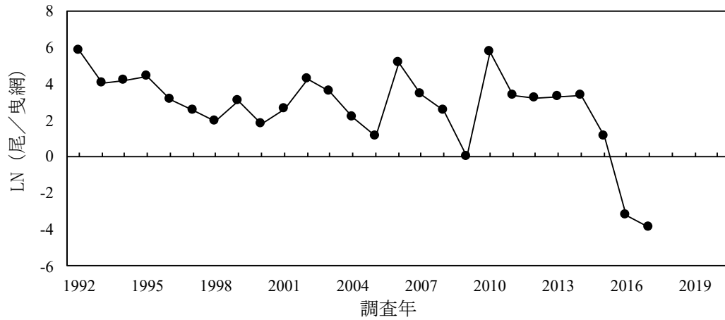
図 4. 資源量指標値の推移：愛知、三重両県が行った新規加入量調査結果（2月上旬伊勢湾内におけるイカナゴ仔稚魚の平均分布密度の対数値）の推移 2018～2020年は仔稚魚が採集されず資源量指標値の計算は不可能。
