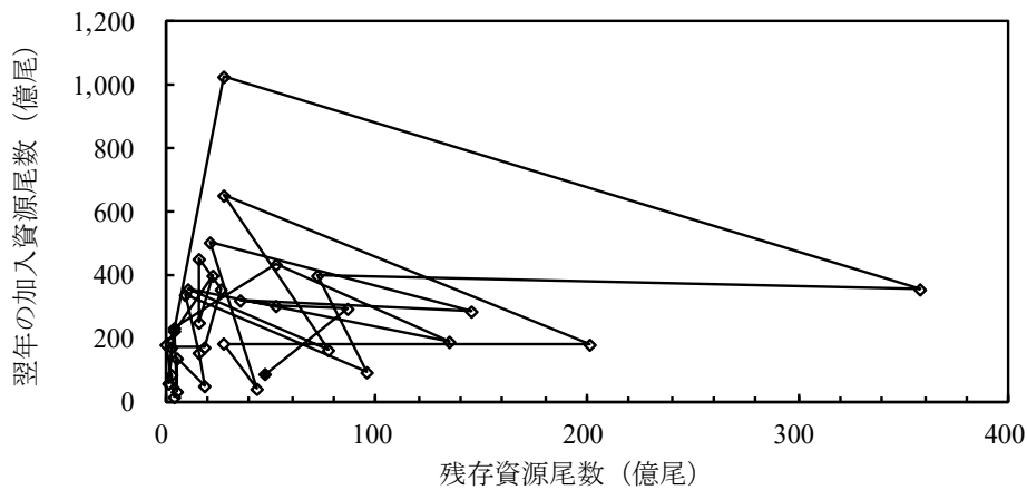
図 8. 伊勢・三河湾におけるイカナゴの再生産関係（残存資源尾数に対する翌年の加入資源尾数の関係：1979～2014年（36年間）） ◇：1979～2013年（35年間）、◆：2014年
