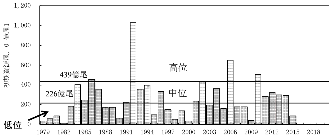
図 5. 伊勢・三河湾におけるイカナゴの推定加入資源尾数の経年変化（1979～2015年） 2016～2020年はデータなし。
