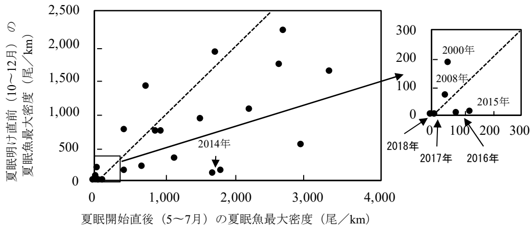
図 10. 夏眠中の減耗の検討 (夏眠開始直後の夏眠魚最大密度と夏眠明け直前の夏眠魚最大密度の関係 : 1979~2018 年 (1995、1998、1999、2005、2006 年を除く 22 年間)) 破線は生残率を 1 とした場合の直線。2014~2017 年の夏眠魚の生残率はそれぞれ 0.070、0.053、0.035、0.033 で、それ以前と比べて低く、年を追うごとに減少。
