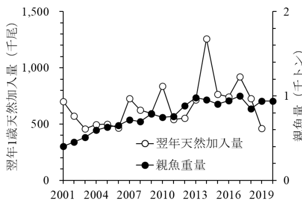
図 11. 親魚量と天然魚加入量
