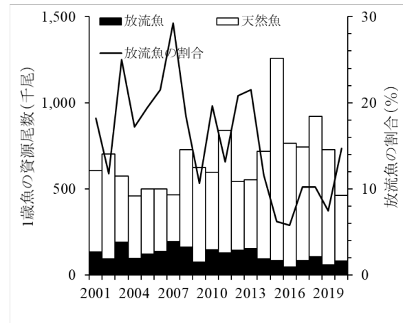
図 10. 天然と放流魚別の 1 歳資源尾数
