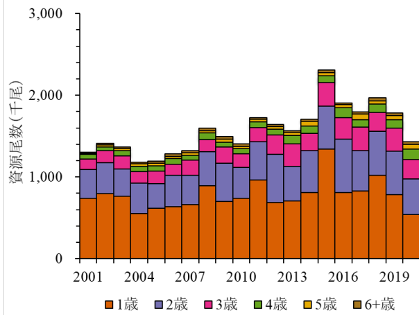
図 7. 年齢別資源尾数 (1 歳以上)
