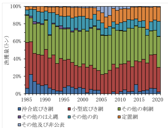
図2. 漁業種類別漁獲割合(太平洋中区)
