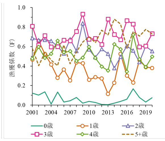
図6. 年齢別漁獲係数
