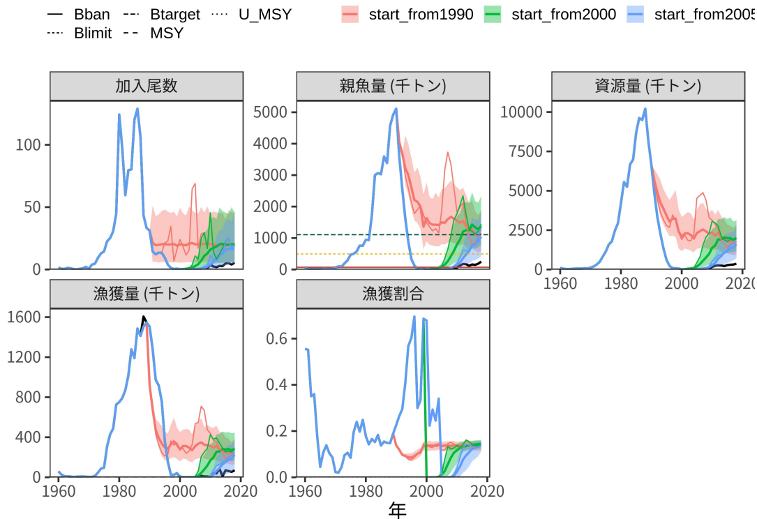
図 4 マイワシ対馬暖流系群で過去にさかのぼった場合のシミュレーションを実施した例．1990 年 (start_from1990)，2000 年 (start_from2000)，2005 年 (start_from2005) から，通常レジームの管理基準値を使って管理を開始した 3 通りの結果の比較．細い実線は過去に見られた残差をそのまま用いたもの（シナリオ 1），塗りの範囲は過去の残差を確率分布からランダムに発生させたシミュレーションの 90 %信頼区間，太い実線はシミュレーションの結果の平均値．親魚量が禁漁水準を割っている 2000 年，2005 年では，管理開始当初の漁獲量はゼロになったのち，親魚量が回復したのちに漁獲が再開している．
