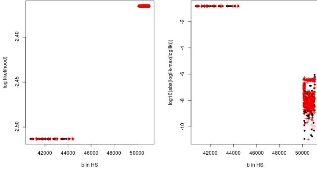
図1 HSに解の不安定性がある場合の例。最尤推定値と思われる値周辺にランダムに初期値を設定してパラメータ推定したときに推定されたHSのパラメータ b (x軸) とそのときの対数尤度 (y軸, 左), 試行した中で得られた最大の対数尤度と個々の推定で得られた対数尤度との差の絶対値の対数 ( \log_{10} ) をとったもの (y軸, 右). 右図の y 軸は差の \log_{10} をとったものなので, -3 は最大対数尤度との差が 0.001 であることを示す. 図の黒点と赤点は, 異なる乱数のシードからランダムに初期値を変えてそれぞれ 500 回繰り返し計算を行った場合の結果. 左図で示すように尤度が高い b=5 万トン付近では尤度の値がほとんど変わらないパラメータの範囲が存在する. 右図で, 尤度の差の対数をとると 10^{-6} 以下の差で尤度の違いが見られるが, 尤度の違いの傾向はスムーズではなく, 高い初期値依存性を示唆する.
