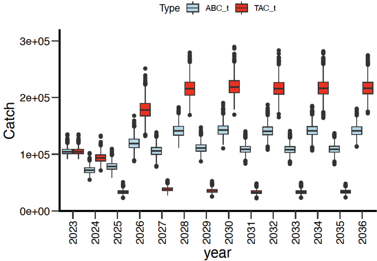
図5 ABCの繰入・繰越を行う場合の結果の図
