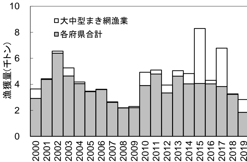
図7. 日本における漁獲量
