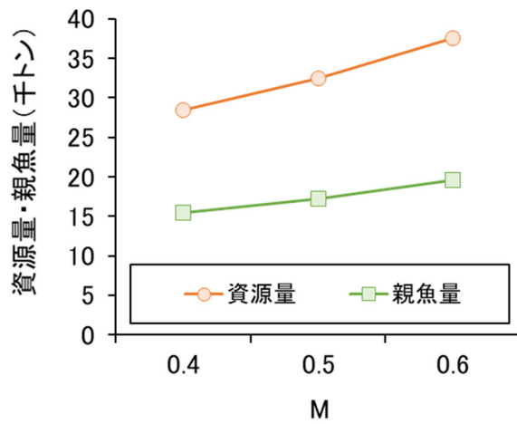
図 4-4. 自然死亡係数 M を変化した場合の資源量と親魚量
