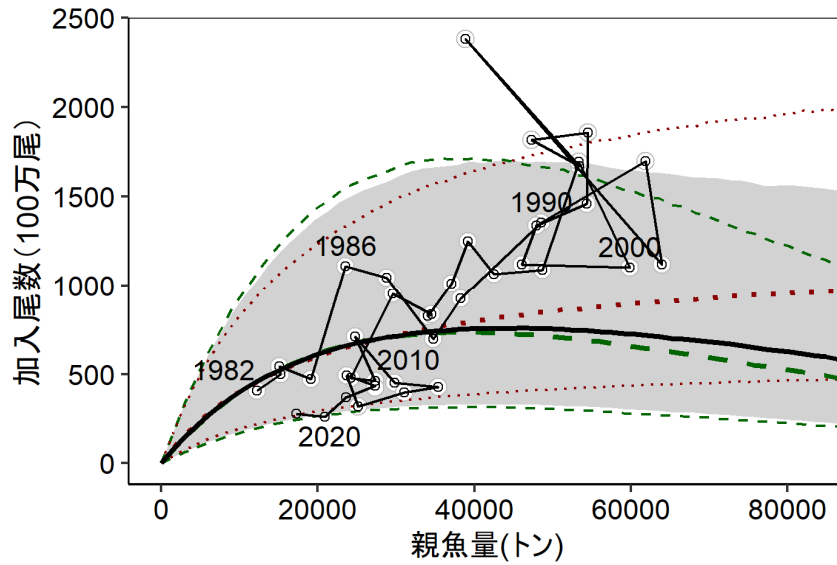
図 4-9. 親魚量と加入量との関係（白抜丸印および実線: 1982～2020 年）。太線は本系群で適用した再生産関係式（黒）、リッカー型（緑）およびベバートン・ホルト型（赤）の予測値であり、灰色領域と細線はそれぞれ仮定されている再生産関係において観察データの 90%が含まれると推定される範囲である。各再生産関係式のパラメータは令和 2 年 3 月に開催された「管理基準値等に関する研究機関会議」（井須ほか 2020）に示された値に基づく。白丸印は再生産関係を求めるのに使用した令和元（2019）年度資源評価における親魚量と加入量との関係（1982～2017 年）。
