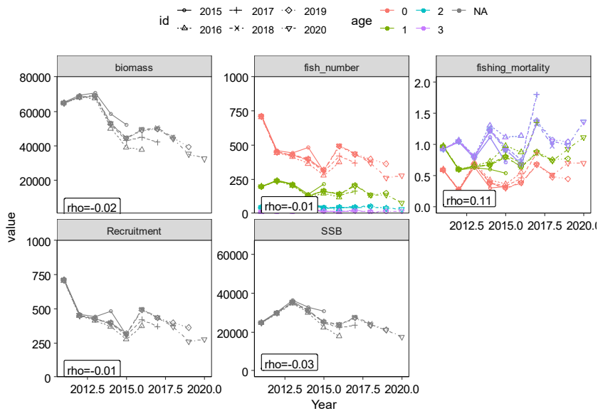
補足図 2-2. レトロスペクティブ解析の結果
