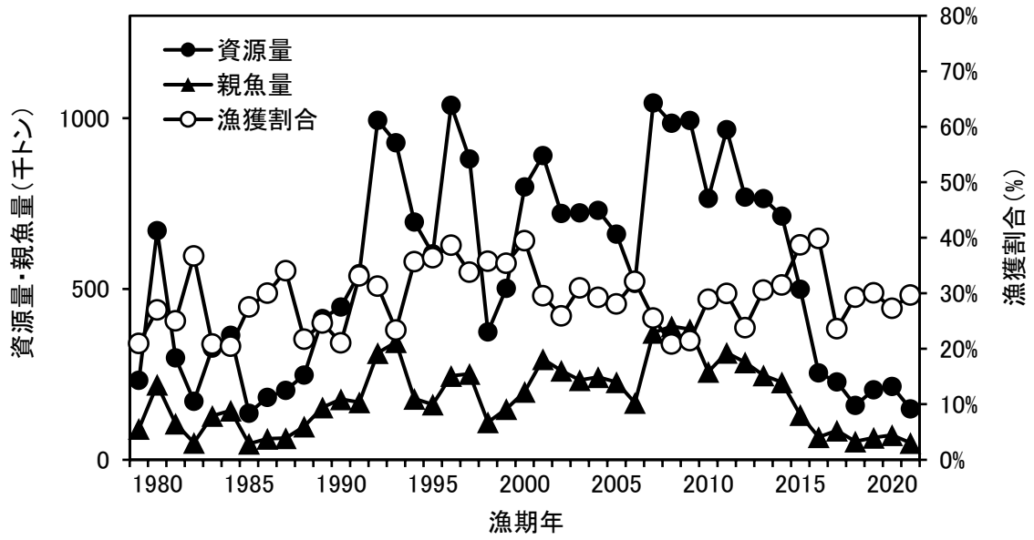
図 4-1. 資源量と親魚量と漁獲割合
