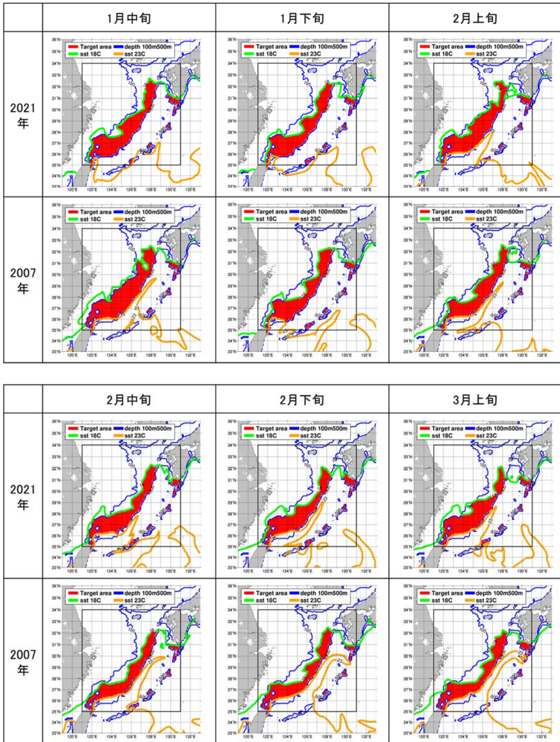
補足図 4-7. 2007年と2021年の1月中旬～3月上旬の東シナ海におけるスルメイカの再生産可能海域（赤色の海域） 再生産可能海域の定義は水深100～500mかつ表面水温18.0～23.0°Cの海域。
