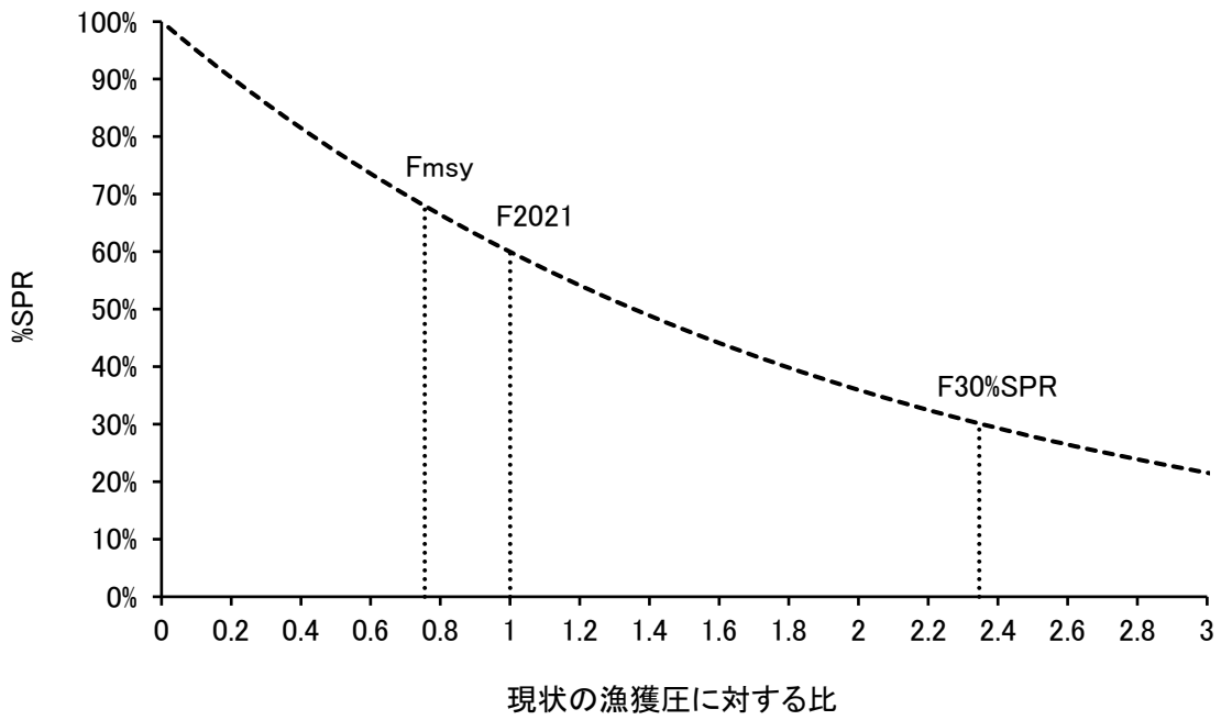
図 4-7. %SPR と現状の漁獲圧との関係
