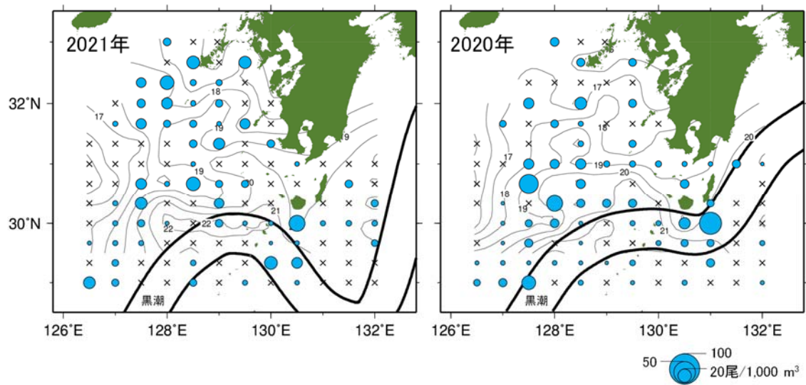
補足図 4-2. 2020、2021 年 2 月上旬～2 月下旬の九州南西海域で採集されたスルメイカ幼生の水平分布（尾/1,000 m 3 ）、海面水温（細実線）および黒潮流路（2 本の太実線） 黒潮流路は、海洋速報（ http://www.kaiho.mlit.go.jp/ ）を引用。×は採集されなかった点を示す。
