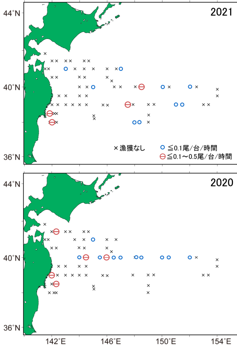
補足図 4-4. 2020、2021 年 6 月に実施された第 1 次漁場一斉調査における CPUE（釣り機 1 台 1 時間あたり漁獲尾数）の分布 ×は漁獲がなかった点を示す。
