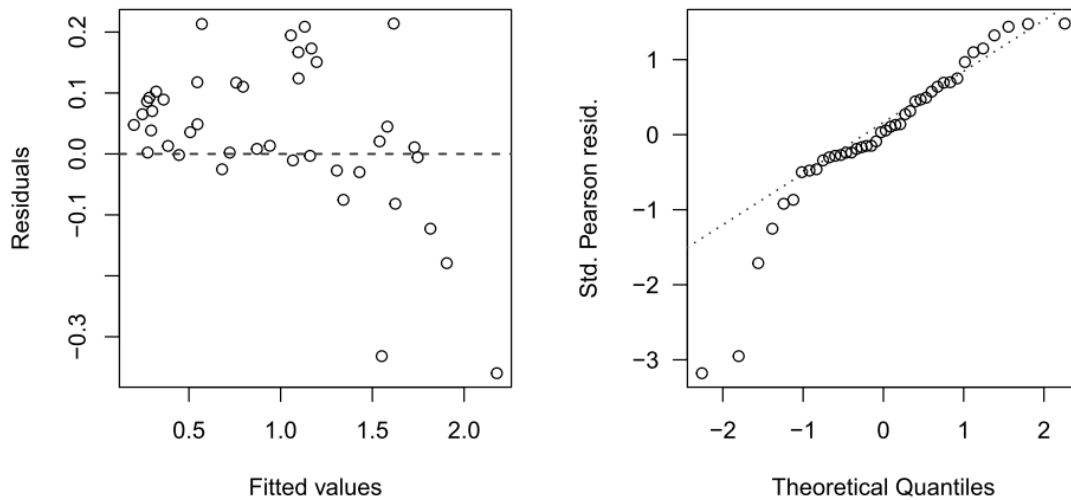
補足図 3-1. 2020 年度の資源量指標値予測モデル（加賀ほか 2021）の残差分布と QQ プロット
