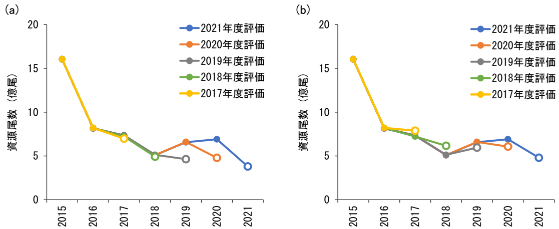
補足図 3-3. 資源量指標値の予測に関するレトロスペクティブ解析の結果
