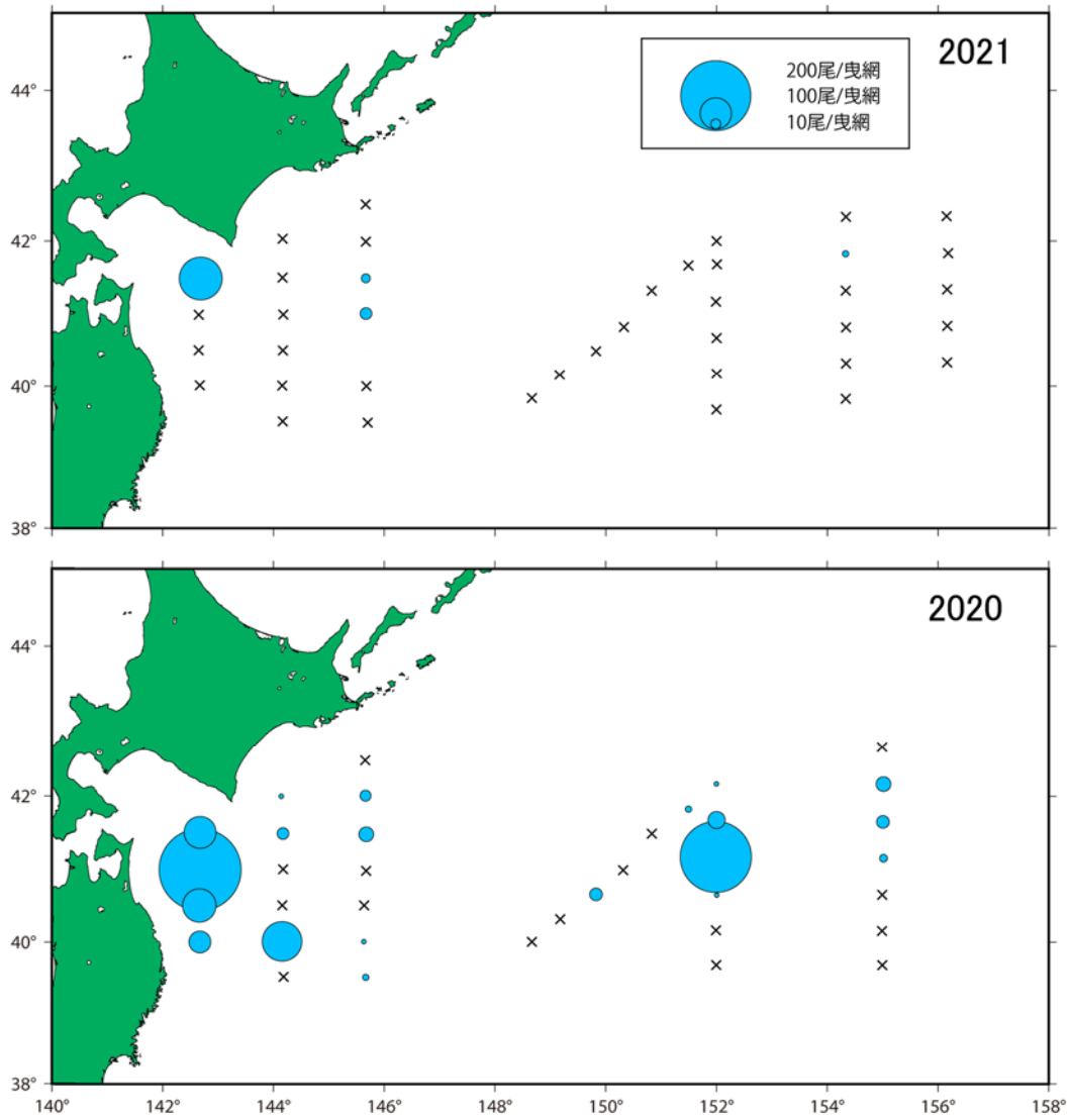
補足図 4-6. 2020 年、2021 年 7 月に実施された加入量把握調査で漁獲されたスルメイカの CPUE (尾/網)
