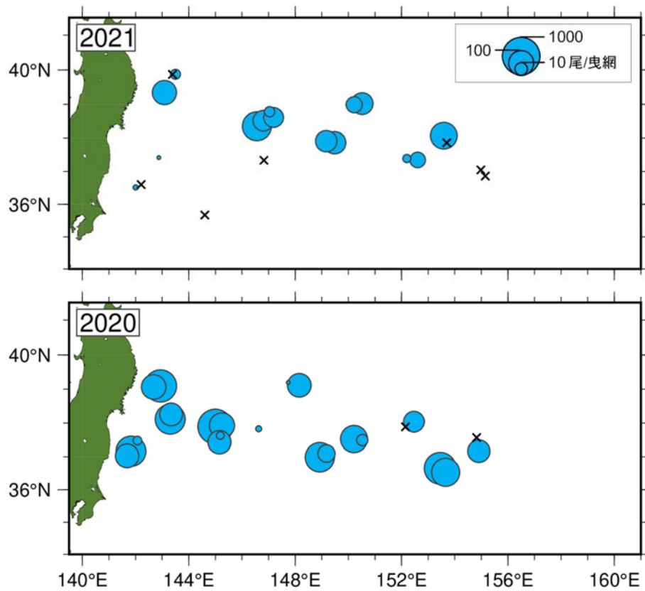
補足図4-5. 2020、2021年5～6月に実施された移行域幼稚魚調査で漁獲された幼体のCPUE (尾/網)
