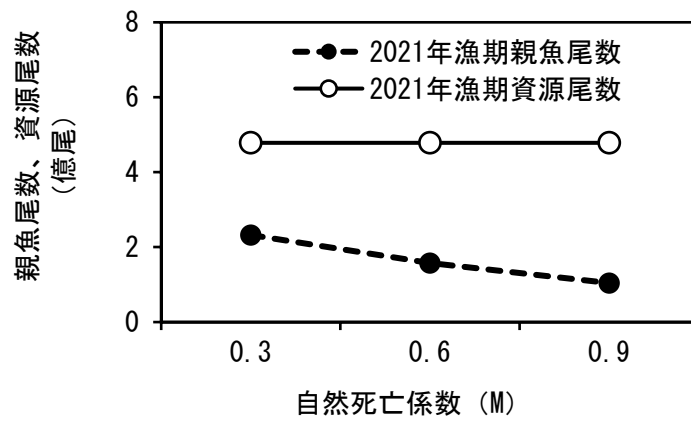
図 4-4. 自然死亡係数と親魚尾数、資源尾数の関係 (標準値 0.6)
