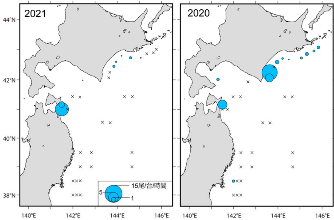
補足図 4-3. 2020、2021 年 8 月下旬～9 月中旬に実施された第 2 次漁場一斉調査および道東太平洋いか類南下期資源調査における CPUE (釣り機 1 台 1 時間あたり漁獲尾数) の分布 ×は漁獲がなかった点を示す。
