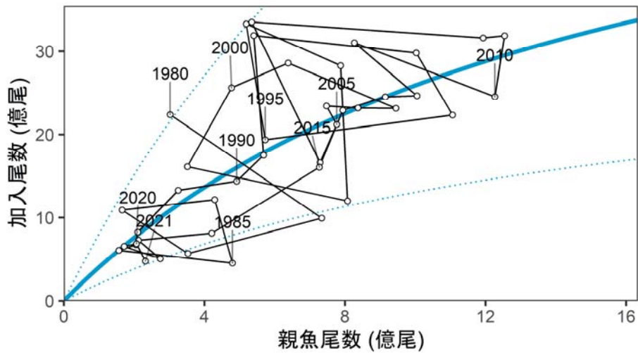
図 4-8. 親魚量と加入量の関係（再生産関係）
