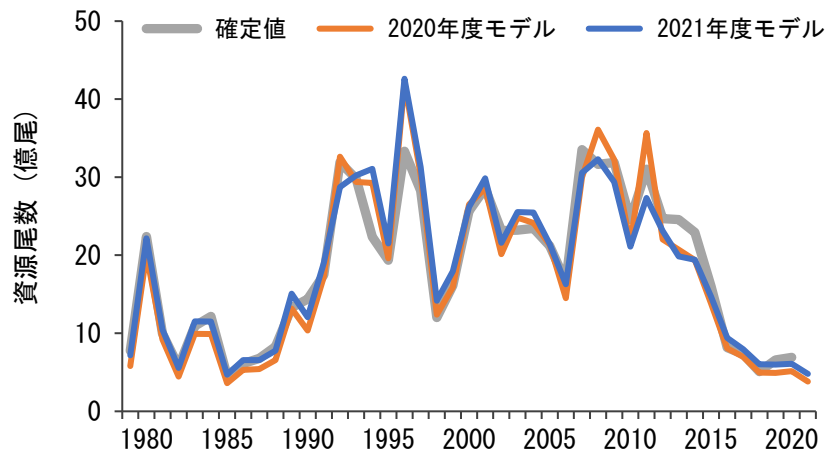
補足図 3-4. 資源量指標値予測モデルの交差検証 (Leave one out 法) における予測結果
