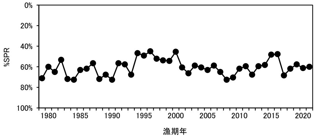
図 4-6. %SPR の経年変化
