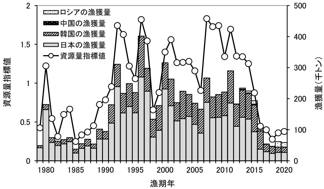
図 3-2. 国別漁獲量と資源量指標値の推移
