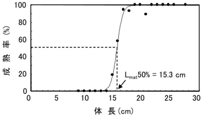
図3. 体長と成熟割合の関係
