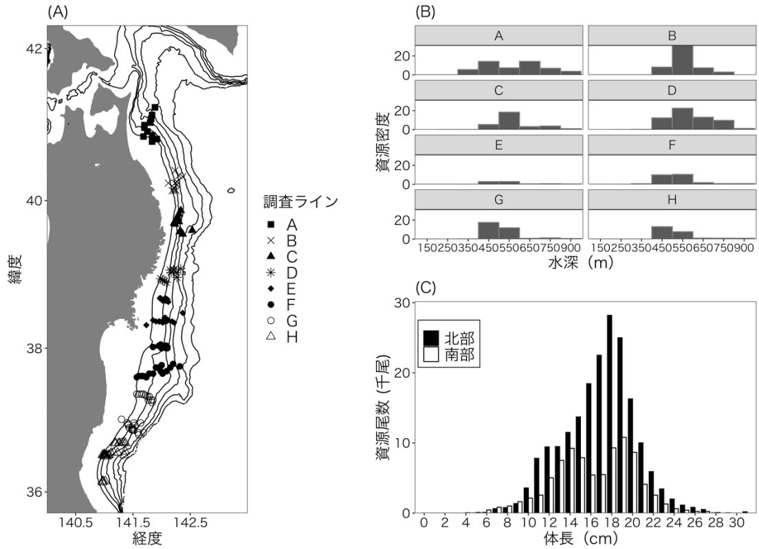
補足図 3-1. 2020 年 10～11 月の資源量調査の概要 (A) 曳網地点、(B) 各調査ラインにおける水深帯別の分布密度 (千尾/km 2 )、(C) 東北北部海域 (北緯 38°50'以北; A から D)・南部海域 (北緯 38°50'以南; E から H) における体長組成 ここでは、採集効率を 1 と仮定した場合の結果を示している。
