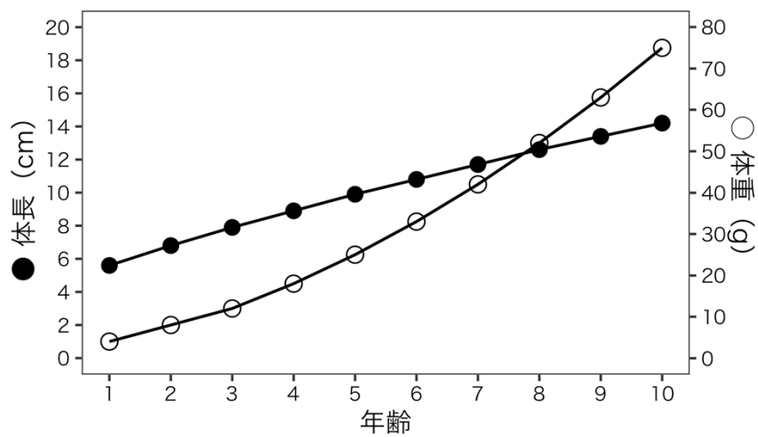
図2. 年齢と成長（体長・体重）の関係
