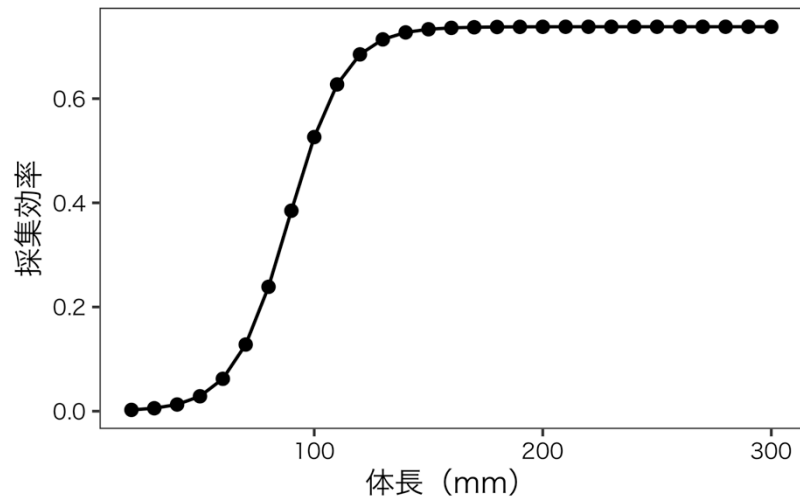
図7. 体長と採集効率の関係
