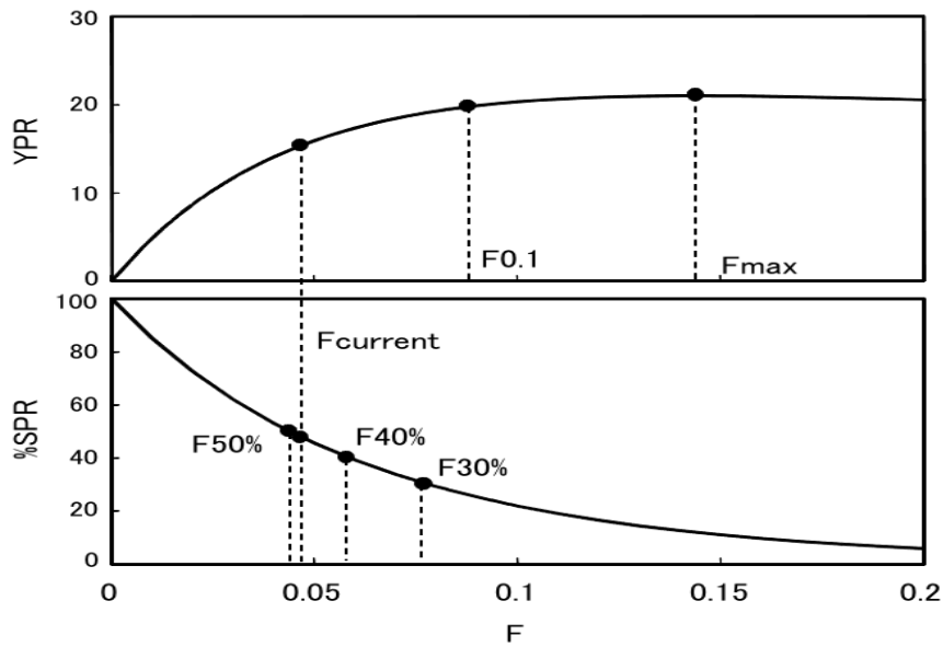
図 16. 様々な F と YPR 曲線および %SPR 曲線との関係
