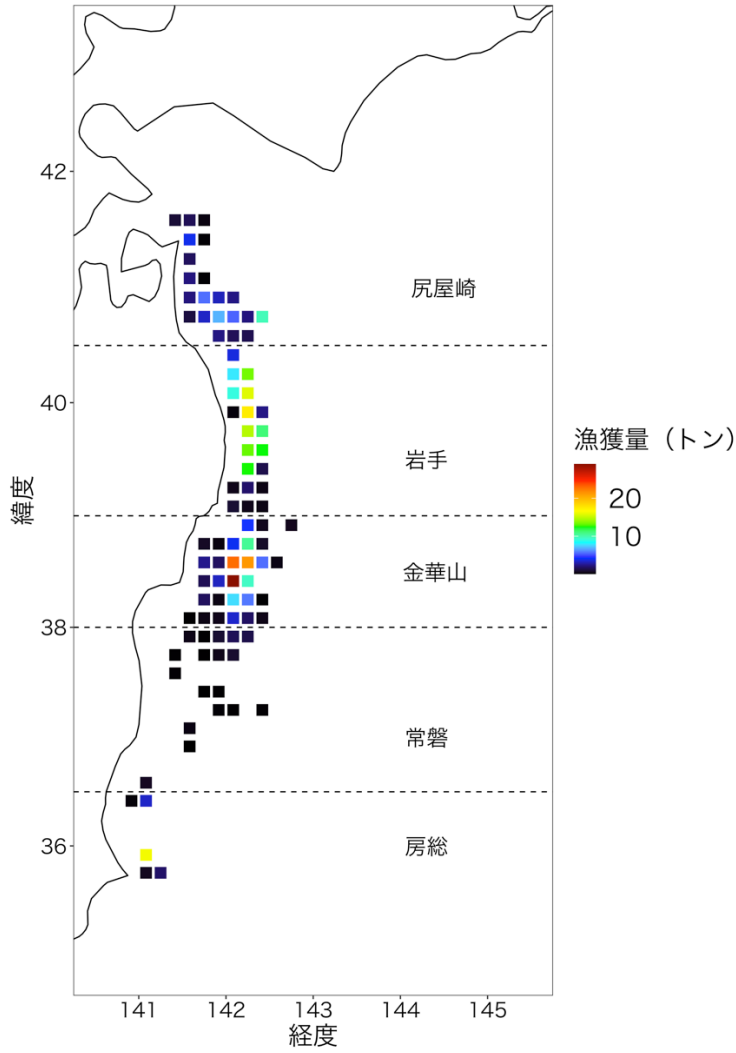
図4. 2019年の沖合底びき網漁業（沖底）の漁場 単位はトン。
