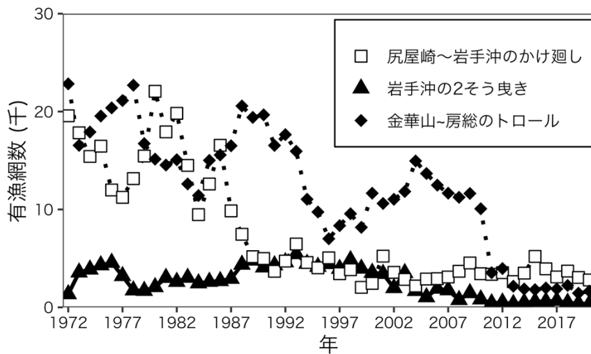
図6. 沖底による漁獲努力量の推移 2019年の値は暫定値。
