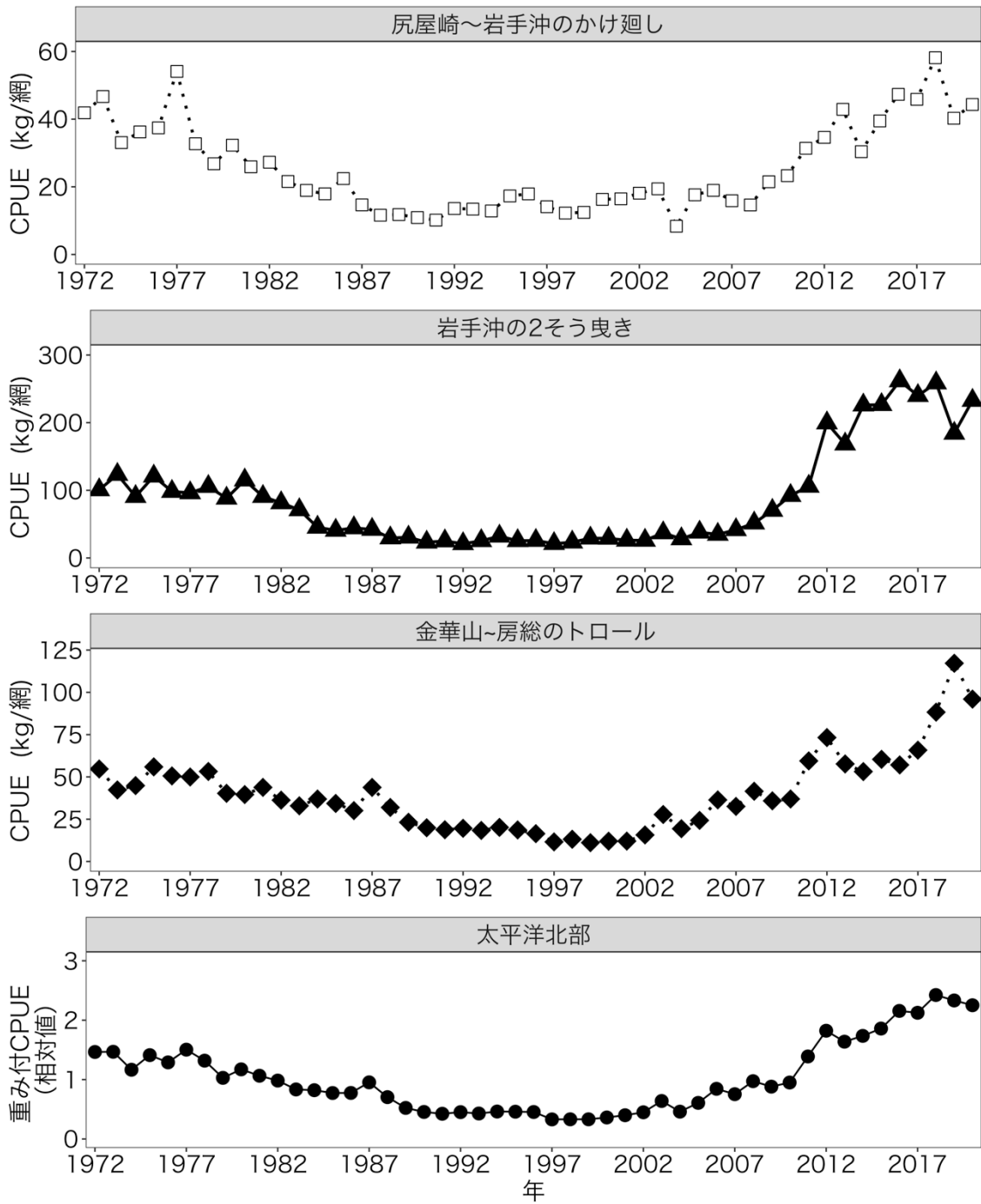
図 8. 沖底の CPUE および重み付け CPUE の推移 2020 年の値は暫定値。
