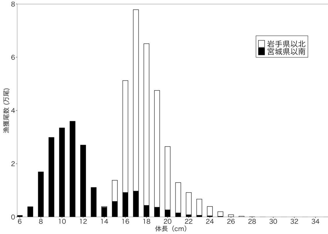
図9. 2020年の漁獲物の体長組成
