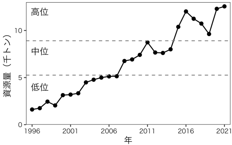
図10. 資源量 (1月時点) の推移 破線は水準の境界を示す。
