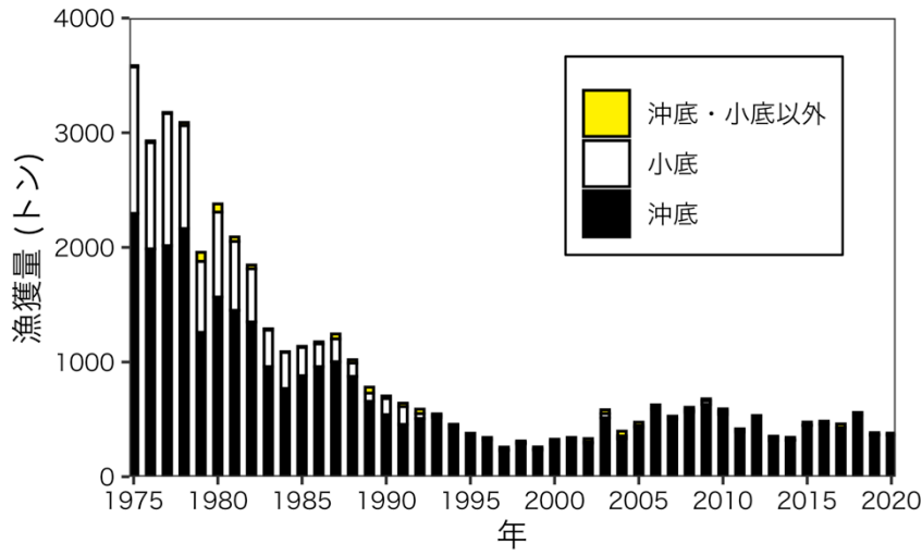
図5. 漁業種類別漁獲量の推移 2020年の値は暫定値。
