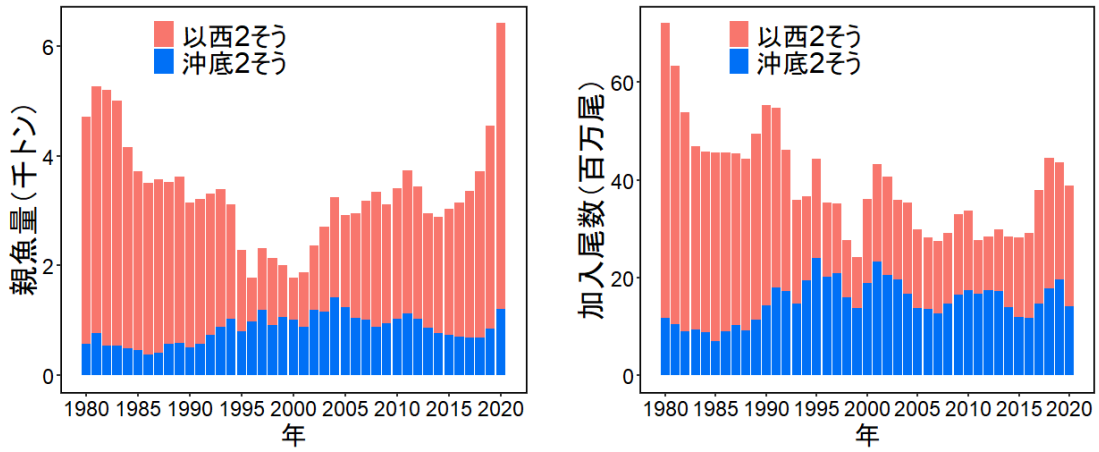
補足図 3-2. コホート計算から得られた親魚量（左）と加入尾数（右）
