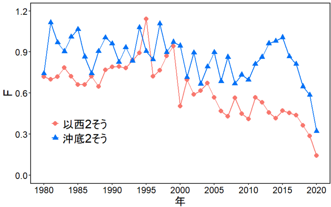
補足図 3-4. コホート計算から得られた漁獲係数 (F) の推移
