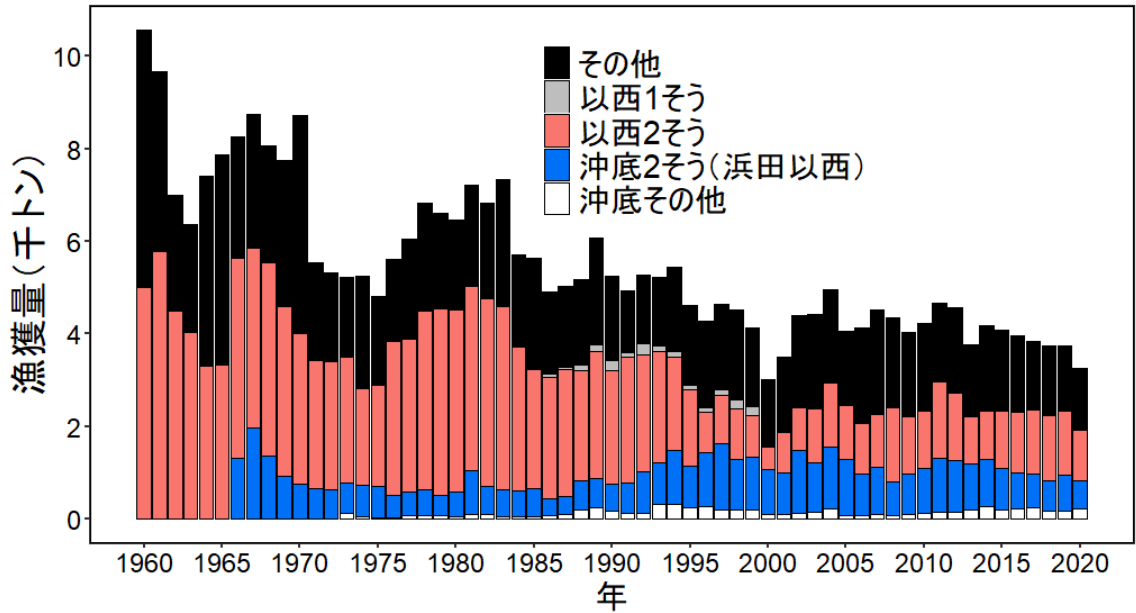
図8. キダイの漁業種類別漁獲量
