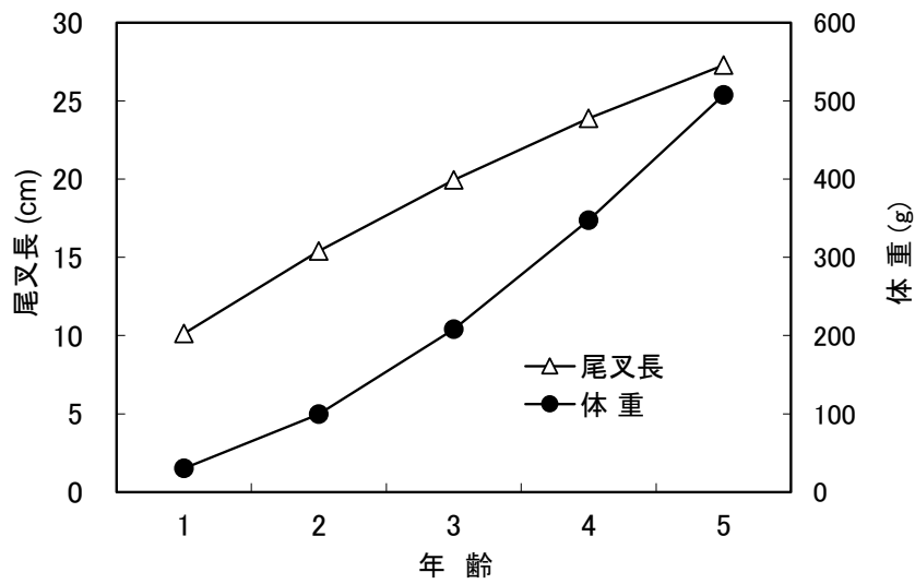
図2. キダイ年齢と成長
