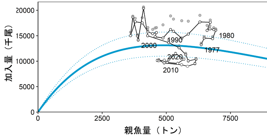
図4 再生産関係
