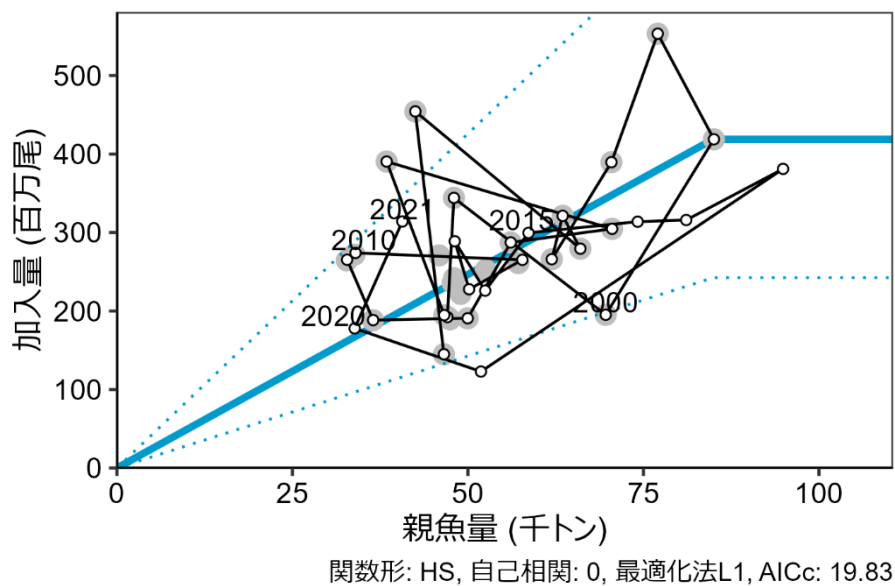
図 4-11. 親魚量と加入量の関係（再生産関係） 平成 31 年 4 月に開催された「管理基準値等に関する研究機関会議」（林ほか 2019）で提案された再生産関係式と再生産関係のプロット（灰色の丸印）。図中の再生産関係式（青実線）の上下の点線は、仮定されている再生産関係において観察データの 90%が含まれると推定される範囲である。実線と白抜きの丸印で示したのは今年度の評価で得られた再生産関係のプロット。図中の数字は年級群を示す。
