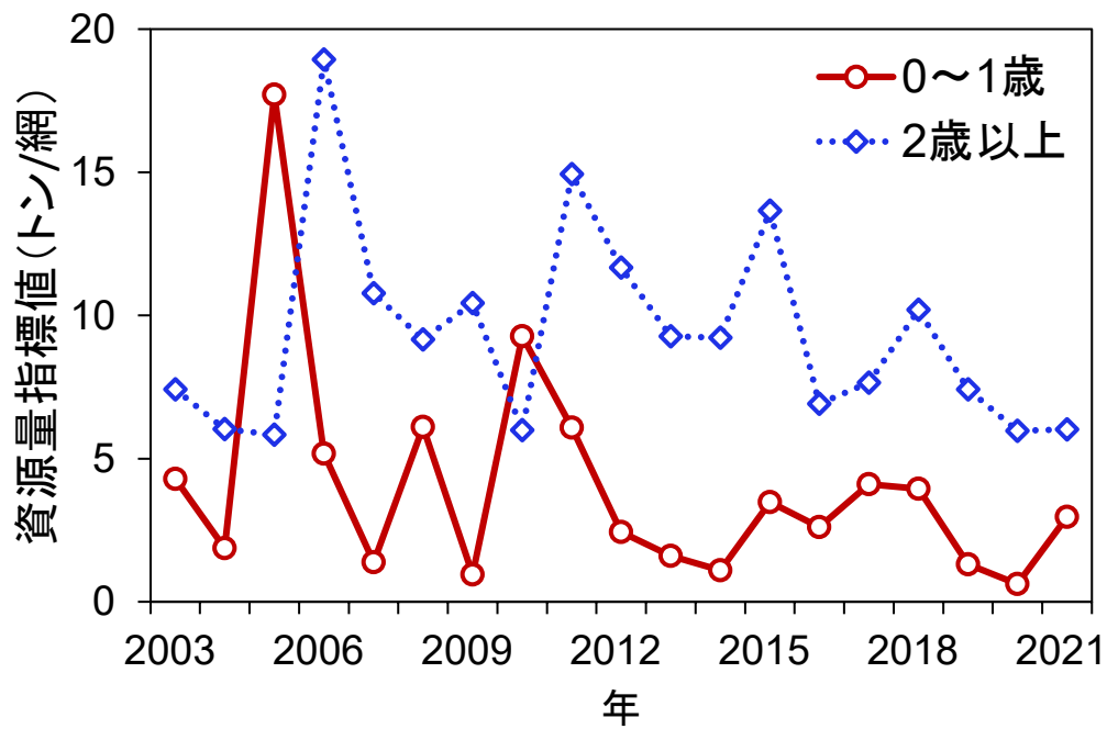
図 4-1. 東シナ海・日本海で操業する大中型まき網の銘柄別漁獲量から算出した年齢別の資源量指標値(トン/網)の推移(上図)と枕崎港に水揚げする中型まき網の資源量指標値の推移(下図)
