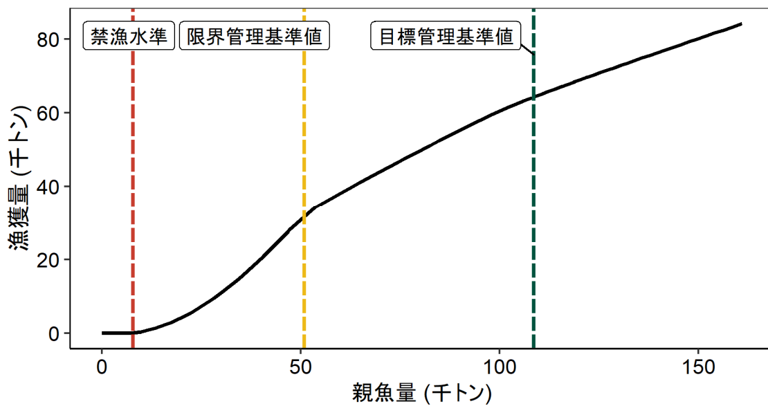
図 5-1. 漁獲管理規則（調整係数 \beta=0.95 の場合） 目標管理基準値（ SB_{target} ）はホッケ-スティック型再生産関係に基づき算出した SB_{msy} である。限界管理基準値（ SB_{limit} ）および禁漁水準（ SB_{ban} ）にそれぞれ標準値を用いている。黒破線： F_{msy} 、灰色破線：0.95 F_{msy} 、黒太線：HCR、赤破線：禁漁水準、黄色破線：限界管理基準値、緑色破線：目標管理基準値を示す。a) は縦軸を漁獲圧にした場合、b) は縦軸を漁獲量で表した場合である。b) については、漁獲する年の年齢組成によって漁獲量は若干異なるが、ここでは平衡状態における平均的な年齢組成の場合の漁獲量を示した。
