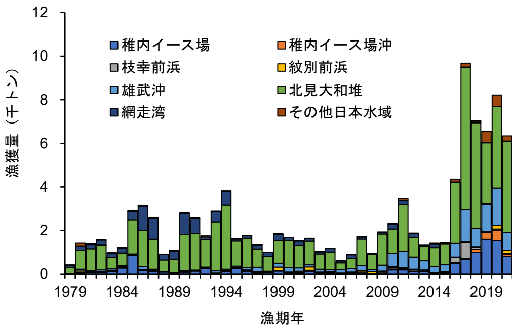
図4. 漁場別に区分したオホーツク海南部における沖底によるマダラ漁獲量
