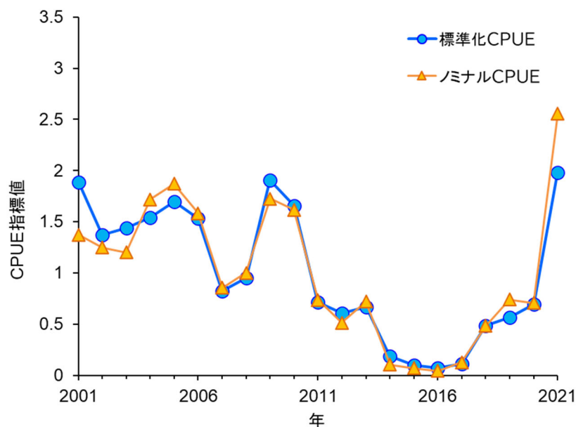
補足図 4-1. 羅臼漁協所属の刺網標準化 CPUE 指標値の推移
