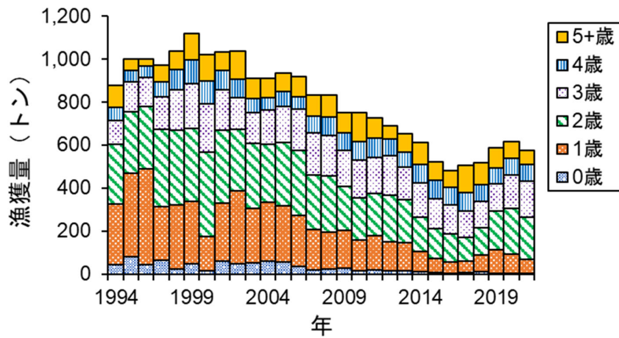
図 3-3. 年齢別漁獲量の推移
