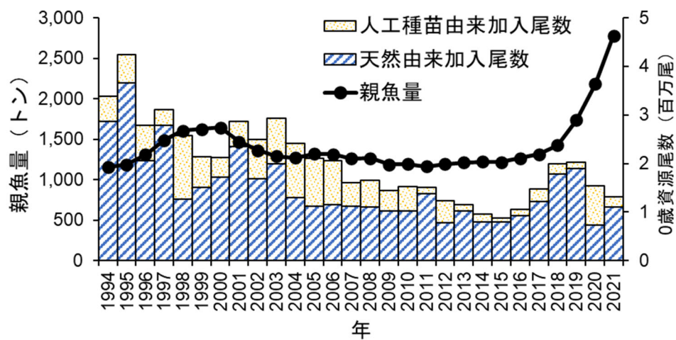
図 4-5. 親魚量および加入尾数の推移
