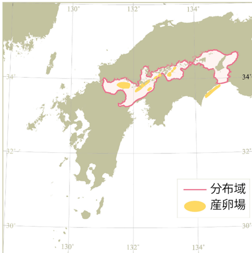
図 2-1. ヒラメ瀬戸内海系群の分布
