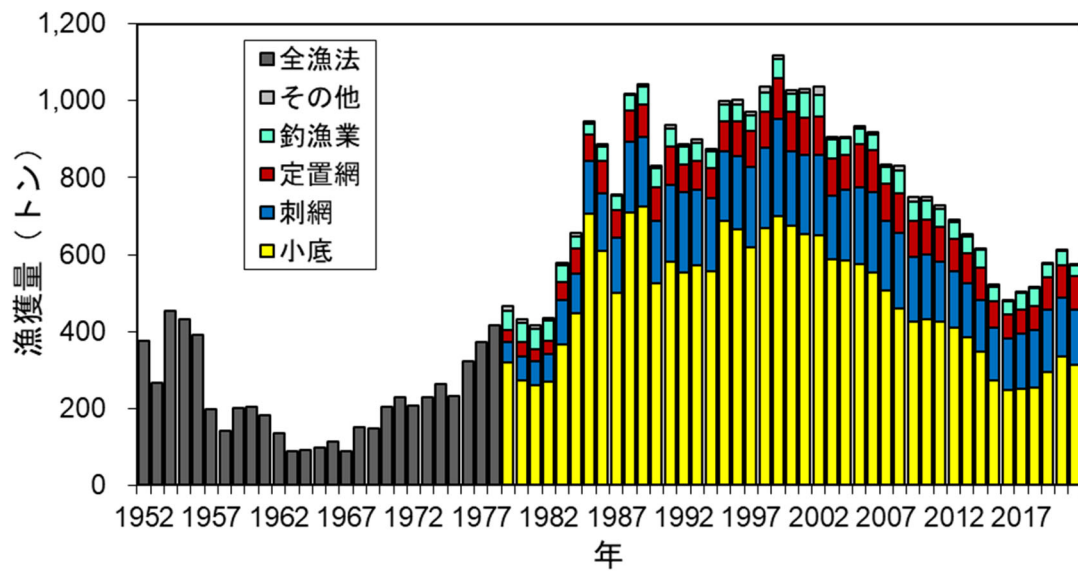
図 3-1. 漁業種類別漁獲量の推移 1978 年以前は全漁業合計値を示す。
