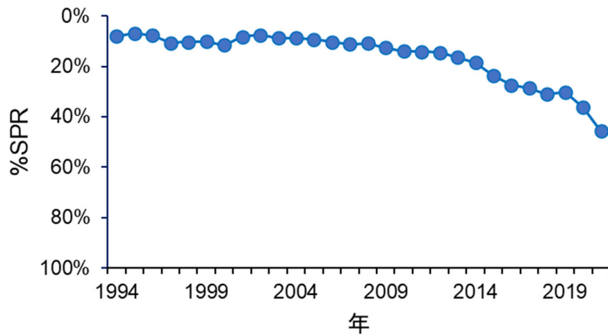
図 4-12. 各年における%SPR 値の経年推移 %SPR は漁獲がないときの親魚量に対する漁獲があるときの親魚量の割合を示し、Fが高い（低い）と%SPRは小さく（大きく）なる。
