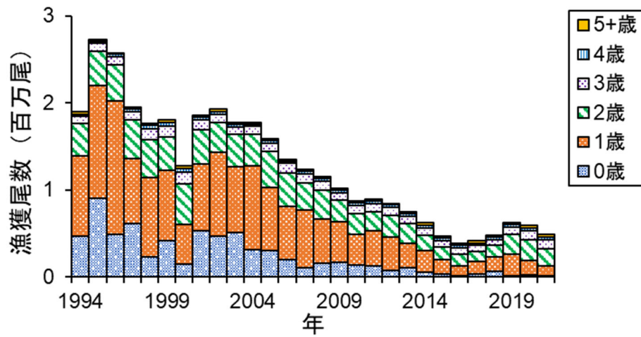
図 3-2. 年齢別漁獲尾数の推移
