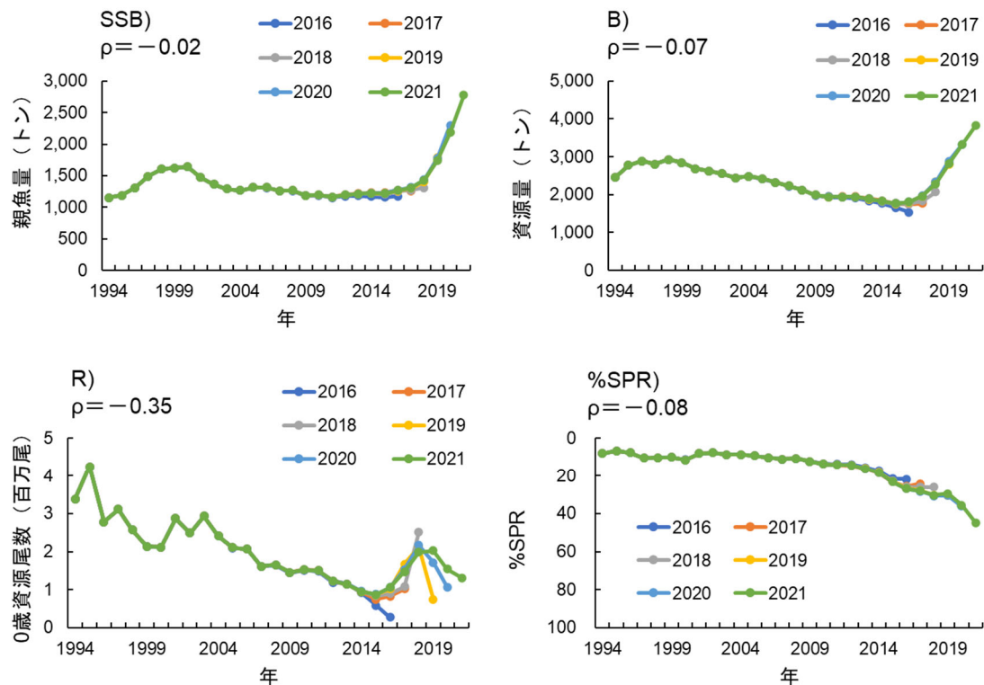
補足図 2-2. 親魚量 (SSB)、資源量 (B)、0 歳資源尾数 (R)、%SPR のレトロスペクティブ解析結果 凡例の数字は VPA 最終年を示す。
