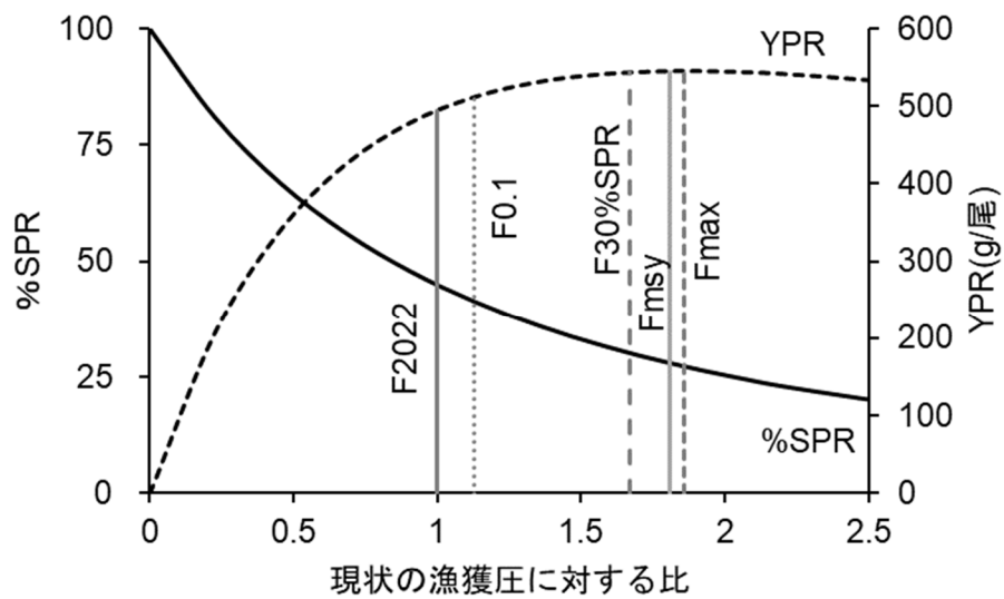
図 4-13. 現状の漁獲圧（F2022）に対する YPR、%SPR の関係
