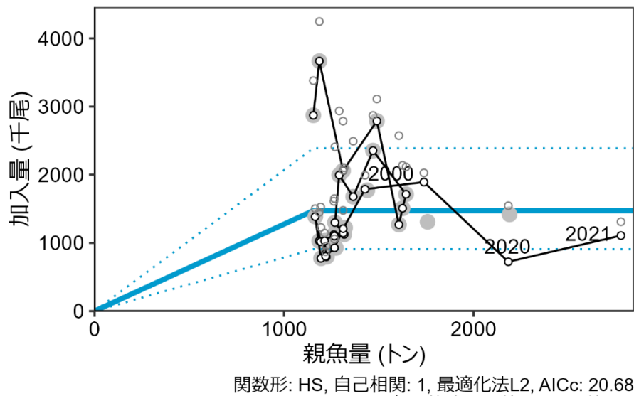
図 4-14. 親魚量と加入量の関係 青実線は本系群で適用した再生産関係式であり、上下の点線は、仮定されている再生産関係において観察データの 90%が含まれると推定される範囲である。再生産関係式のパラメータは令和 3 年 9 月に開催された「管理基準値等に関する研究機関会議」(山下ほか 2021) に示された値に基づき、塗りつぶしの灰色丸印はこの再生産関係推定時の親魚量と加入量を示す。白抜きの丸印は今年度評価において推定された 1994~2021 年の親魚量と加入量を示し、黒色は天然のみ、灰色は種苗放流を加味した加入量である。図中の数字は加入群の年級(生まれ年)を示す。
