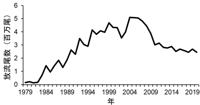
図 4-11. 1979 年以降の放流尾数の推移
