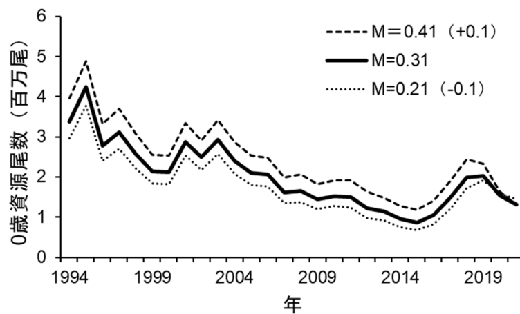
図 4-8. 自然死亡係数 M の値による 0 歳資源尾数の感度解析
