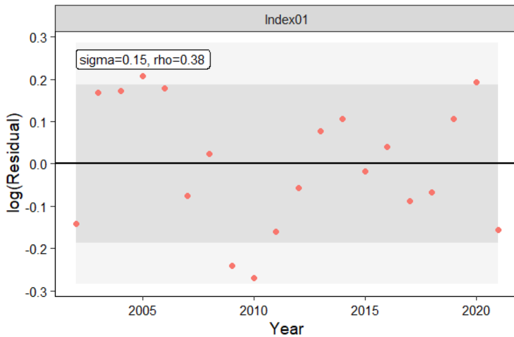
補足図 2-1. チューニング VPA における残差プロット
