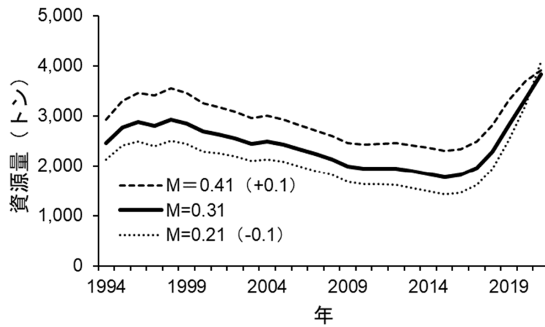
図 4-6. 自然死亡係数 M の値による資源量の感度解析
