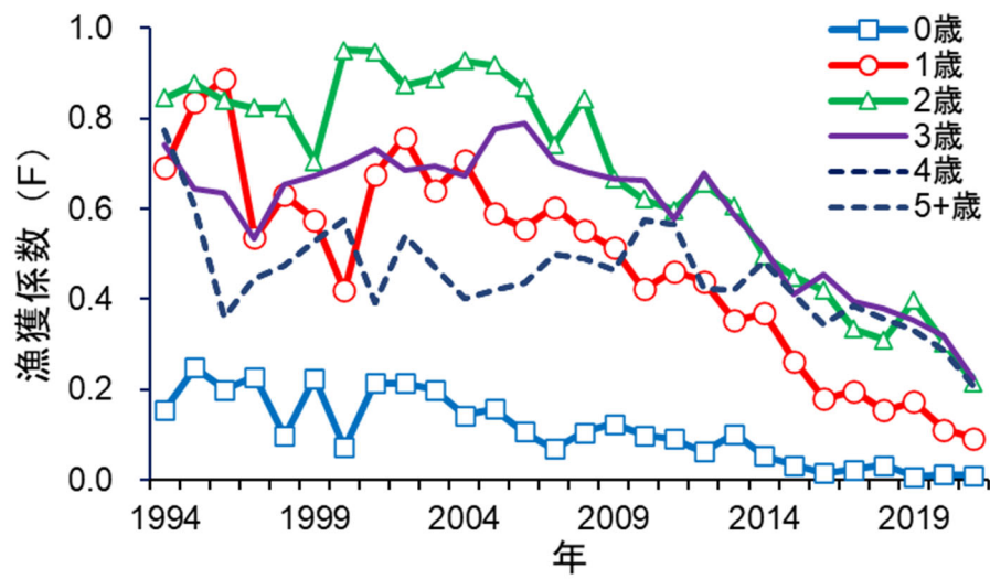
図 4-9. 年齢別漁獲係数 F の推移
