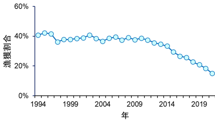
図 4-10. 漁獲割合の推移
