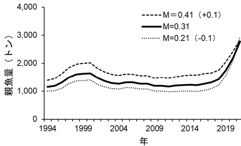
図 4-7. 自然死亡係数 M の値による親魚量の感度解析
