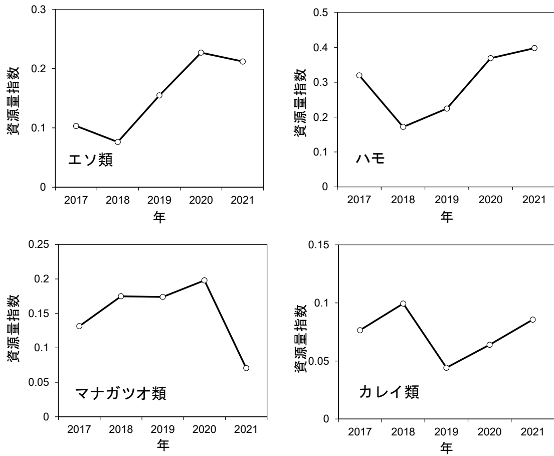
補足図 4-3. VAST を用いて推定された直近 5 年（2017～2021 年）のエソ類、ハモ、マナガツオ類、カレイ類の資源量指数（それぞれの魚種の解析に用いた期間の平均で規格化した値）
