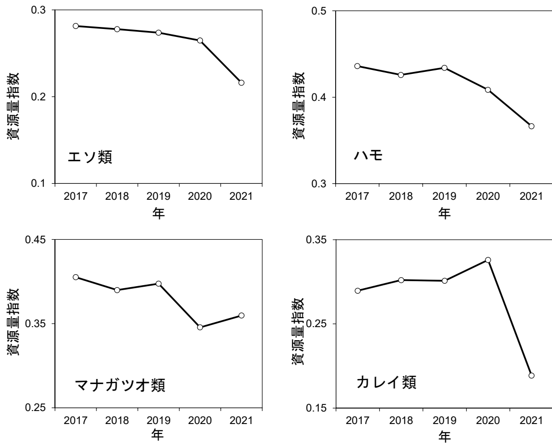
図 17. 直近 5 年（2017～2021 年）の我が国の漁場におけるエソ類、ハモ、マナガツオ類、カレイ類の資源量指数
