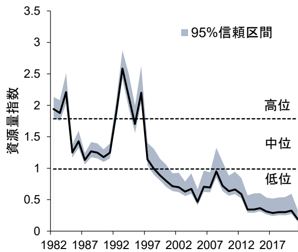
図 16. カレイ類の資源量指数の推移
