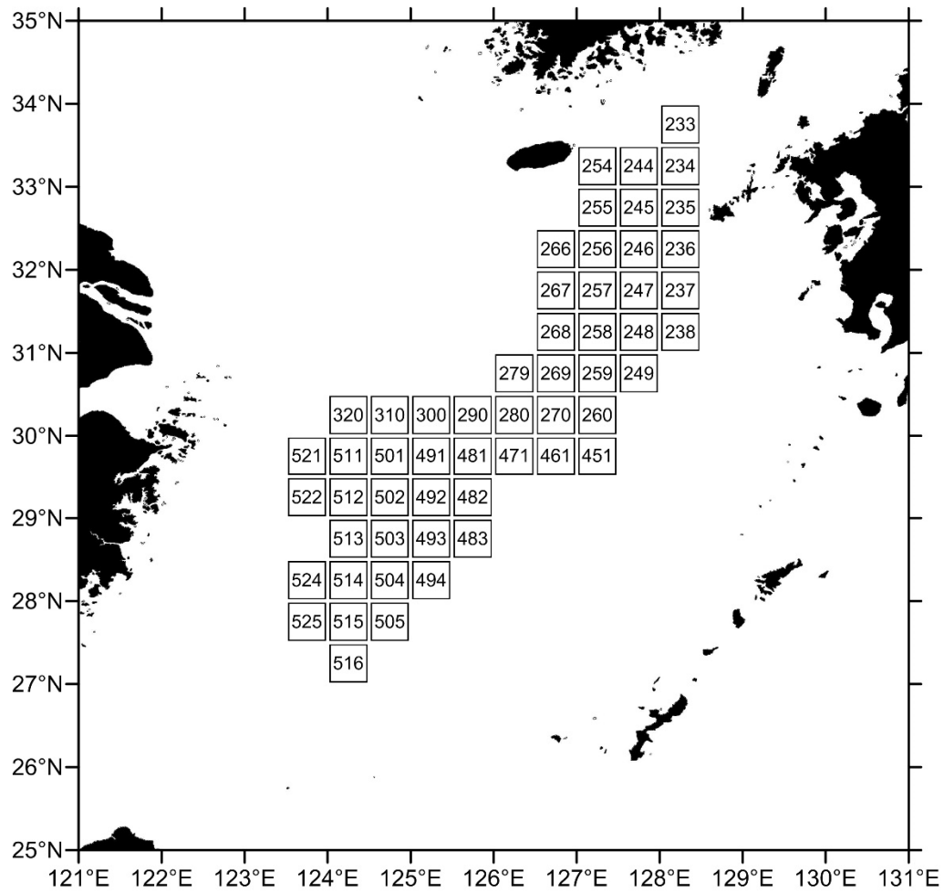
図 15. カレイ類の資源量指数解析に用いた漁区 (55 漁区)
