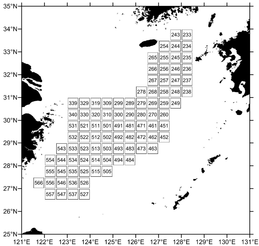
図 9. エソ類の資源量指数解析に用いた漁区 (91 漁区)
