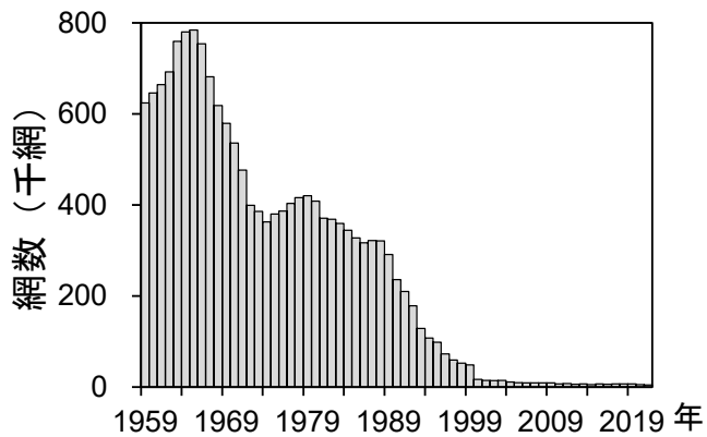
図 7. 以西底びき網漁業の漁獲努力量（1959～2021 年）
