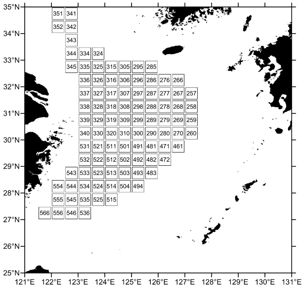
図 11. ハモの資源量指数解析に用いた漁区 (97 漁区)
