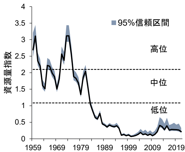
図 10. エソ類の資源量指数の推移
