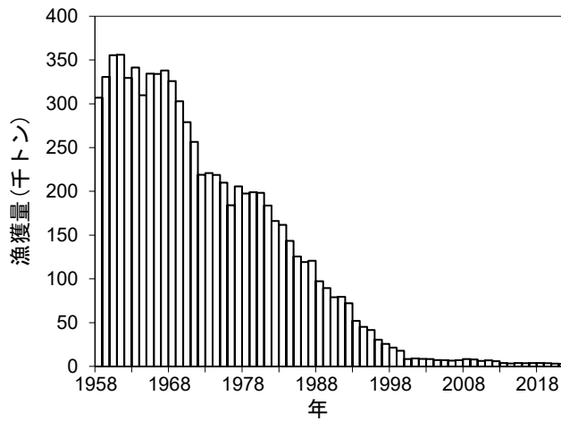
図 4. 以西底びき網漁業（2 そうびき）の漁獲量
