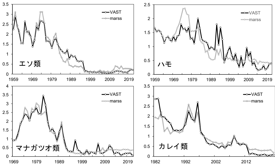
補足図 4-2. VAST および MARSS モデルを用いて推定されたエソ類、ハモ、マナガツオ類、カレイ類の資源量指数（それぞれの魚種の解析に用いた期間の平均で規格化した値）
