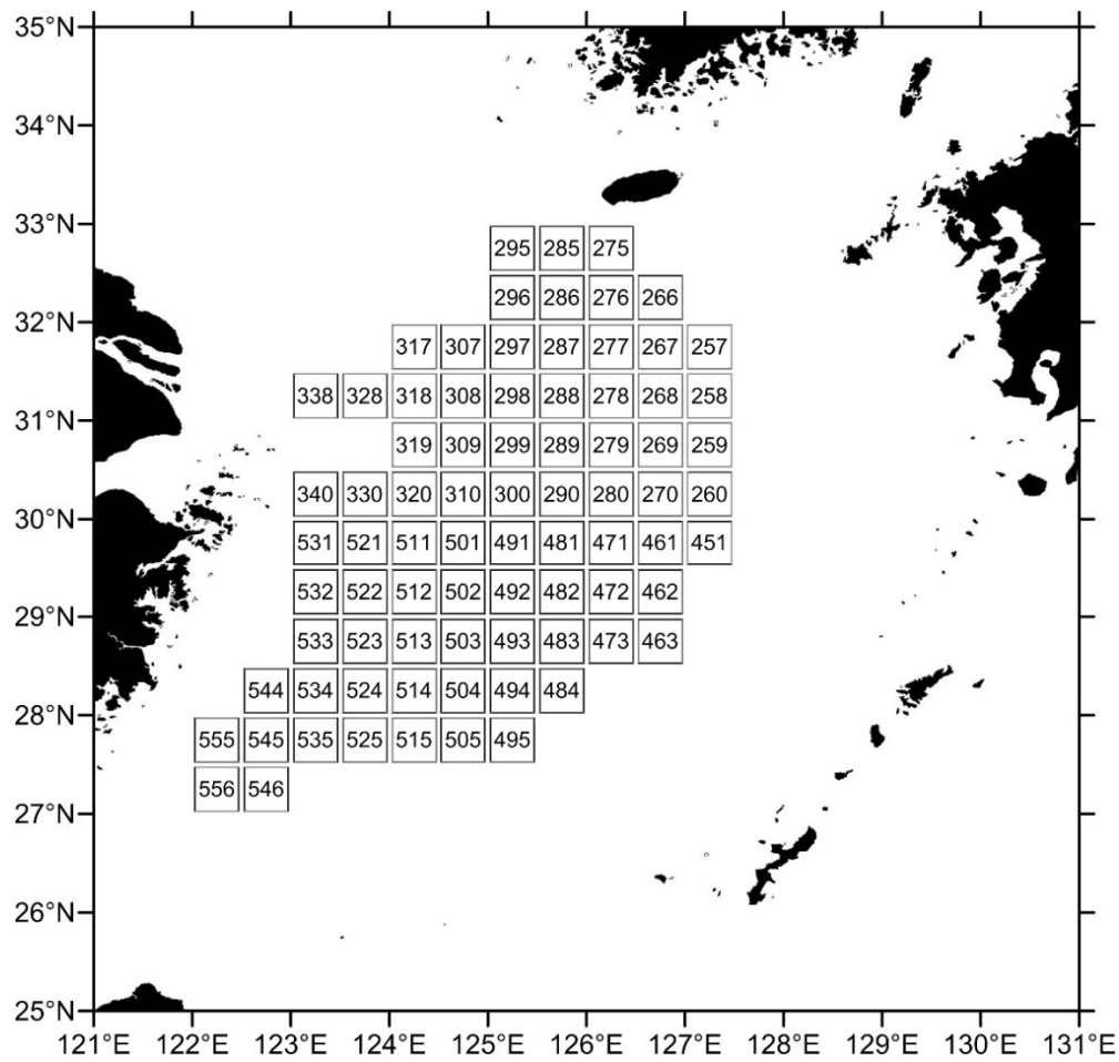
図 13. マナガツオ類の資源量指数解析に用いた漁区（80 漁区）
