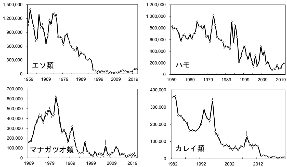
補足図 4-1. VAST を用いて推定されたエソ類、ハモ、マナガツオ類、カレイ類の資源量指数（バーは標準誤差）
