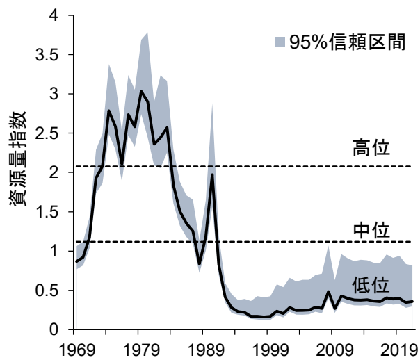
図 14. マナガツオ類の資源量指数の推移
