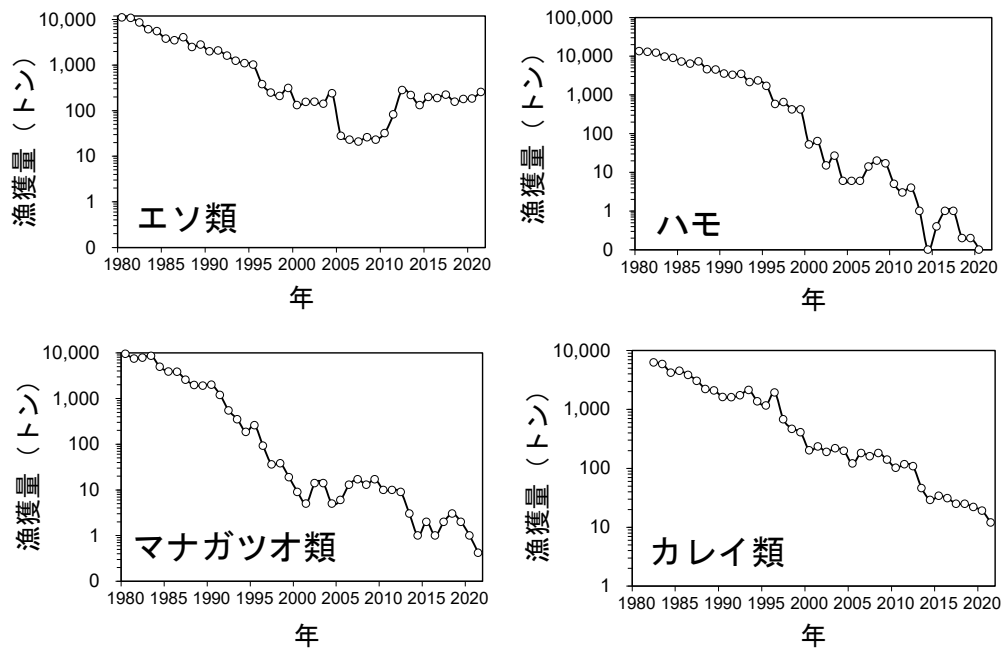
図 6. 以西底びき網漁業（2 そうびき）によるエソ類、ハモ、マナガツオ類、カレイ類の漁獲量（対数軸）
