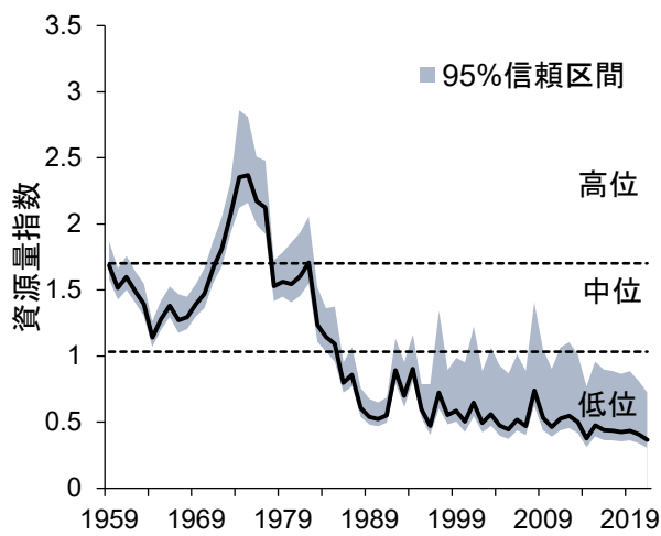
図 12. ハモの資源量指数の推移
