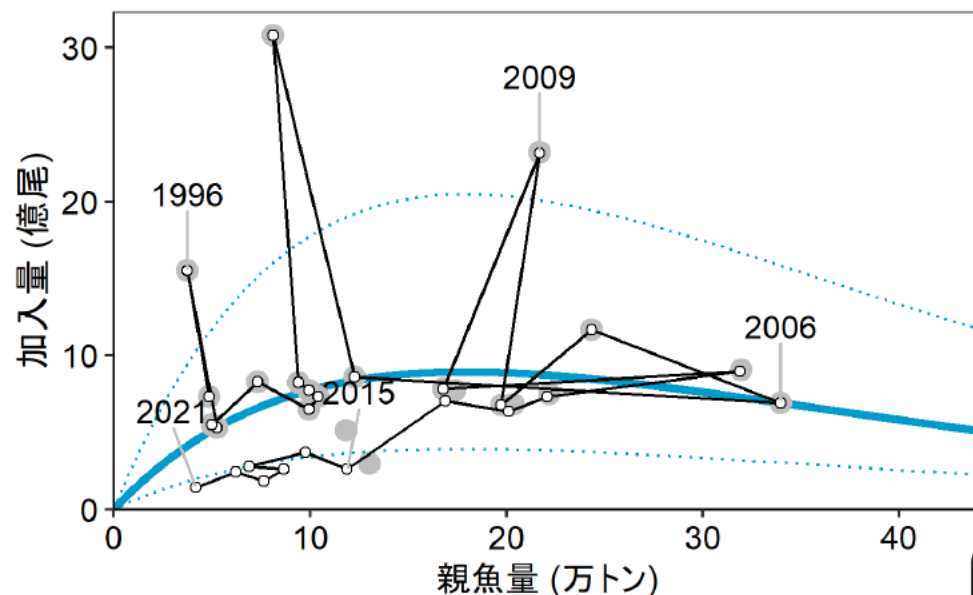
図6 再生産関係
