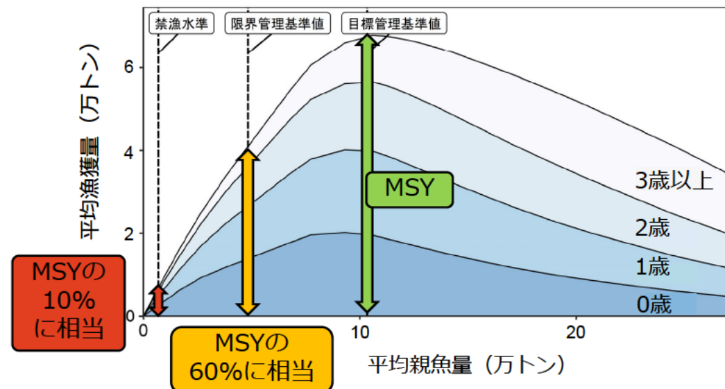
図7 管理基準値と禁漁水準
