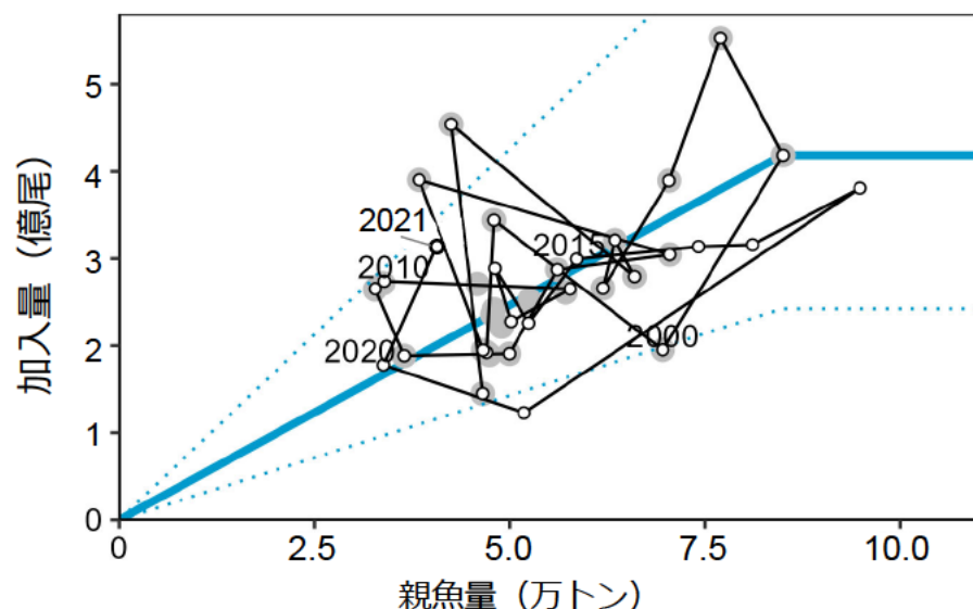
図6 再生産関係
