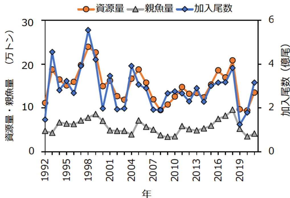
図4 資源量・親魚量・加入量
