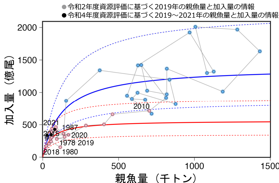
図6 再生産関係
