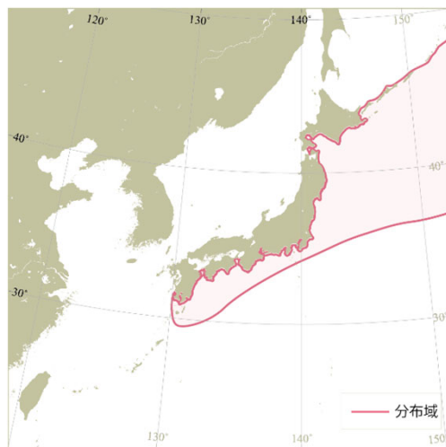
図1 分布域
