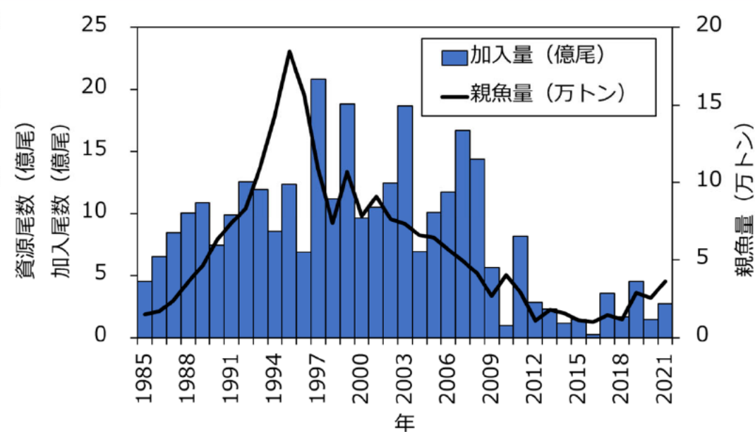
図5 加入量と親魚量の推移
