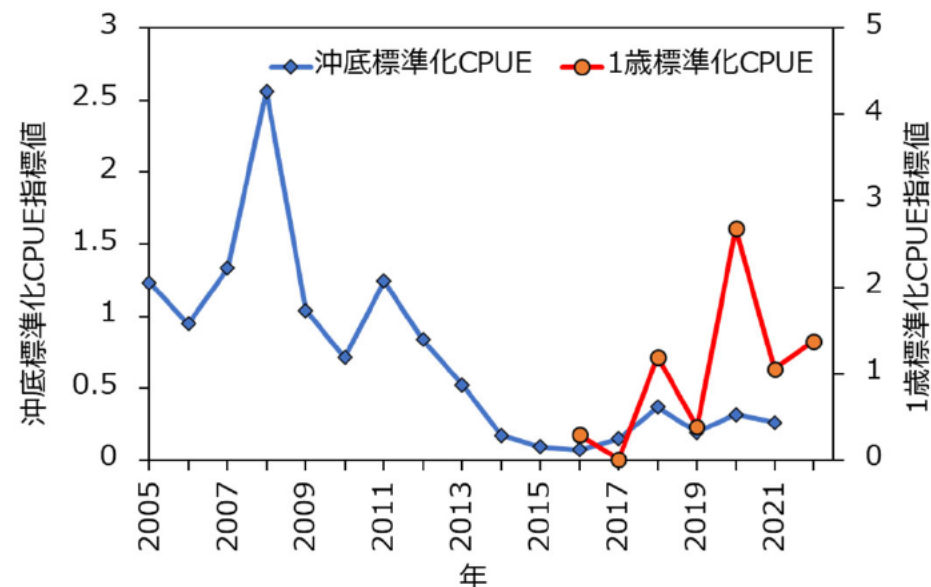
図3 資源評価に用いたCPUE指標値
