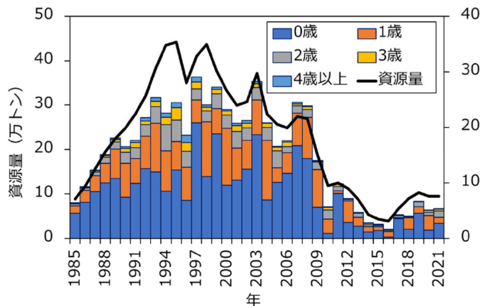
図4 資源量と年齢別資源尾数
