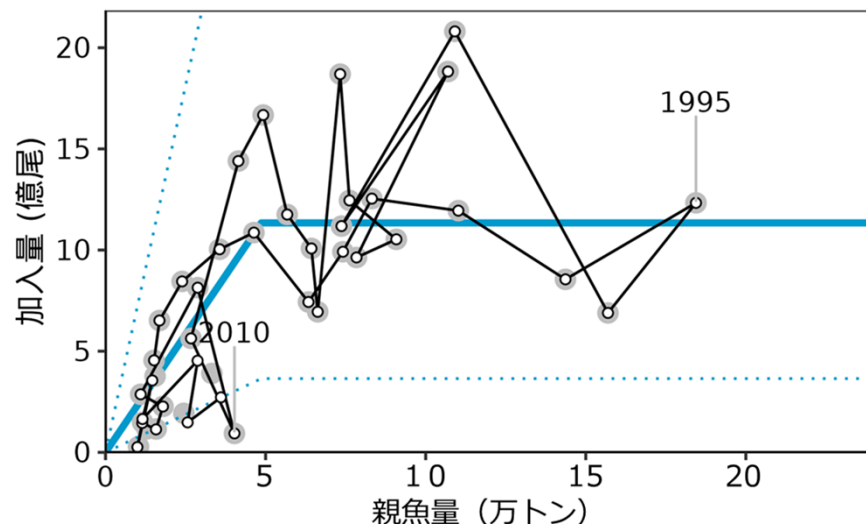
図6 再生産関係
