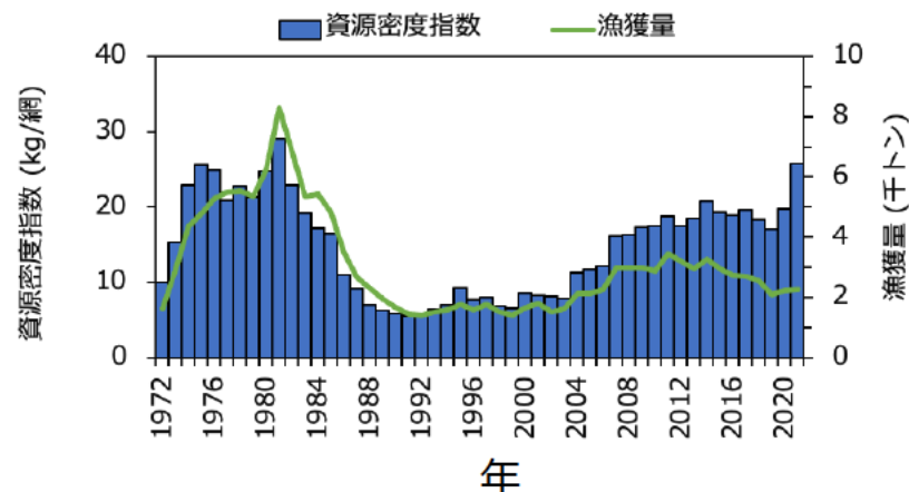
図3 沖合底びき網漁業における漁獲量と資源密度指数の推移
