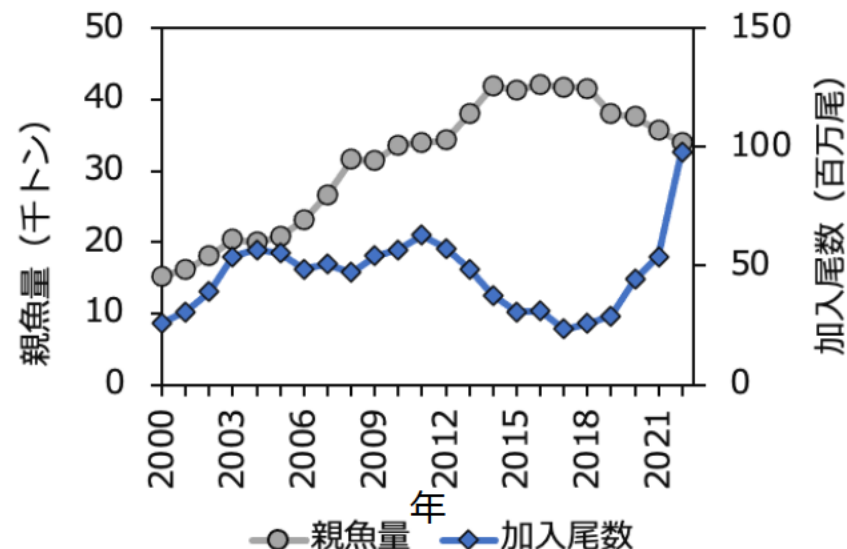
図5 加入量と親魚量の推移
