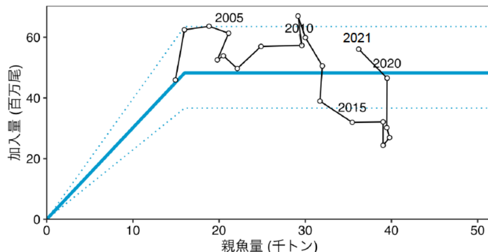
図6 再生産関係
