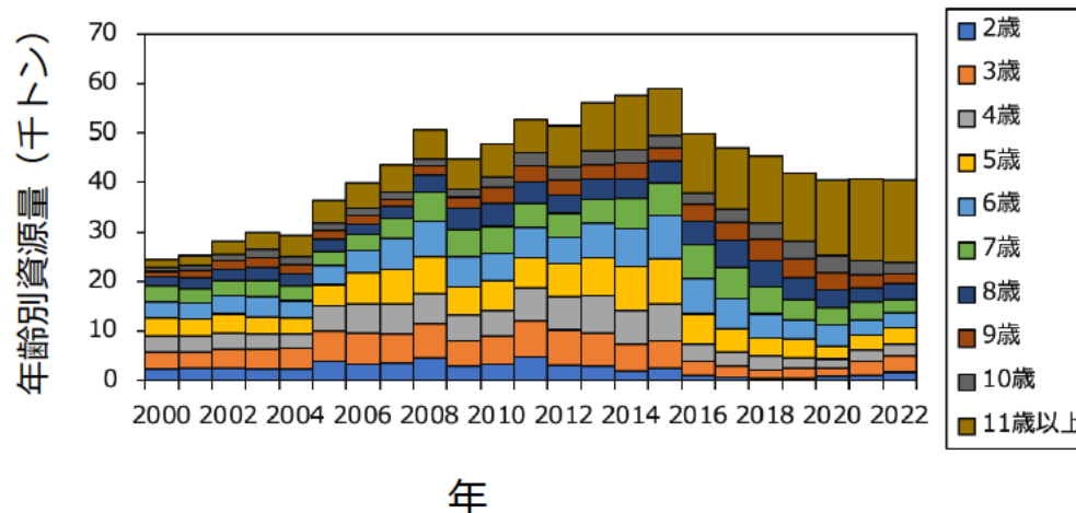
図4 年齢別資源量の推移
