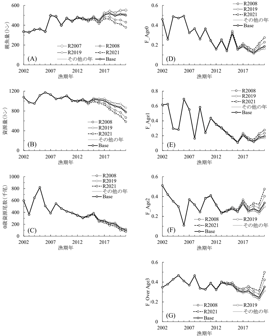
補足図 4-7. 2007 年以降チューニングとした場合の VPA 結果におけるジャックナイフ法によるチューニング指標値の影響解析結果 Base は各年の指標値を全て使用した場合。R2008、R2019、R2021 は、2008、2019、2021 年漁期それぞれの指標値を除外した場合。「その他の年」は Base データから大きな変化がない年を同一色で示した。なお、親魚量については、2007 年を除外した場合 (R2007) も Base データからの変化が大きいので、マーカーを追加した。(A)：親魚量 (単位：トン)、(B)：資源量 (単位：トン)、(C)：0 歳資源尾数 (単位：千尾)、(D)：0 歳 F、(E)：1 歳 F、(F)：2 歳 F、(G)：3 歳以上 F。
