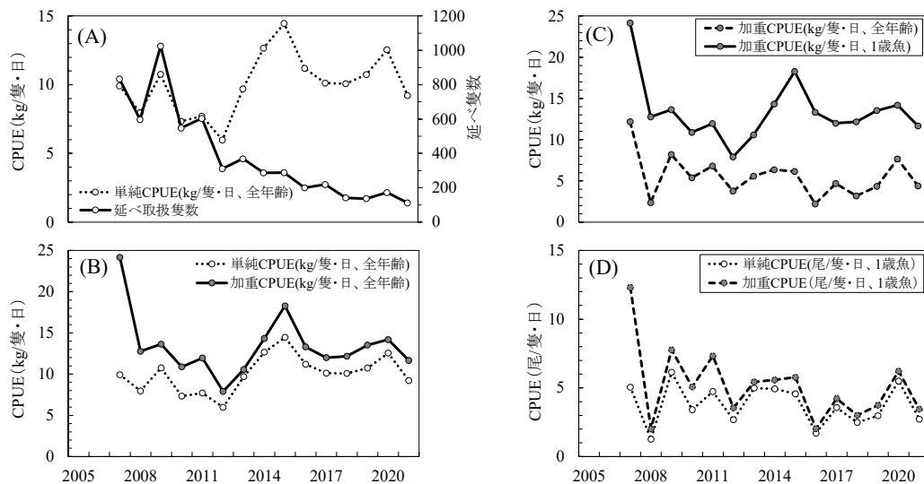
補足図 4-2. 大分県の漁協船別取扱量から抽出した、伊予灘以西・豊予海峡以北における、はえ縄の資源量指標値 (A): 漁獲努力量(延べ取扱隻数)と単純 CPUE (全年齢)、単位(kg/隻・日) (B): 単純 CPUE と加重 CPUE (全年齢) の比較。単位(kg/隻・日)。(C): 全年齢と 1 歳魚の加重 CPUE の比較。単位(kg/隻・日)。(D): 1 歳魚の加重 CPUE と単純 CPUE の比較。単位(尾/隻・日)。
