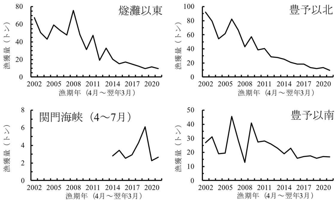
図 7. 海域別の漁獲量の推移 2 瀬戸内海および関門海峡 (4～7 月) の各海域区分における漁獲量の推移。海域区分は補足資料 7 を参照。関門海峡は、2014 年漁期以降の集計判明分を示す。
