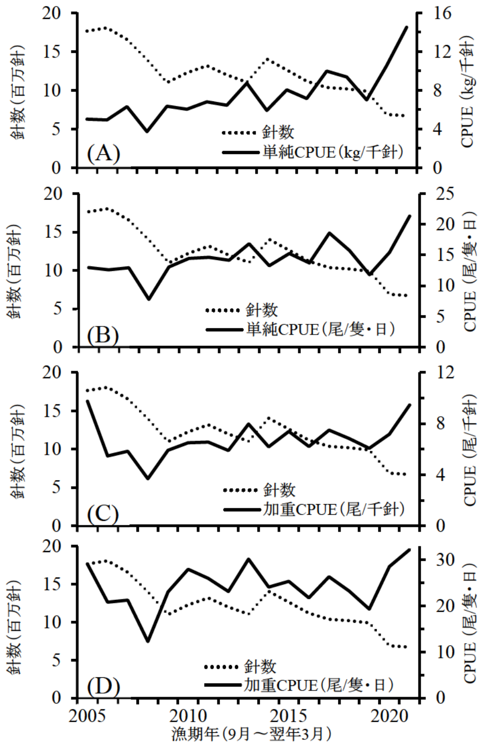
図 8. 九州・山口北西海域の 0 歳以上を対象としたはえ縄の努力量と CPUE の推移
