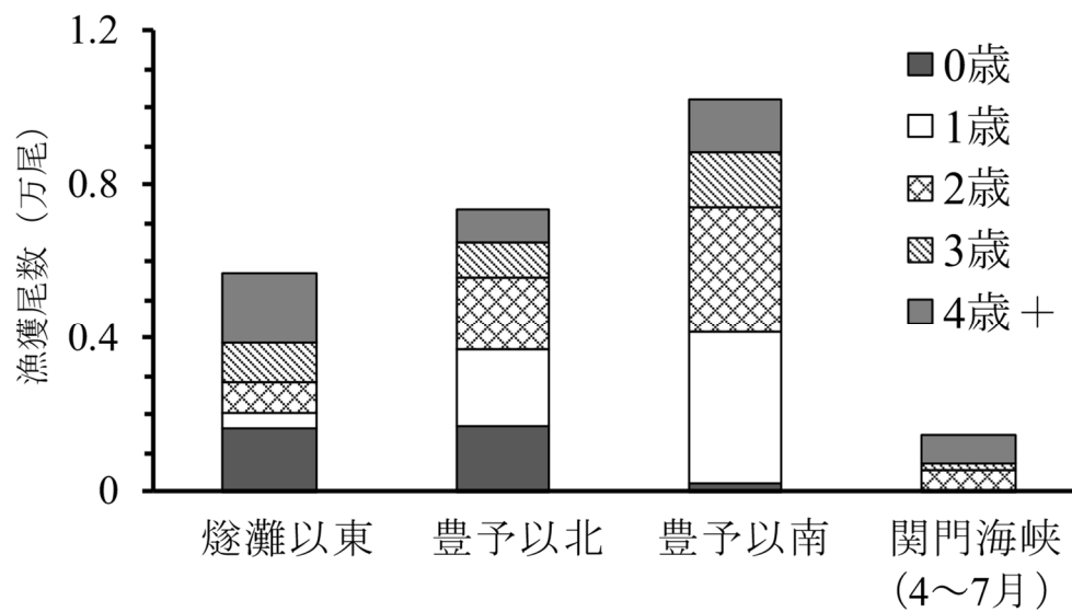
図 18. 2021 年漁期の瀬戸内海（4 月～翌年 3 月）および関門海峡（4～7 月）の海域別年齢別漁獲尾数
