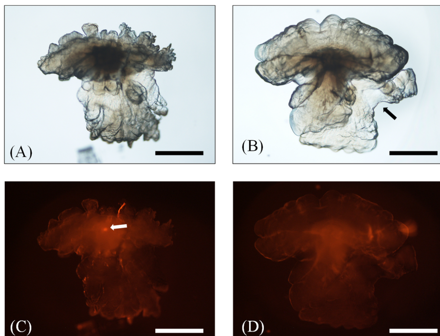
補足図 8-3. トラフグ当歳魚放流個体における耳石 (A) はささくれ状構造があり、奇形と判定、蛍光観察で ALC (白矢印) も確認され放流と判定されたケース。(B) は ALC は認められない (D) が外部形態では薄片化 (黒矢印) があり、放流と判定。
