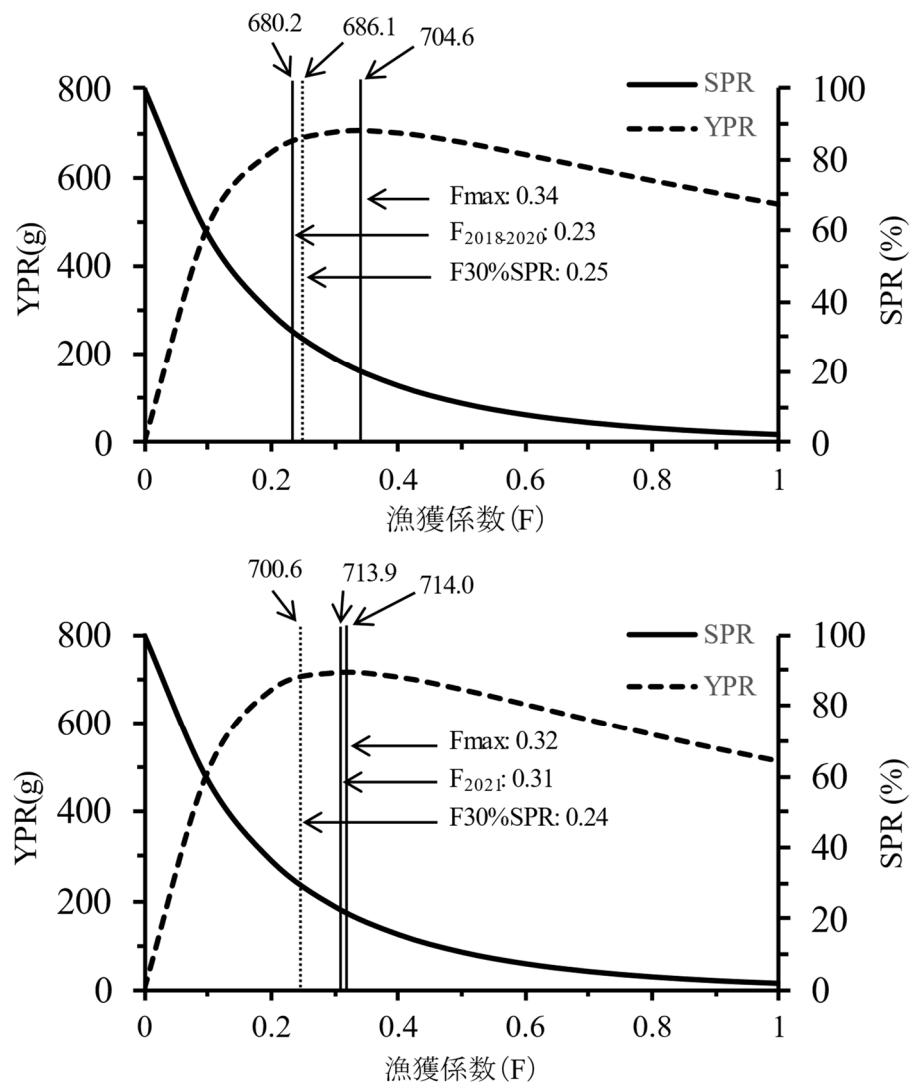
図 24. F と YPR、SPR の関係。(A) 現状の F を 2018～2020 年漁期の年齢別 F 単純平均とした場合。(B) 現状の F を 2021 年漁期の年齢別 F 単純平均とした場合。各縦棒の位置と矢印で示した数値はそれぞれの生物学的管理基準(F)と YPR を示す。
