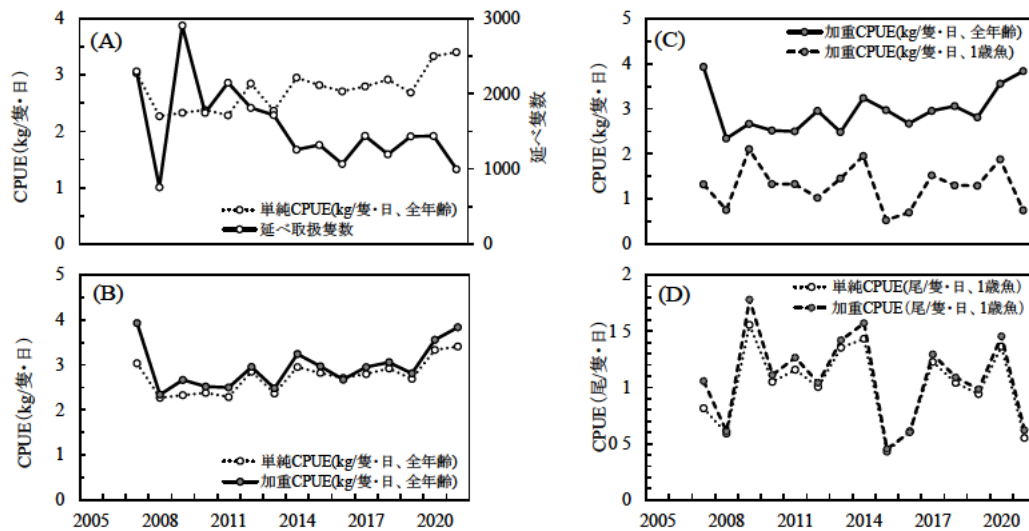
補足図 4-3. 大分県の漁協船別取扱量から抽出した、伊予灘以西・豊予海峡以南における、釣りの資源量指標値 (A): 漁獲努力量 (延べ取扱隻数) と単純 CPUE (全年齢)、単位 (kg/隻・日) (B): 単純 CPUE と加重 CPUE (全年齢) の比較。単位 (kg/隻・日)。(C): 全年齢と 1 歳魚の加重 CPUE の比較。単位 (kg/隻・日)。(D): 1 歳魚の加重 CPUE と単純 CPUE の比較。単位 (尾/隻・日)。
