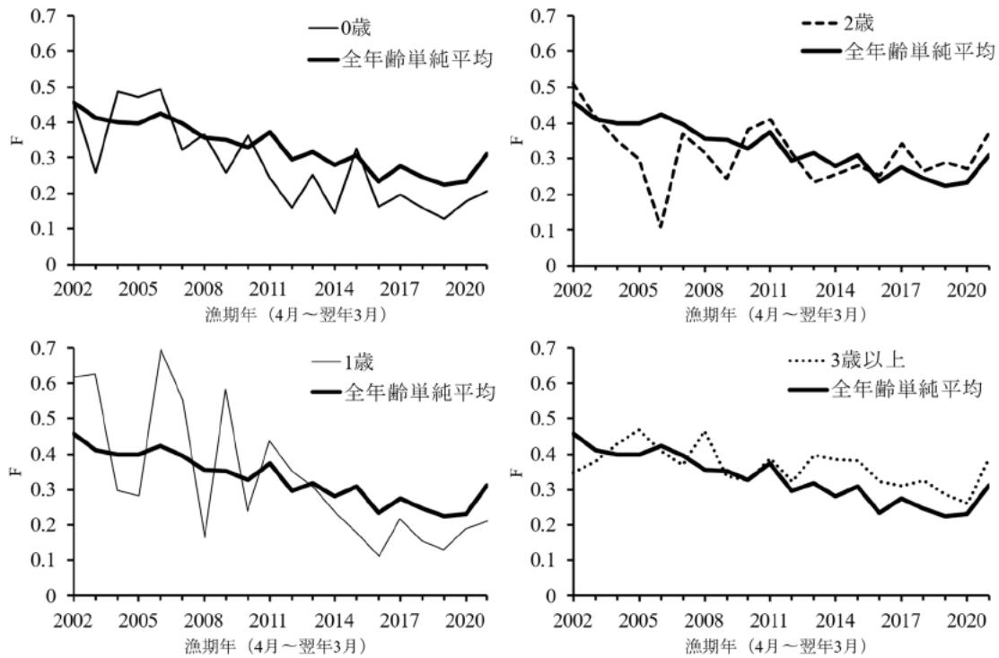
図 23. 各年齢の F と、F の全年齢平均の推移
