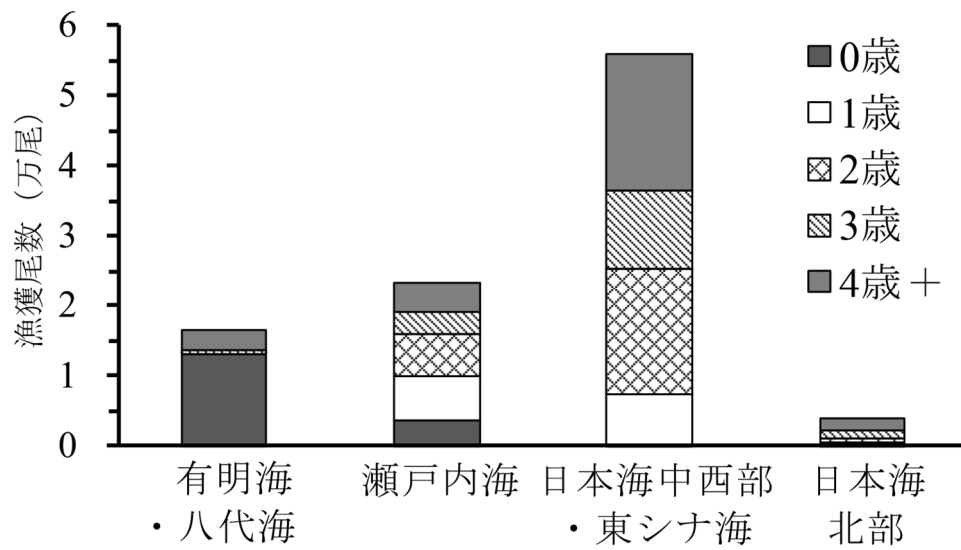
図 17. 2021 年漁期（4 月～翌年 3 月）の海域別年齢別漁獲尾数
