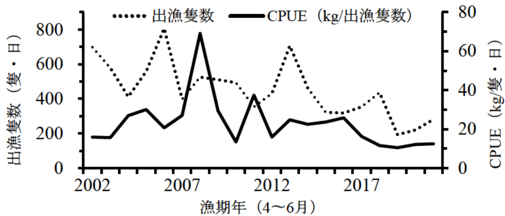
図 10. 備讃瀬戸における標本漁協の 1 歳以上 (1 kg 以上) を対象とした袋待網の努力量と単純 CPUE の推移 2019 年以降は一標本漁協について出漁隻数、単純 CPUE を算出
