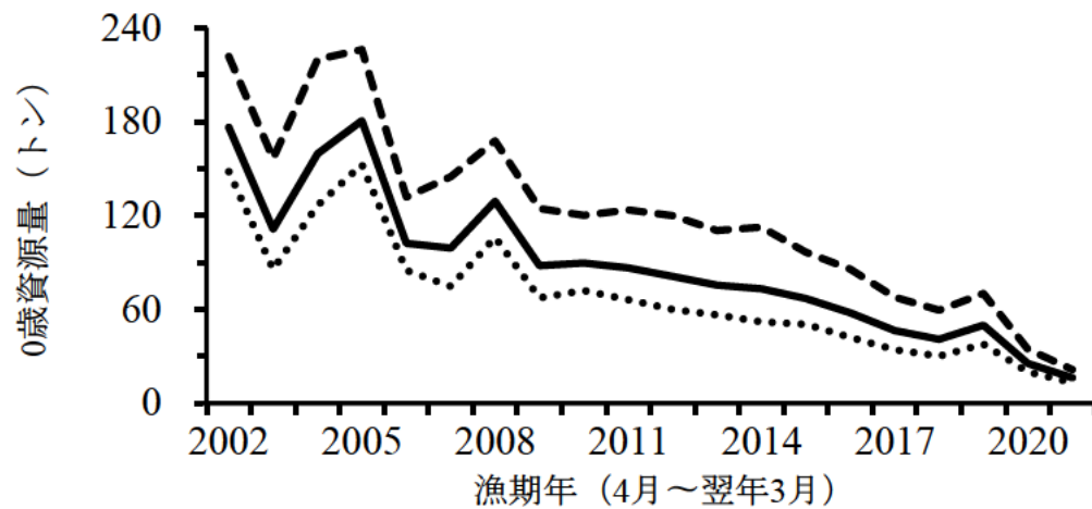
図 22. 0歳資源量についての自然死亡係数 M の感度分析
