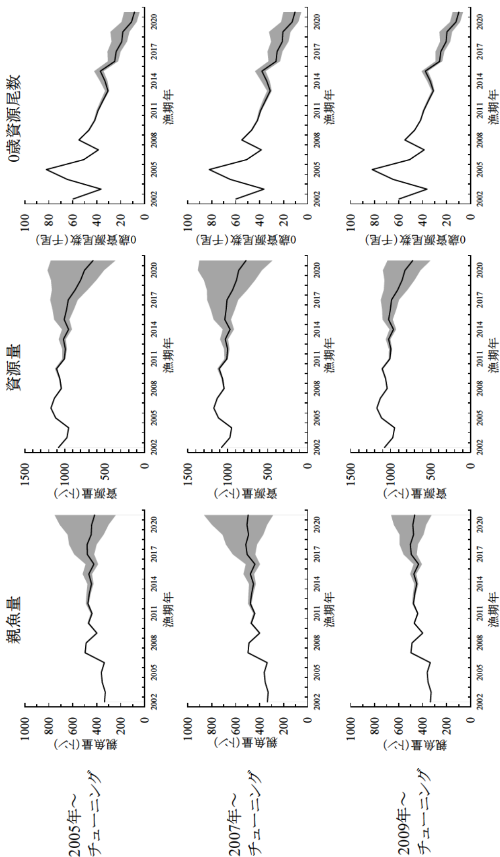
補足図 4-13. チューニング期間の違いによる、ブートストラップ信頼区間推定結果 グレーの範囲は 95%信頼区間を示す。
