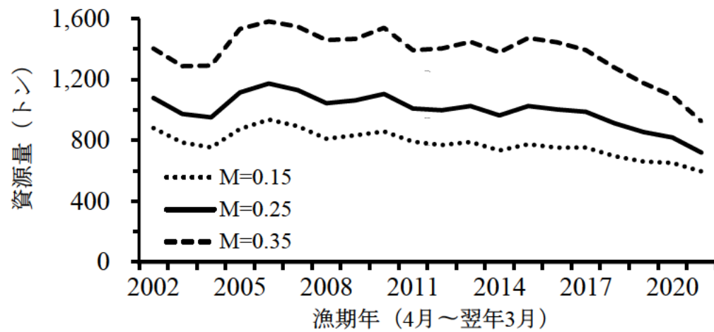
図 20. 資源量についての自然死亡係数 M の感度分析
