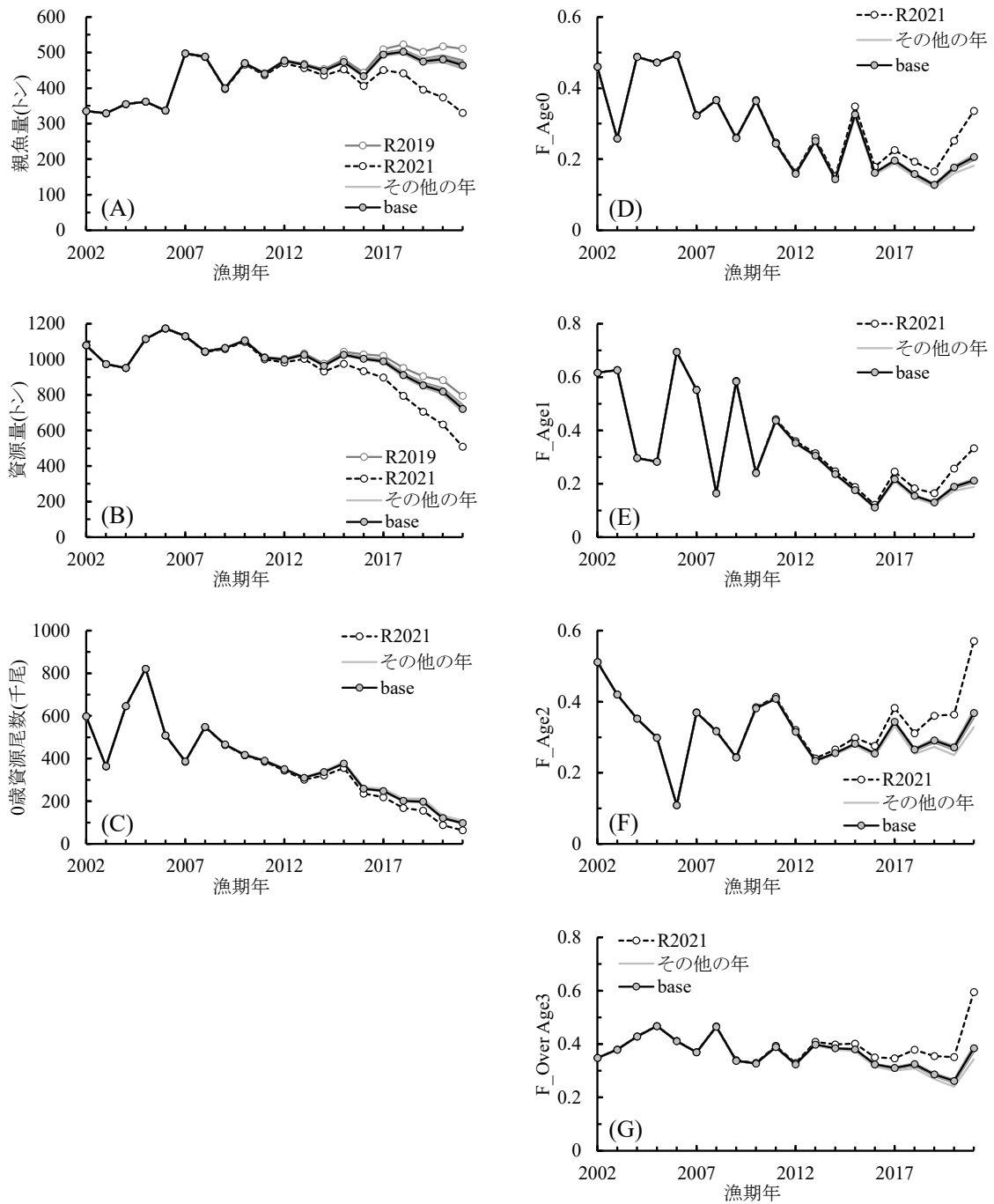
補足図 4-8. ジャックナイフ法による 2009 年以降チューニングとした場合の VPA モデル診断結果 Base は各年の指標値を全て使用した場合。R2021 は、2021 年漁期それぞれの指標値を除外した場合。「その他の年」は Base データから大きな変化がない年を同一色で示した。なお、親魚量と資源量については、2019 年を除外した場合 (R2019) も Base データからの変化が大きいため、マーカーを追加した。(A) : 親魚量 (単位 : トン)、(B) : 資源量 (単位 : トン)、(C) : 加入尾数 (単位 : 千尾)、(D) : 0 歳 F、(E) : 1 歳 F、(F) : 2 歳 F、(G) : 3 歳以上 F。
