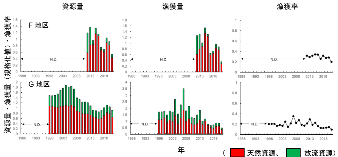
図7. 岩手県南部2地区（F～G）の資源量（左）、漁獲量（中）、漁獲率（右）の推定値 漁法は鉤どり。資源量および漁獲量の値は2012～2021年の平均値を1とした規格化値 で示した。資源量と漁獲率はF地区でDeLury法、G地区でVPAにより推定した。
