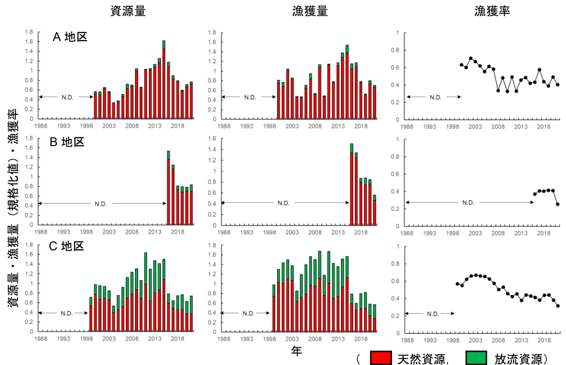
図5. 岩手県北部3地区（A～C）の資源量（左）、漁獲量（中）、漁獲率（右）の推定値 漁法は潜水漁業。資源量および漁獲量の値は2012～2021年の平均値を1として規格化 値で示した。資源量と漁獲率はいずれも DeLury 法により推定した。
