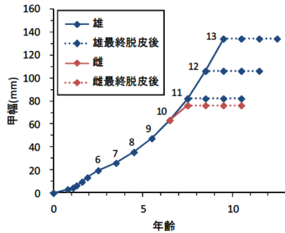
図 2. ズワイガニの年齢、脱皮年齢および甲幅の関係
