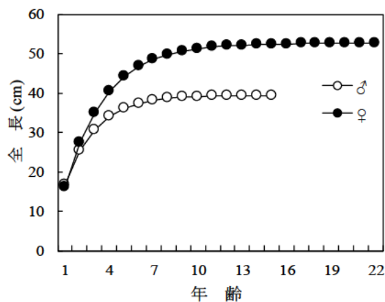
図3. サメガレイの成長
