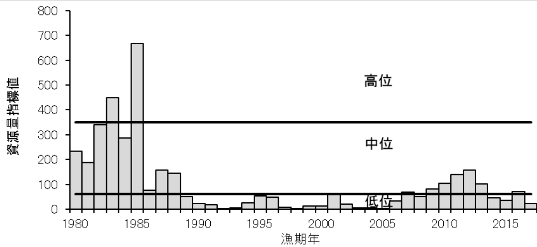
図 12. スケトウダラオホーツク海南部のオッターコントロールの資源量指標値の推移
