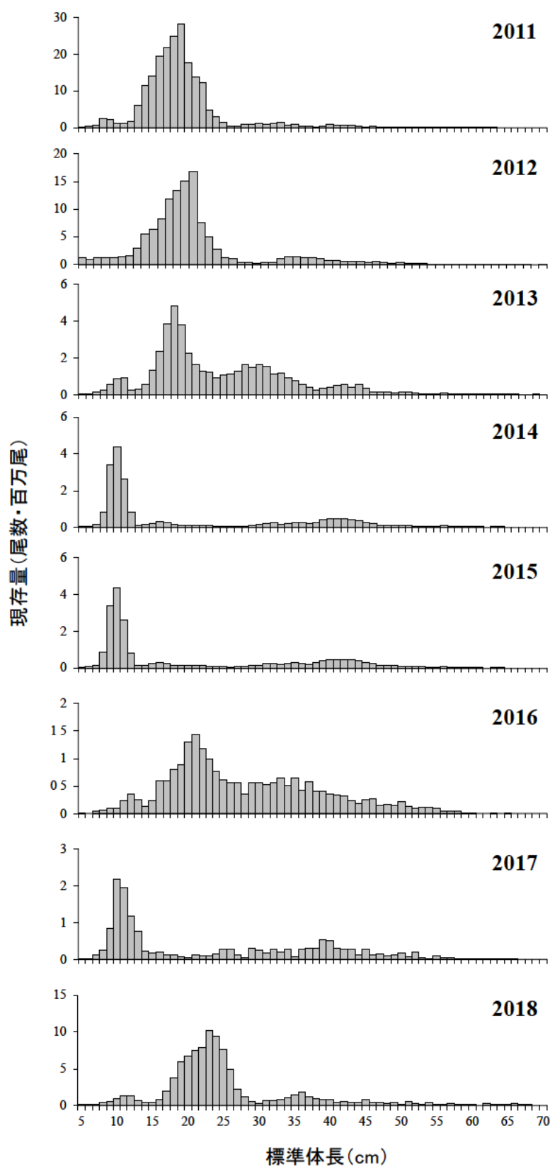
補足図 2-2. オホーツク海底魚資源調査で漁獲されたスケトウダラの体長組成 2018 年の値は暫定値。
