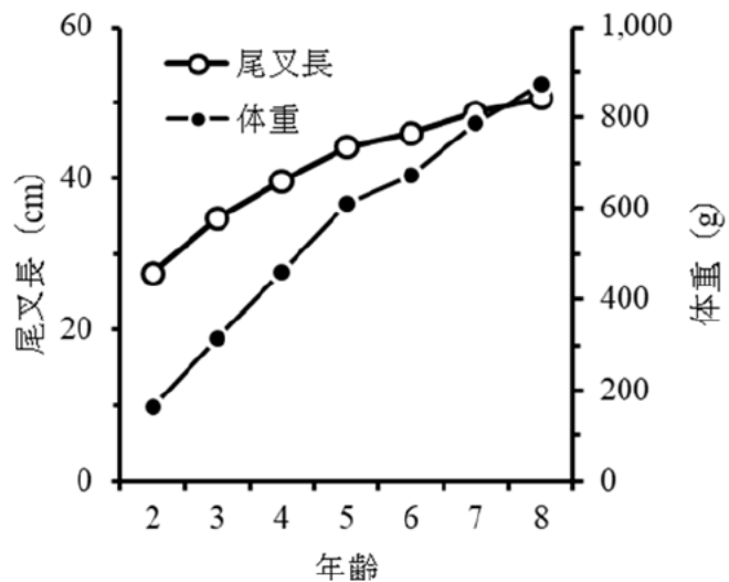
図 3. スケトウダラオホーツク海南部の成長 2008～2017 年漁期の沖底漁獲物の 4～7 月における平均尾叉長と平均体重
