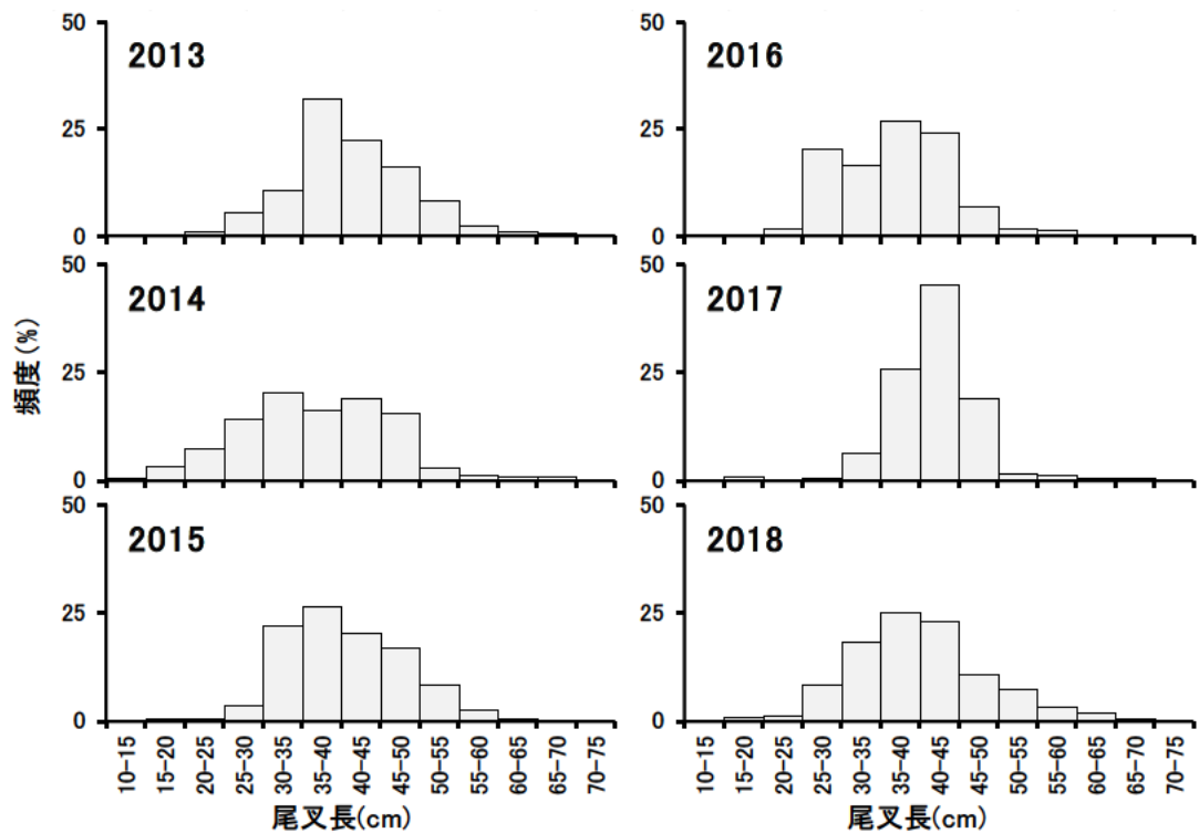
図 10. 紋別・網走港に 4～7 月に水揚げされたスケトウダラの尾叉長組成 2018 年の値は暫定値
