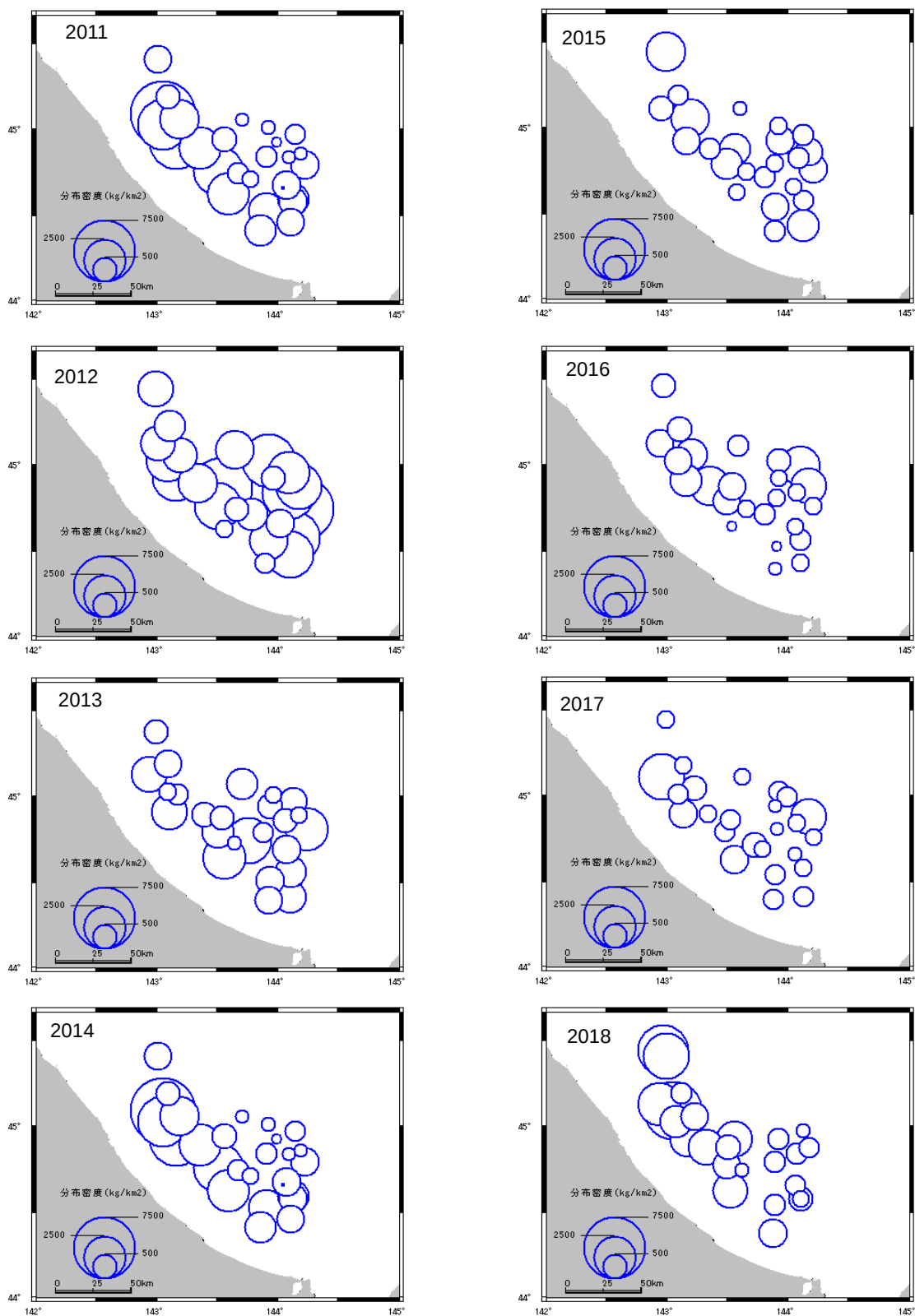
補足図 2-3. 2011～2018 年の各トロール調査点におけるスケトウダラ分布密度 ×は漁獲がなかった調査点を示す。2018 年の値は暫定値。
