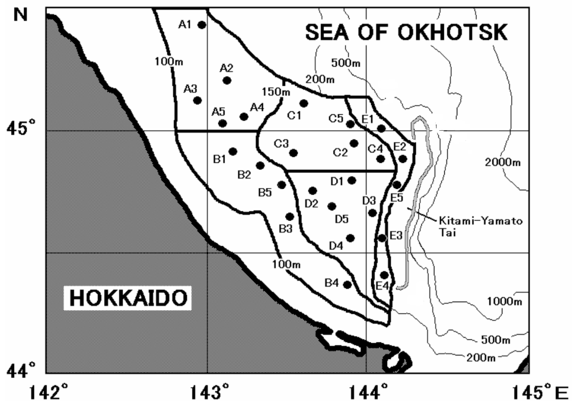
補足図 2-1. オホーツク海底魚資源調査の調査海域および調査定点の配置 太線は現存量の推定範囲（北側は 45.30°N と日ロ中間線、東側は北見大和堆の 200 m 等深線と 144.10°E、陸側は 100 m 等深線をもとに設定）
