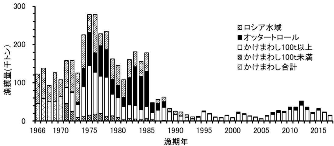
図 4. 沖合底びき網漁業によるスケトウダラオホーツク海南部の漁獲量の推移
