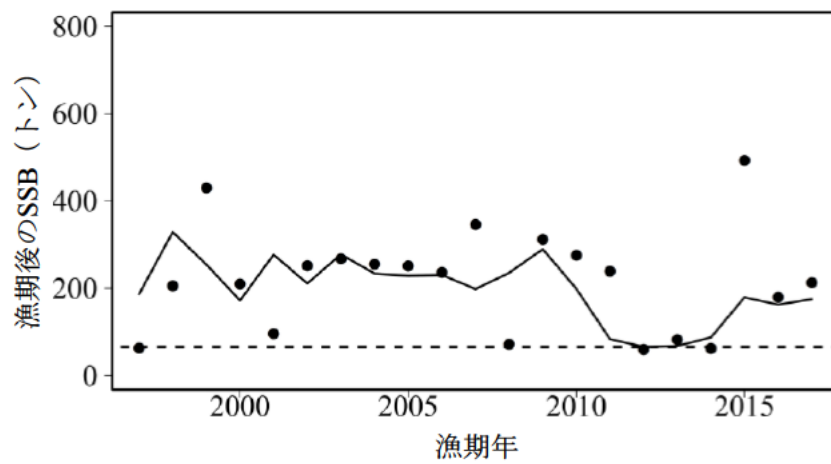
補足図 5-4. トロール調査から予測された漁期後の SSB（黒点）と JASAM によって推定された漁期後の SSB の事後分布の中央値（黒実線）。
