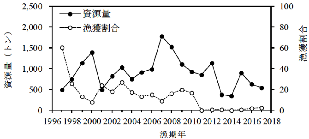
図 12. 面積－密度法により得られた資源量と漁獲割合の経年変化
