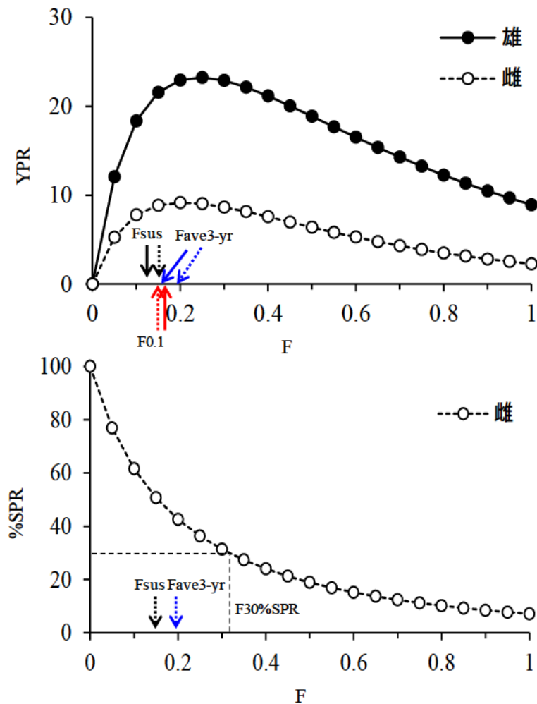
図 17. 雌雄別の F 値と YPR および %SPR の関係
