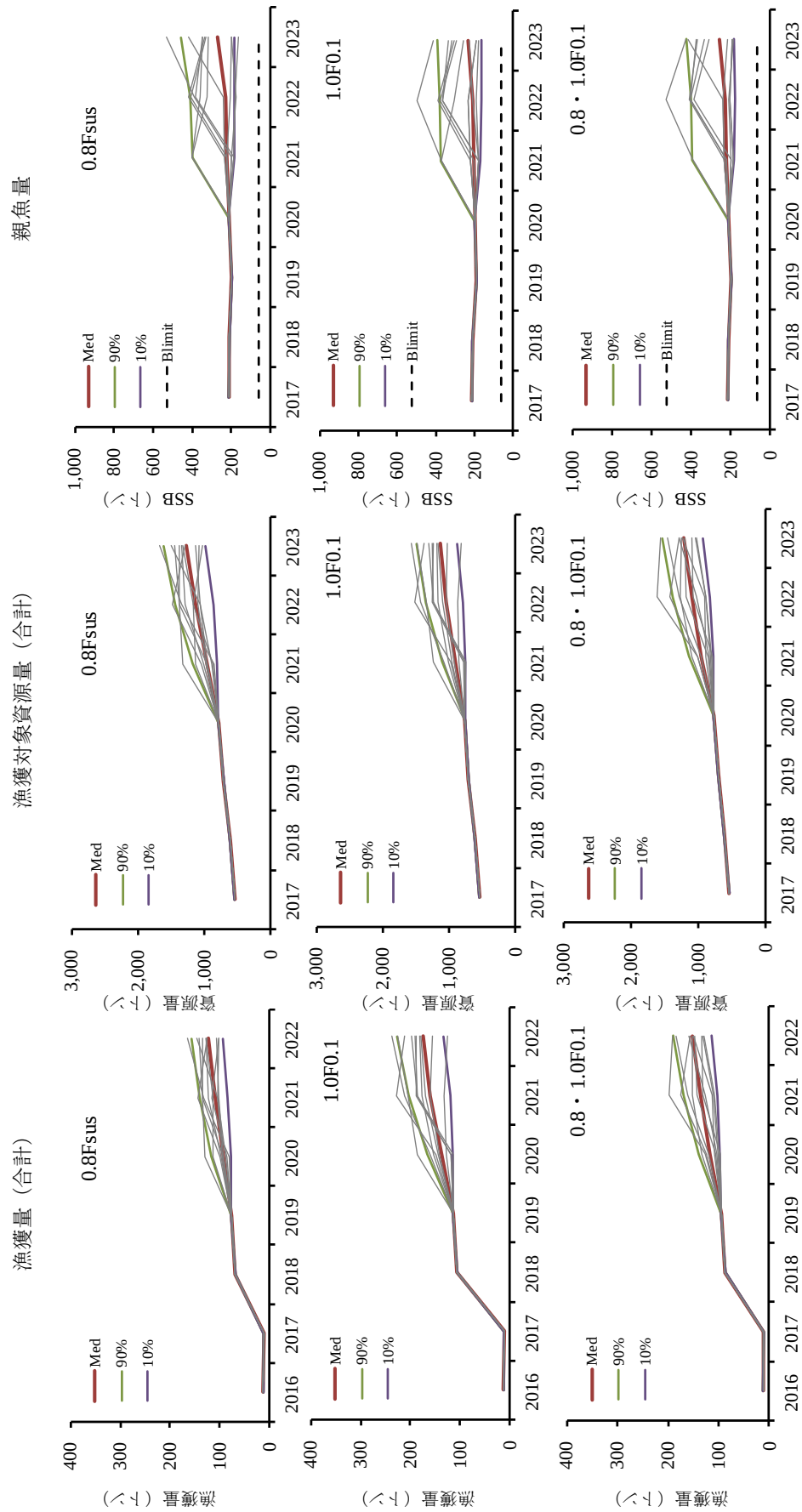
図 20. 加入量の不確実性を考慮したシミュレーションにより得られた漁獲量、資源量および漁期後の親魚量 (SSB) の推移 0.8F sus 、0.8F 0.1 、0.8 * 0.8F 0.1 のケースを示す。
