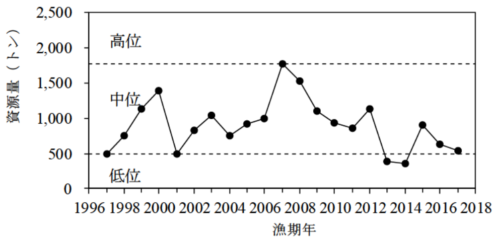
図 15. 資源量と水準の判定基準との関係
