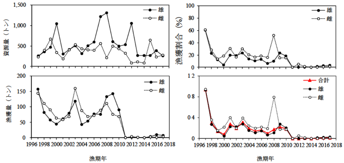
図 13. 雌雄別の資源量、漁獲量、漁獲割合および F 値の推移
