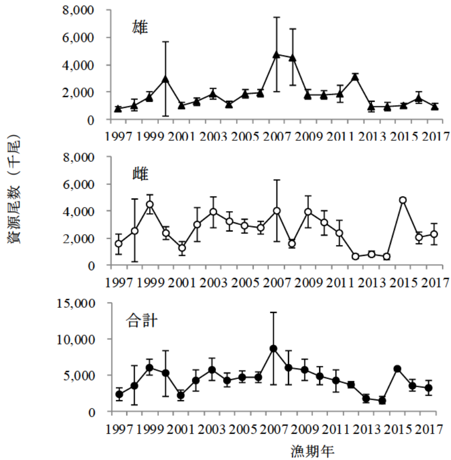
図 11. トロール調査で推定されたズワイガニの資源尾数 バーは 95%信頼区間を示す。
