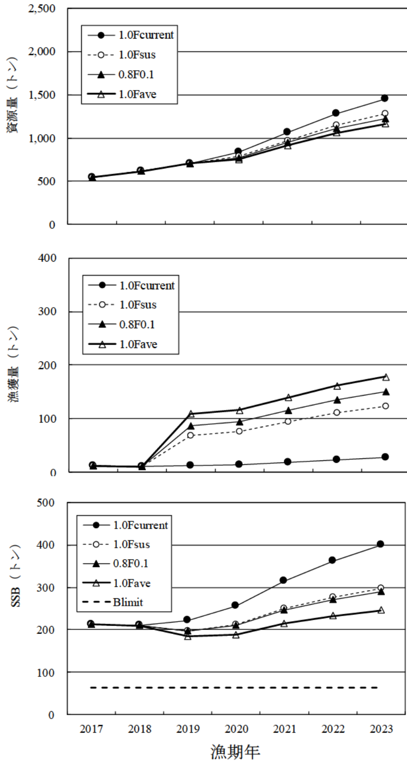
図 18. 各々のシナリオにより得られた漁獲量、資源量および漁期後の親魚量 (SSB) の推移
