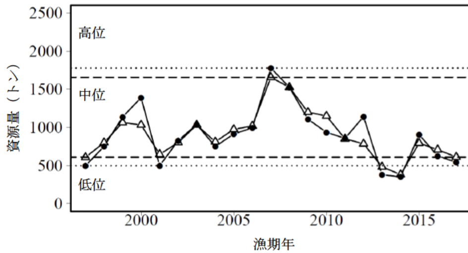
補足図 5-3. トロール調査から推定された資源量（黒点）とその水準境界（短破線）および JASAM によって推定された資源量（三角）とその水準境界（長破線）。
