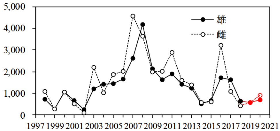
図 16. 加入量の推定値（2018 年以前の値）および予測値（2019～2020 年）の推移
