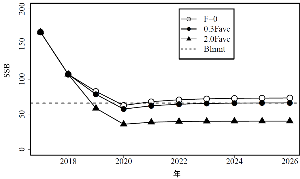
補足図 5-5. JASAM で得られたパラメータを使った将来予測による漁期後の SSB 漁獲なし ( F=0 ) のとき (白丸)、2023 年漁期終了時点で B_{limit} を上回る F ( 0.3F_{ave3-yr} ) での漁獲 (黒丸)、本評価で 0.8F_{0.1} で得られる漁獲量 (86.3 トン) を 2019 年漁期に実現させる F ( 2.0F_{ave3-yr} ) で漁獲 (黒三角) したときの予測結果。
