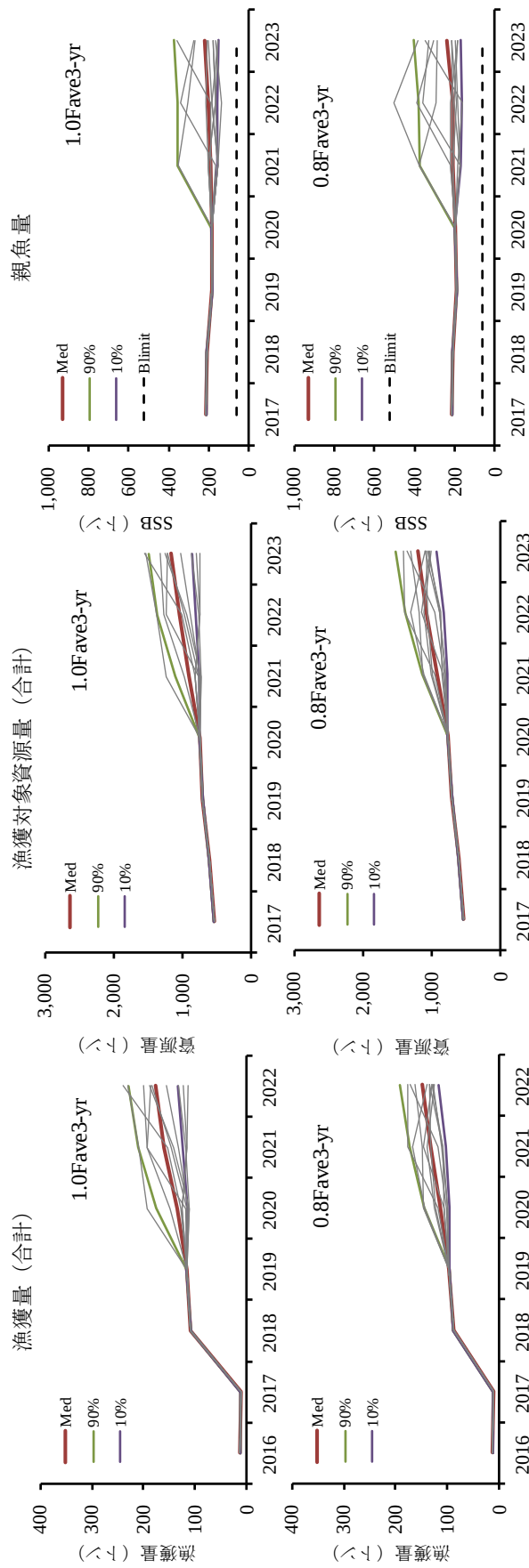
図 21. 加入量の不確実性を考慮したシミュレーションにより得られた漁獲量、資源量および漁期後の親魚量 (SSB) の推移 1.0Fave3-yr、0.8Fave3-yr のケースを示す。
