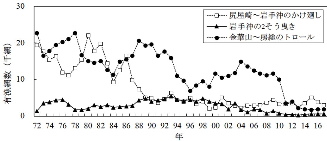
図6. 沖底による漁獲努力量の経年変化 2017年の値は暫定値である。
