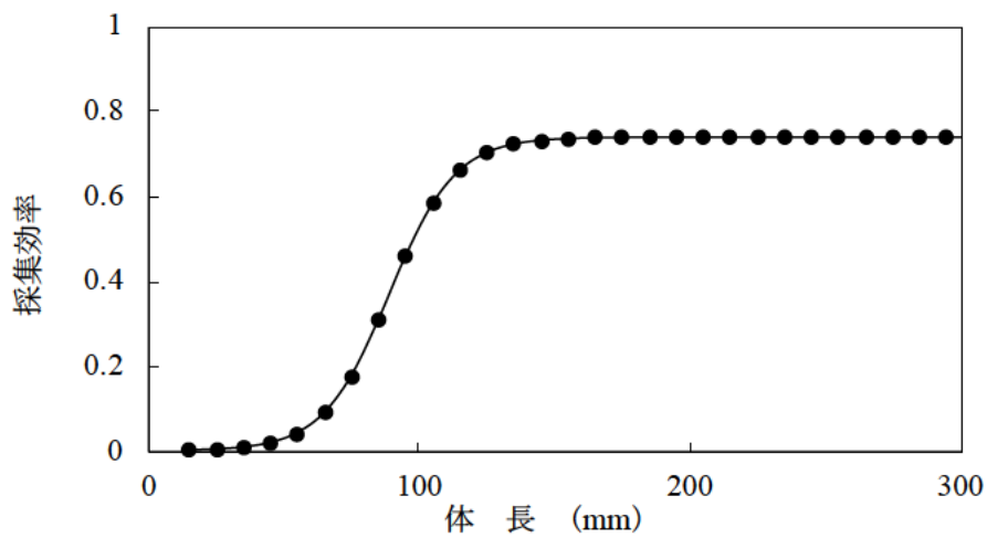
図7. 体長と採集効率の関係
