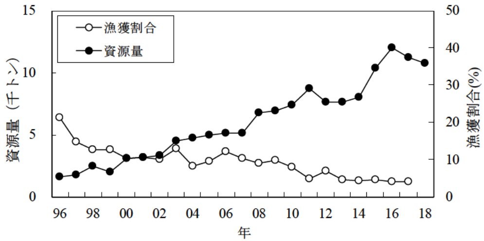
図10. キチジの資源量（1月時点）および漁獲割合の推移
