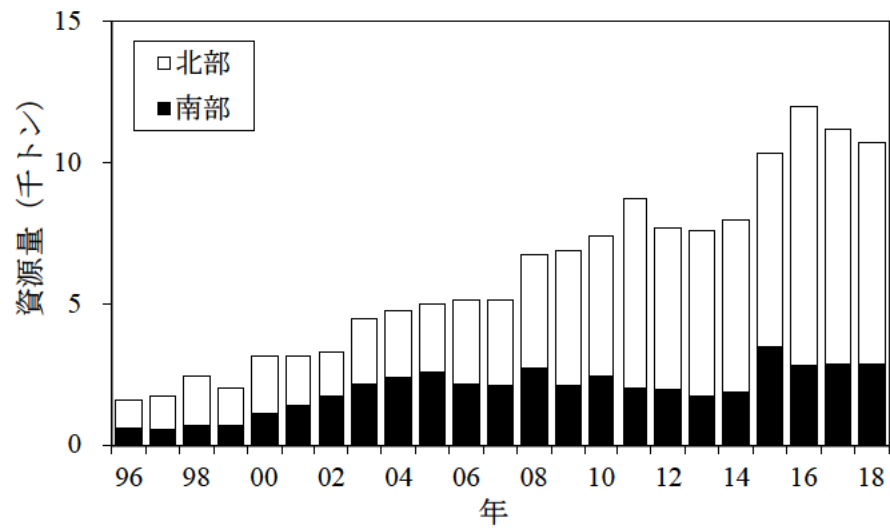
補足図3-3. 太平洋北部の南北別のキチジの資源量（1月時点） Logistic式から得られた採集効率を用いた。
