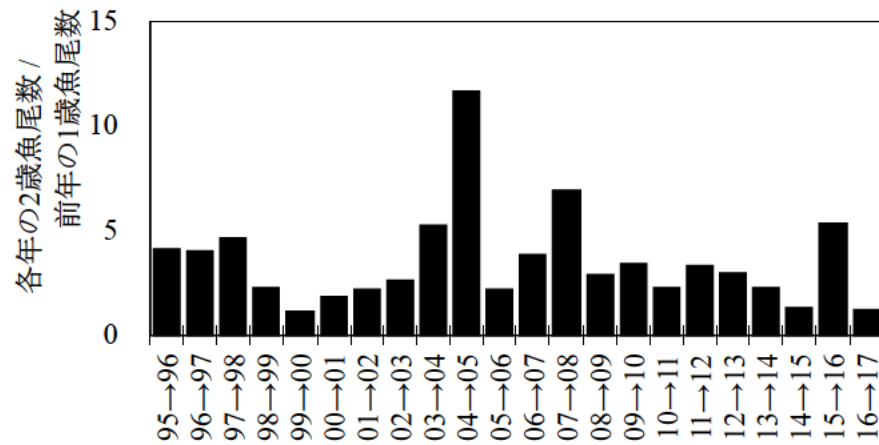
補足図4-1. 採集効率を一定の1とした場合の各年の2歳魚尾数と前年の1歳魚尾数の比率
