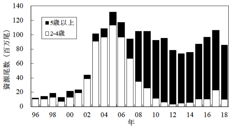
図11. キチジの資源尾数（1月時点）の推移
