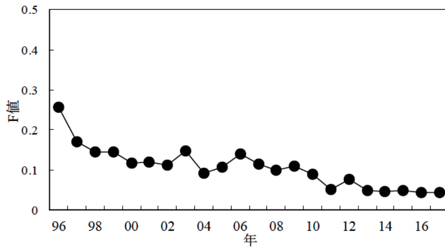
図12. F値の経年推移
