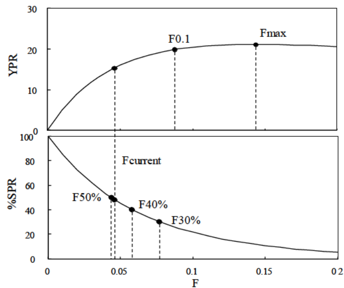
図17. 様々なFとYPR曲線および%SPR曲線との関係
