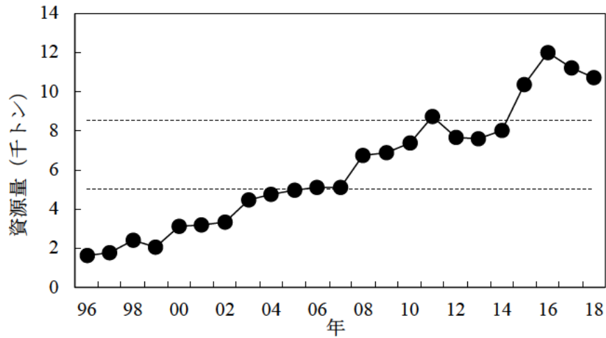
図16. キチジの資源量 (1月時点) の推移 破線は水準の境界を示す。
