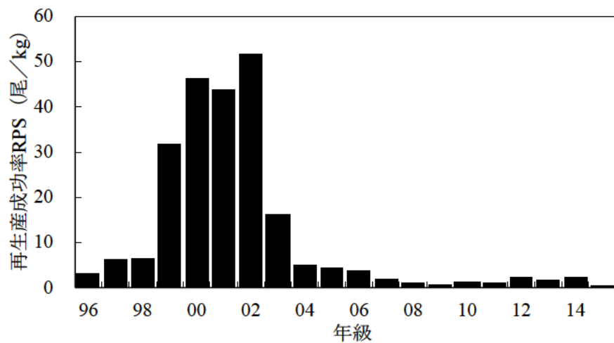
図13. 再生産成功率 (RPS) の推移
