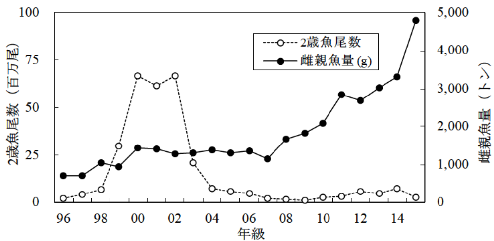
図14. 雌親魚量と加入量の推移
