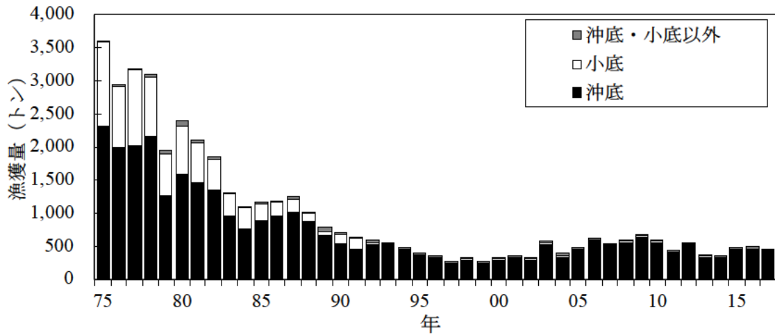
図5. 太平洋北部におけるキチジ漁獲量の推移
