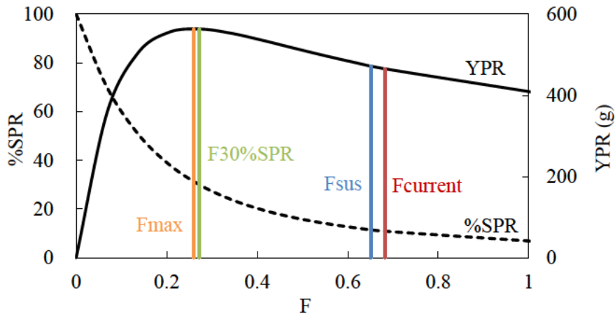
図 20. 漁獲係数(F)と%SPR、YPR の関係
