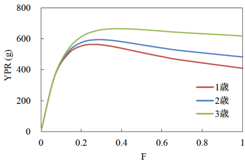
図 22. 漁獲開始年齢別の漁獲係数(F)と YPR の関係 現状は漁獲開始年齢 1 歳、 F=0.68 。
