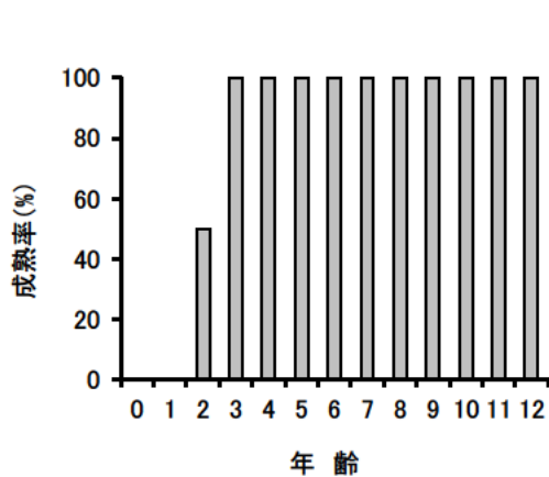
図3. ヒラメ日本海西部・東シナ海系群の年齢別成熟率
