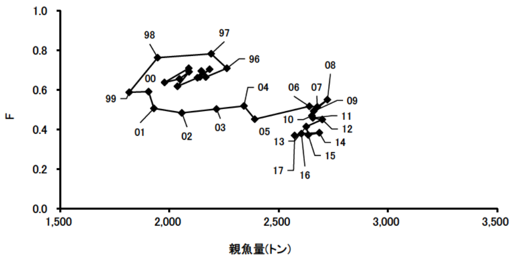
図 15. 親魚量と漁獲係数 F の関係
