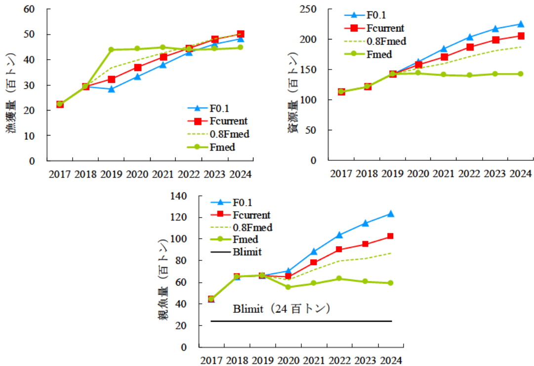
図 14. 様々な F による漁獲量 (左上)、資源量 (右上)、親魚量 (下) の予測
