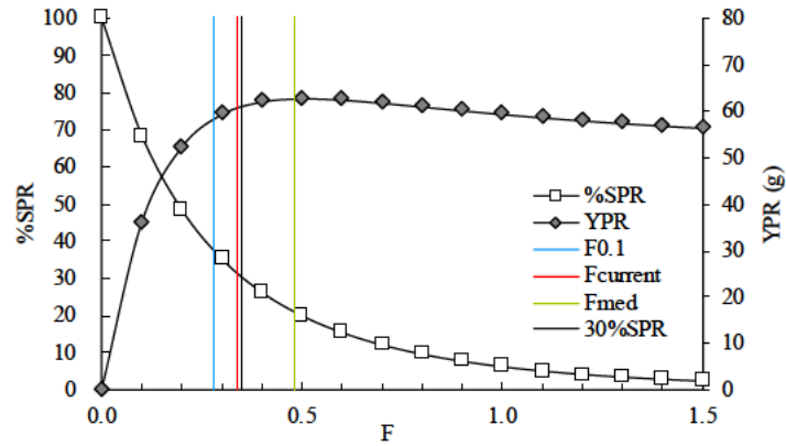
図 13. %SPR、YPR と F の関係
