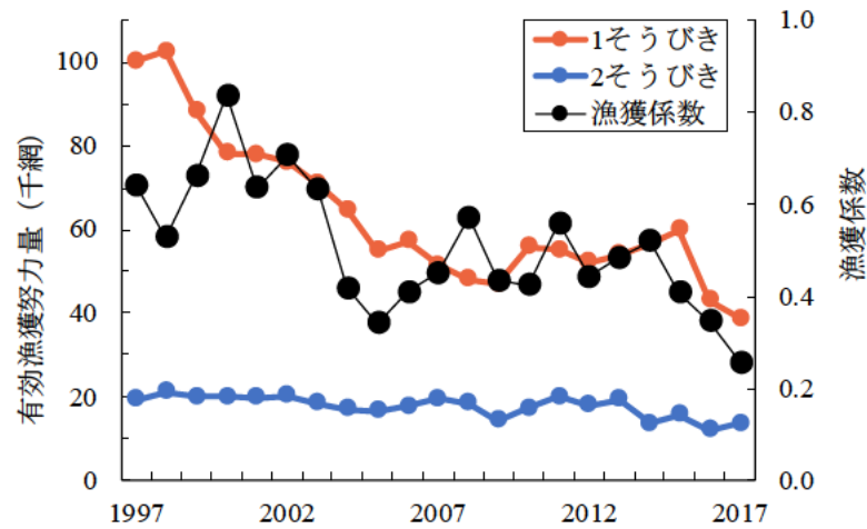
図 12. 漁獲係数と有効漁獲努力量の推移 漁獲係数は各年齢の F 値の単純平均。
