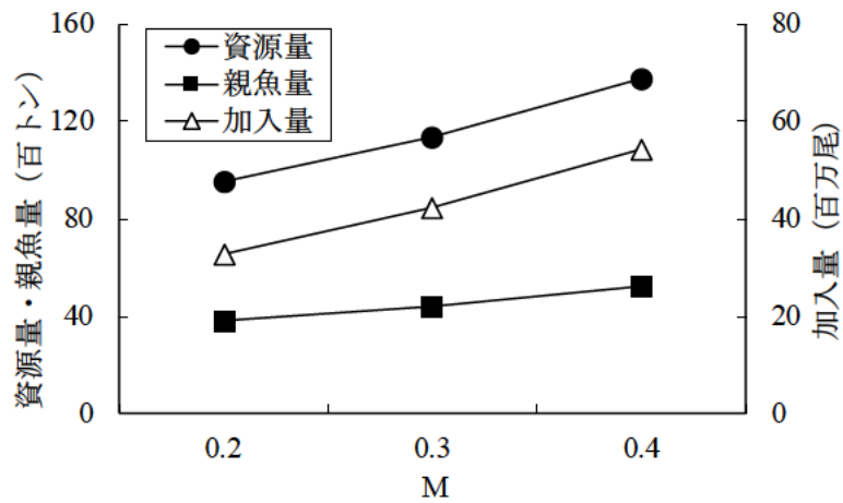
図 11. M と 2017 年資源量、親魚量、加入量（1 歳魚）の関係
