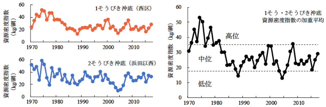
図 5. 沖合底びき網データから推定した資源密度指数の推移
