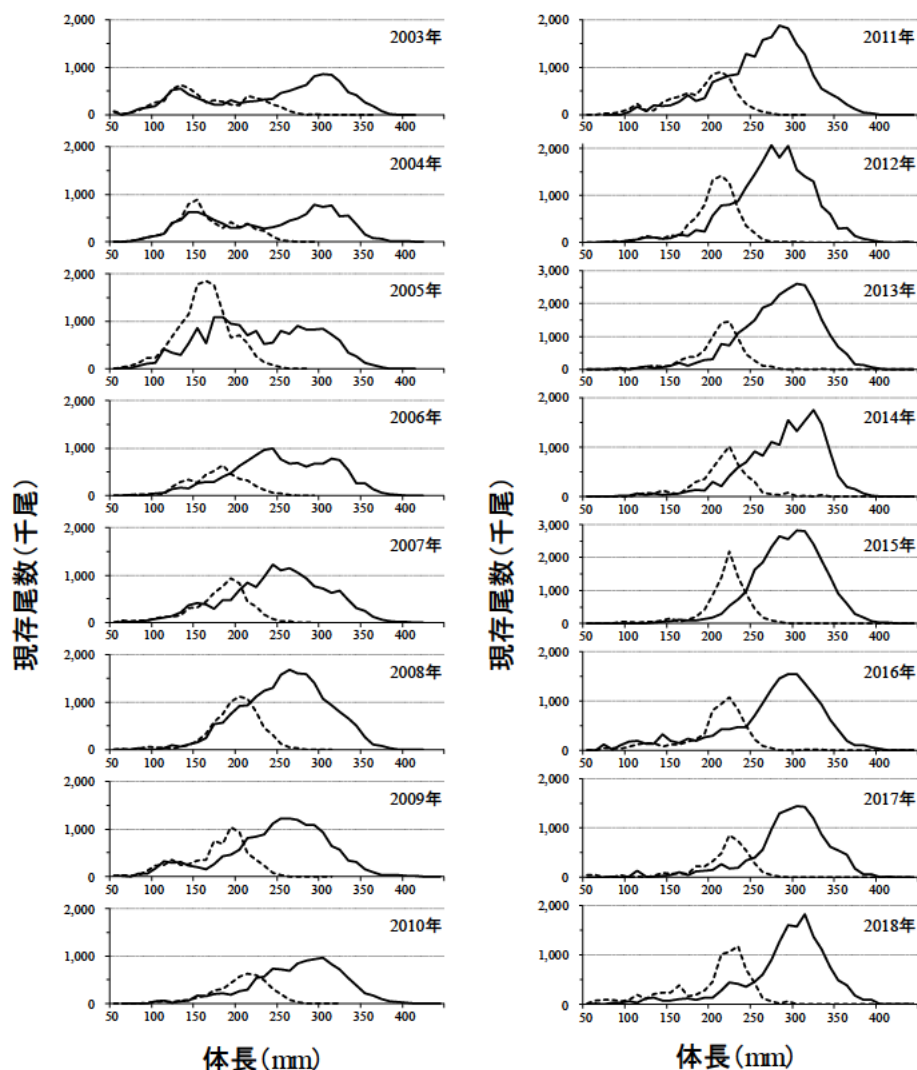
図9. ズワイガニ等底魚資源調査（但州丸）に基づく日本海西部におけるアカガレイの体長組成 実線は雌、破線は雄。
