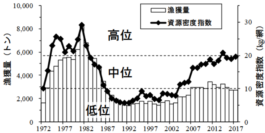
図 4. 日本海における沖底（1 そうびき）の漁獲量と資源密度指数 破線は水準の区分であり、資源密度指数 20（高一中）、10（中一低）。
