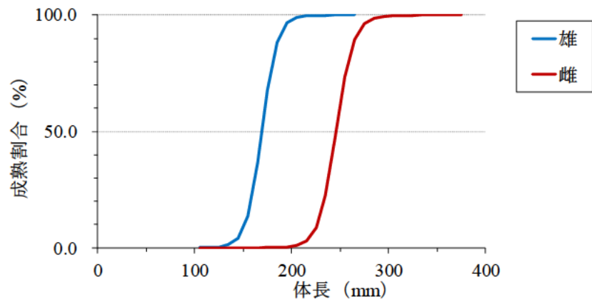
図 3. 日本海（京都府沖）におけるアカガレイの体長と群成熟率の関係（藤原ほか 2009）
