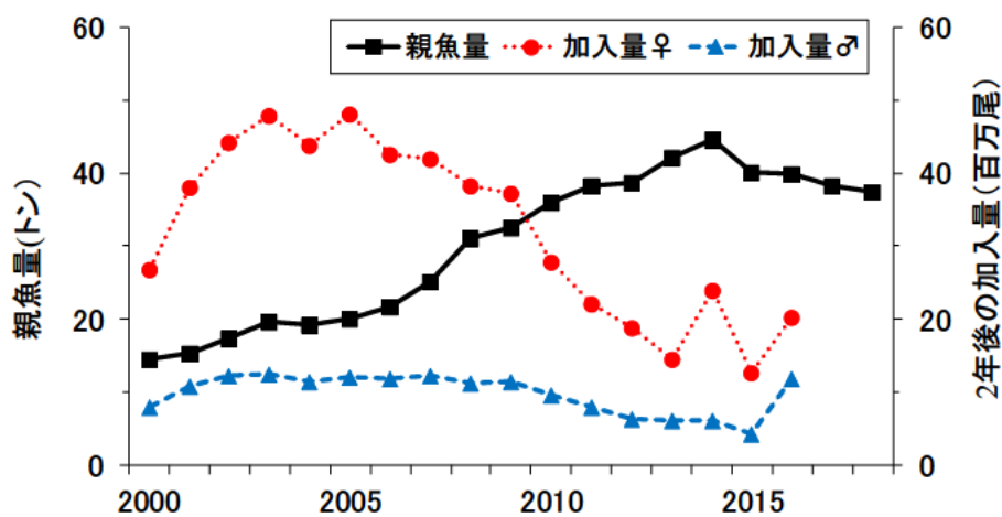
補足図 3-4. 親魚量（雌のみ）と2年後の雌雄別加入量
