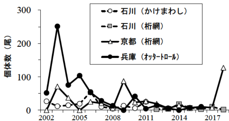
図10. 3府県における新規加入量調査結果に基づく小型個体（体長100～150mm（2歳魚））の単位努力量あたり採集数 石川県はかけまわし1曳網あたりおよび2012年以降は桁網1曳網あたり、京都府は桁網10曳網あたり、兵庫県はオッターロール5曳網あたりの採集個体数に、それぞれ換算。
