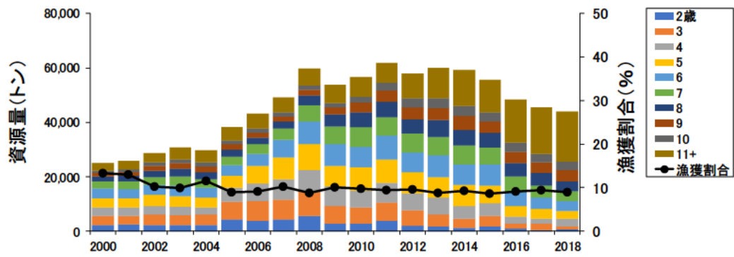
補足図 3-2. 資源量（雌雄合計）と漁獲割合
