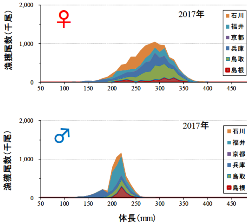
図 8. 日本海西部における 2017 年の漁獲物の雌雄別および府県別の体長組成
