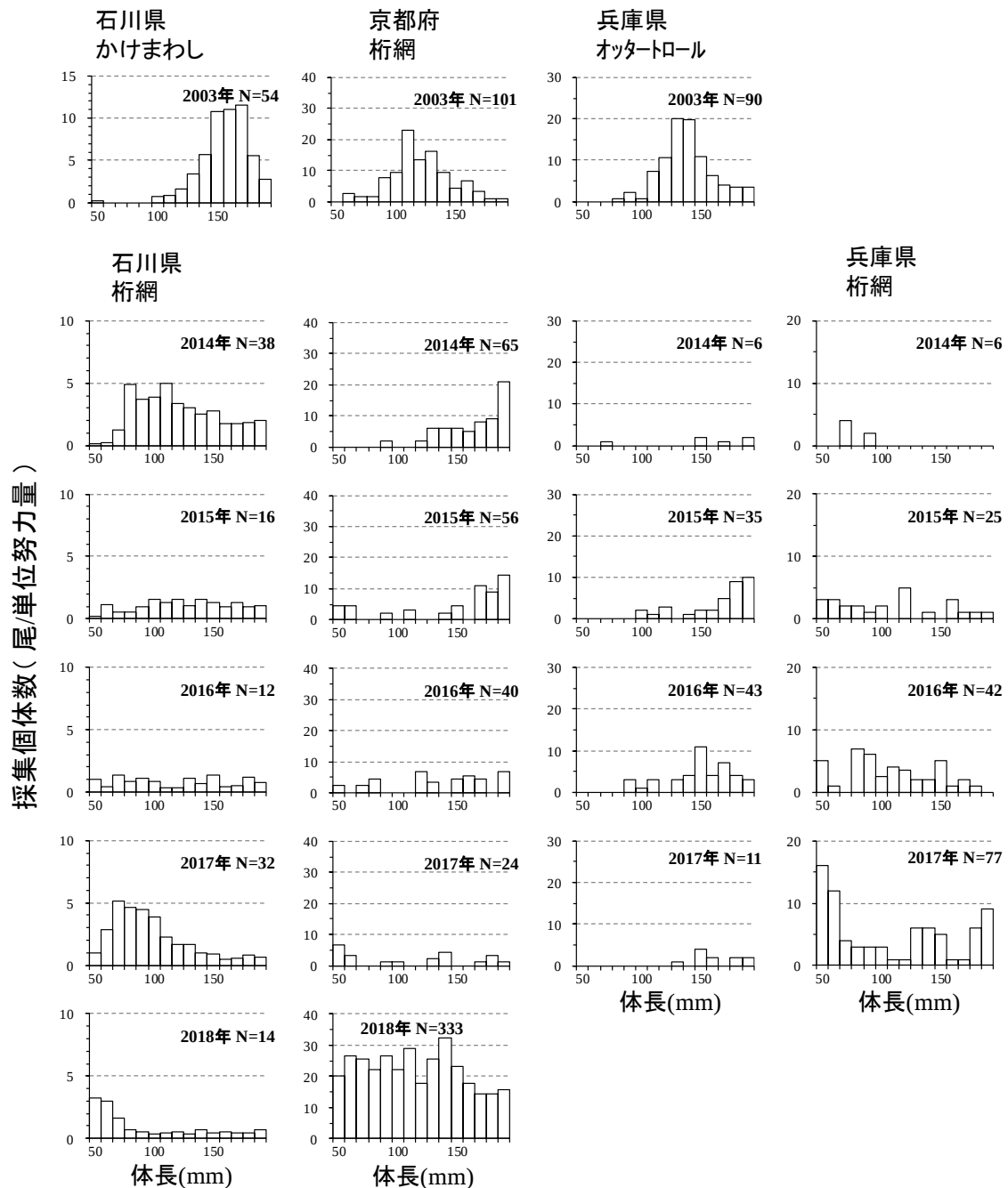
図 11. 3 府県の新規加入量調査に基づく体長組成 (2003 年、2014～2018 年)
