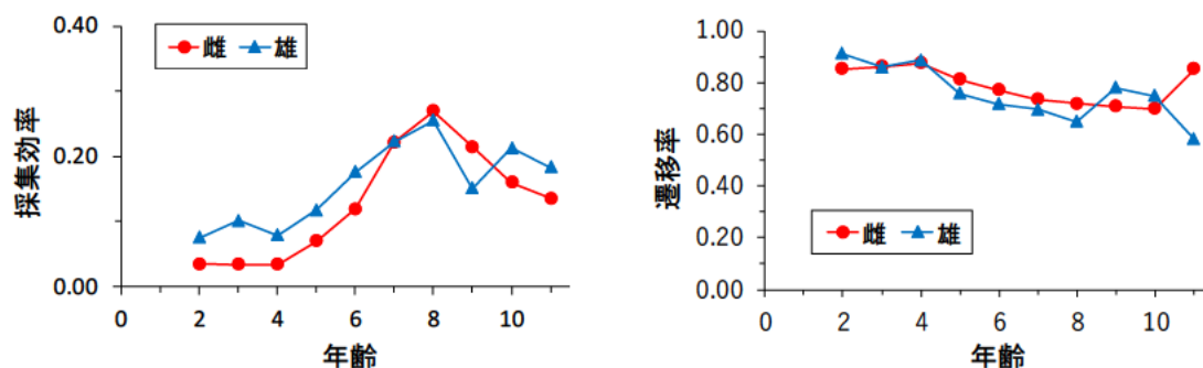
補足図 3-1. 雌雄別年齢別の採集効率と遷移率
