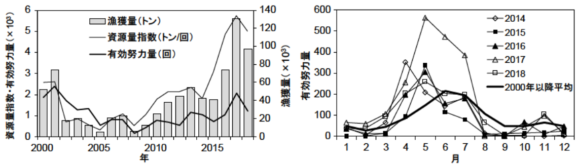
図 5. 北部まき網の有効努力量と漁獲量、資源量指数の推移 (JAFIC 集計値、道東含まず) 努力量＝投網数、資源量指数＝ \sum 緯度経度 30 分単位メッシュの CPUE、有効努力量 ＝漁獲量／資源密度指数、資源密度指数＝資源量指数／有漁メッシュ数。
