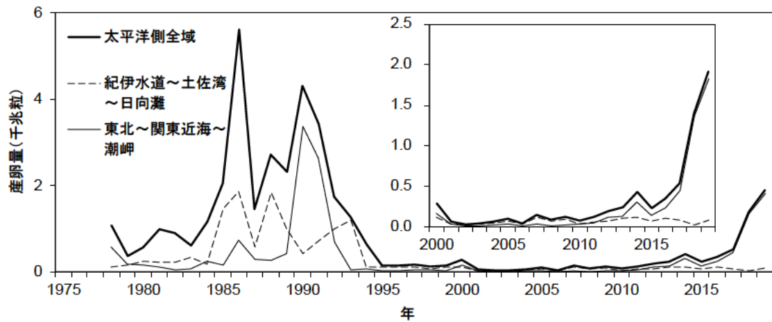
図 7. 産卵量の推移 卵稚仔調査協議会による前年 10 月から 9 月までの集計値。2019 年は 5 月までの暫定値。太平洋側全域は同協議会の区分の海区Ⅰ～Ⅳ、紀伊水道～土佐湾～日向灘は海区Ⅲ、東北～関東近海～潮岬は海区Ⅰ・Ⅱの値。
