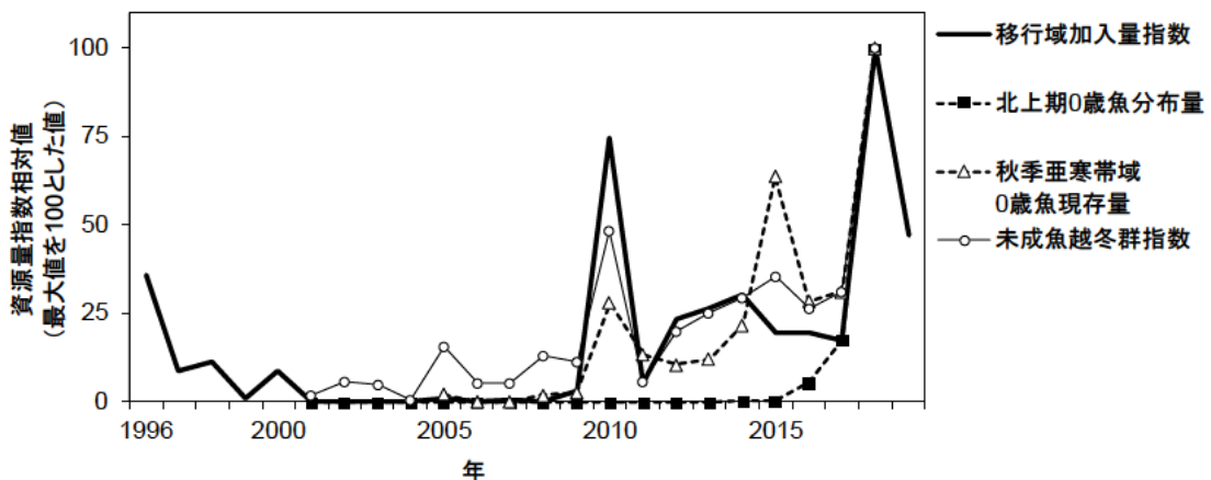
図 8. 加入量の指標となる資源量指数の推移 各指数については補足資料 3 を参照。未成魚越冬群指数は前年の加入量と対応するので 1 年ずらし、2002 年以降を示した。2018 年以降の移行域加入量指数は、前年までと調査時期が異なるため比較には注意が必要。
