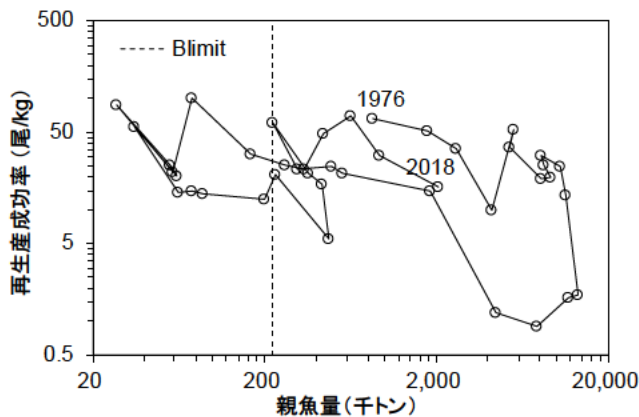
補足図 5-1. 親魚量と RPS の関係
