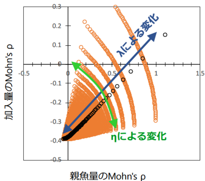
補足図 2-1. 親魚量と加入量のレトロスペクティブバイアスの関係 黒丸は、通常のリッジ VPA で \lambda を変化させたもの。オレンジの丸は、0 歳と 1 歳以上でペナルティの重みを変えたリッジ VPA で \lambda と \eta を変化させたもの。
