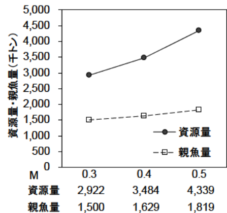
図12. 自然死亡率 M と資源量、親魚量の関係 M の変化に対する2018年の推定値の感度解析。
