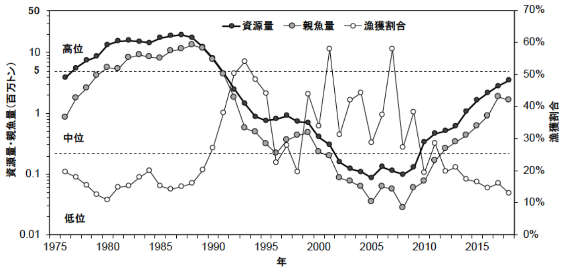
図10. 資源量、親魚量および漁獲割合の推移 図中破線は資源水準区分の親魚量の目安。
