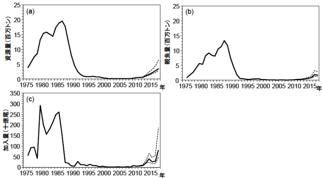
補足図 2-2. (a) 資源量、(b) 親魚量、(c) 加入量の推定値と 80%信頼区間。実線が推定値、破線が信頼区間を示す。
