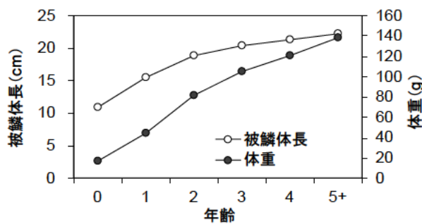
図 2. 年齢と成長 (2016～2018 年漁獲物平均値)
