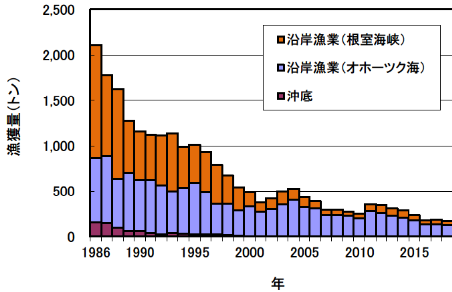
図 3. キチジオホーツク海系群の漁獲量の推移 2018 年は暫定値。
