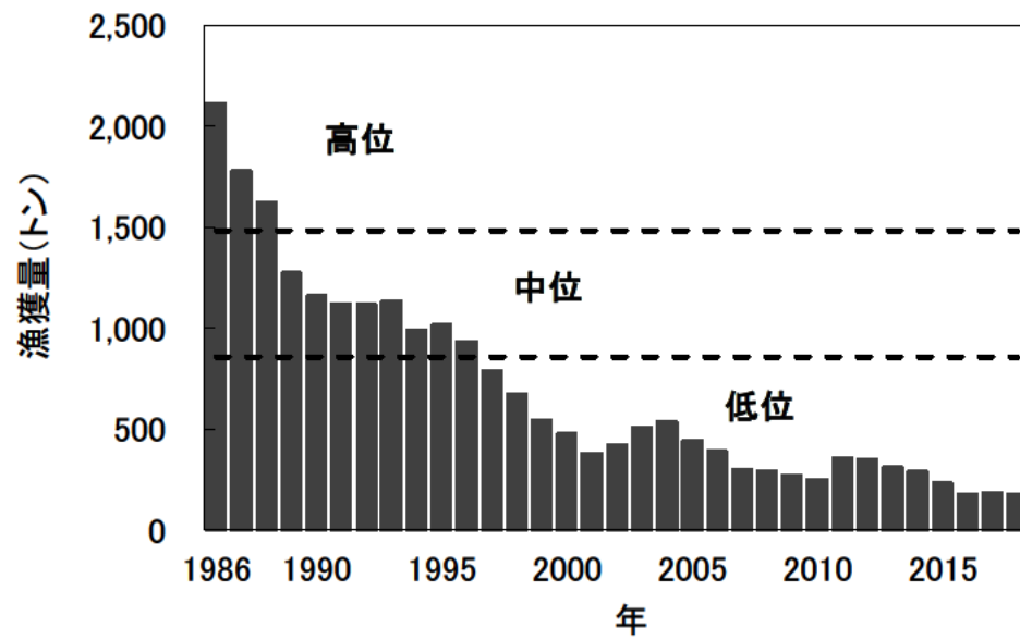
図 5. キチジオホーツク海系群の漁獲量の推移と資源水準の判断
