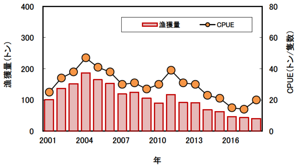
図 4. オホーツク海における延縄漁業の漁獲量と CPUE（資源量指標値）の推移 2018 年は暫定値。（網走水産試験場 印刷中を改変）
