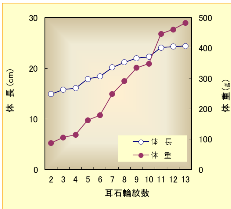
図2. オホーツク海におけるキチジの耳石輪紋数と体長、体重の関係（城 2010）
