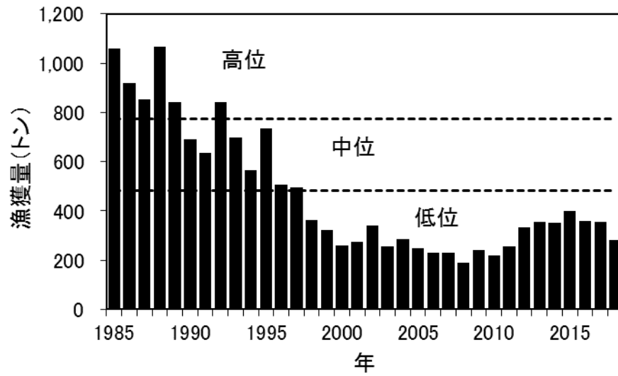
図 7. キチジ道東・道南の資源水準の判断
