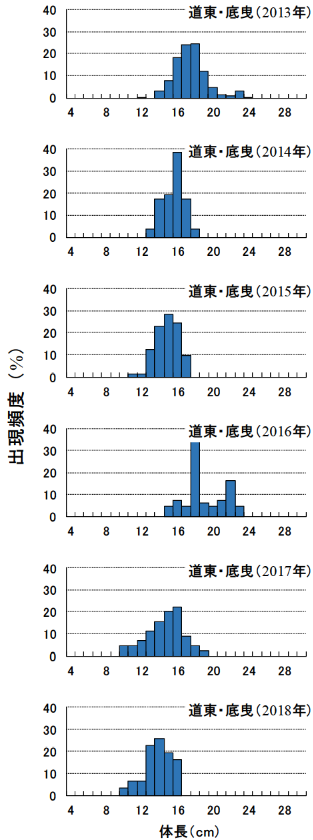
図 5. 道東海域におけるキチジ漁獲物の体長組成（底曳は沖底とえびこぎ網を含む）
