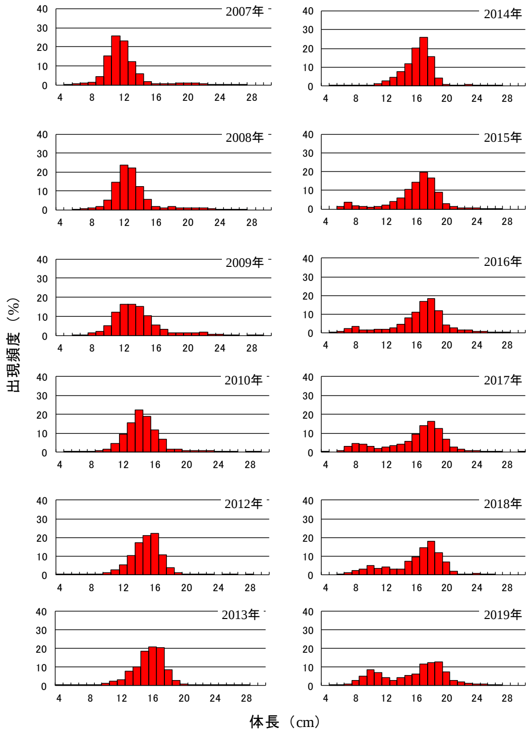
図 6. 着底トロール調査で採集されたキチジの体長組成 (2011 年は欠測)
