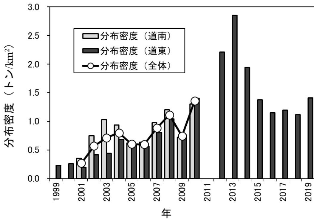
図 4. 着底トロール調査によるキチジの分布密度推定値の推移
