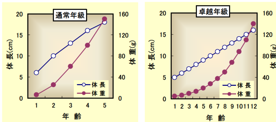
図 2. キチジの年齢と体長・体重の関係
