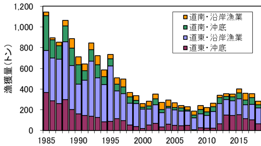
図 3. キチジ道東・道南の漁獲量の推移
