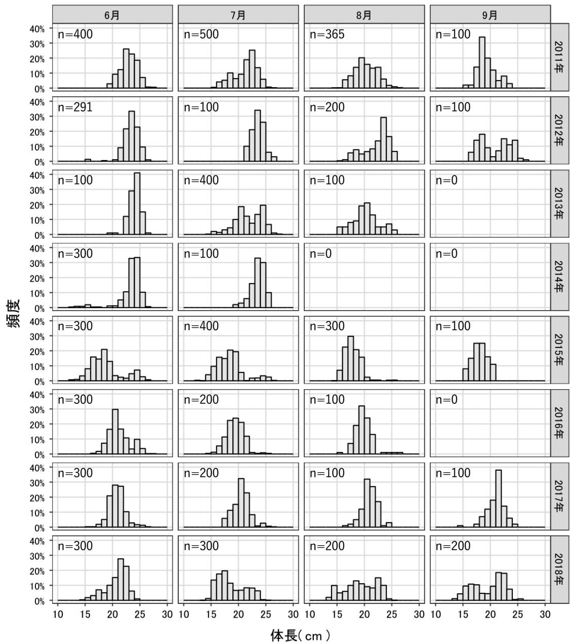
図6. 宗谷海峡周辺において沖底により漁獲されたイカナゴ類の6～9月の体長組成（稚内水産試験場 未発表資料）
