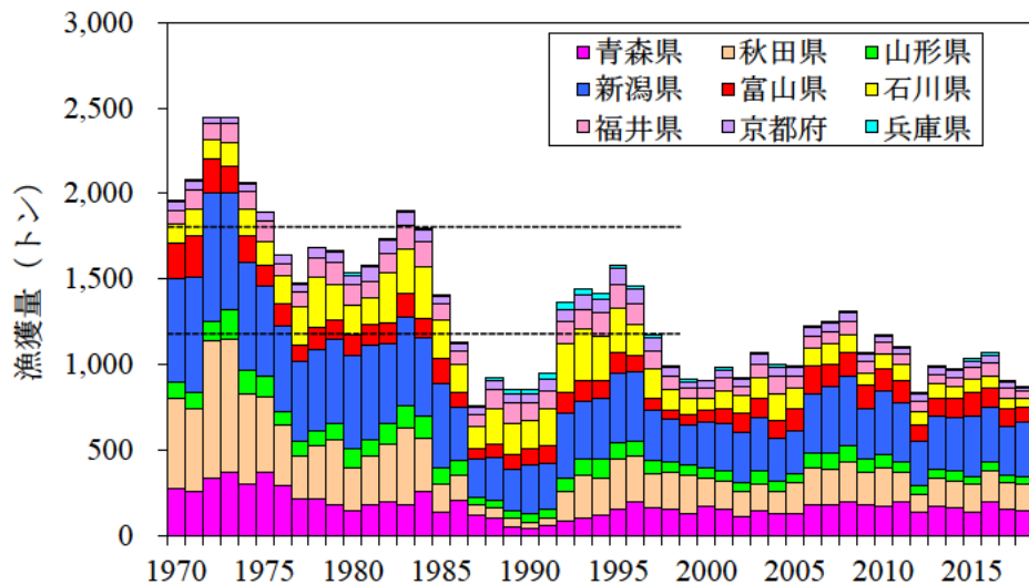
図 6. 漁獲量の経年変化（農林統計、ただし青森県は県統計）
