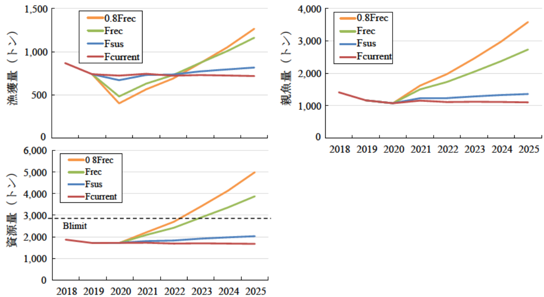
図 21. 様々な F による漁獲量(左上)と資源量(下)および親魚量 (右上) の推移
