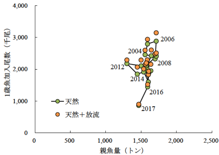
図 17. 親魚量と 1 歳魚加入尾数の関係
