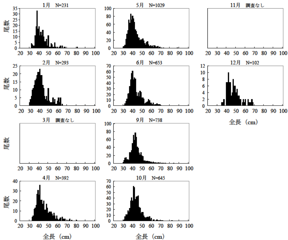
図 9. 新潟県岩船港における漁獲物の全長組成（2018 年） 尾数は各月の調査尾数を示す。
