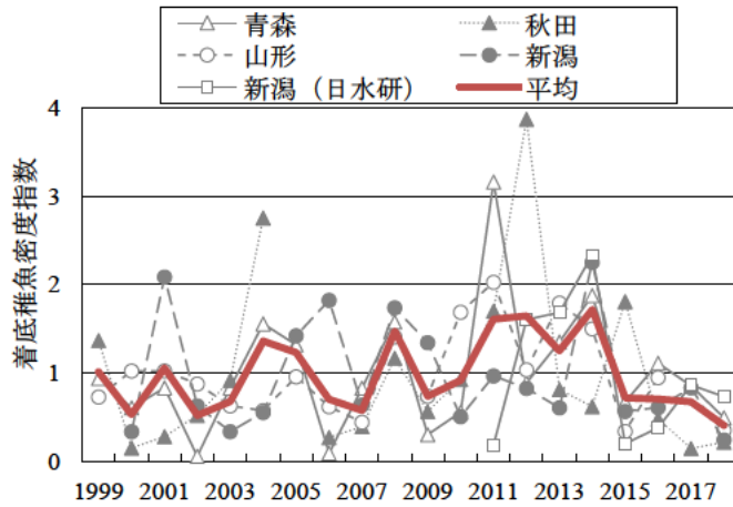
図 19. 着底稚魚密度指数の推移 各調査期間内の平均を 1 とする（各調査資料より計算）。
