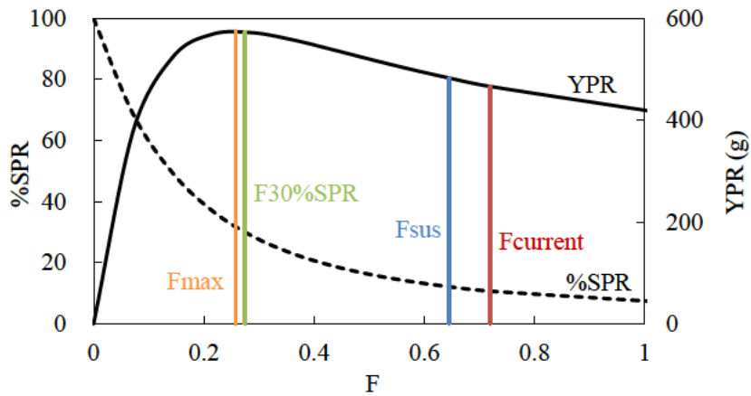
図 20. 漁獲係数(F)と%SPR、YPR の関係
