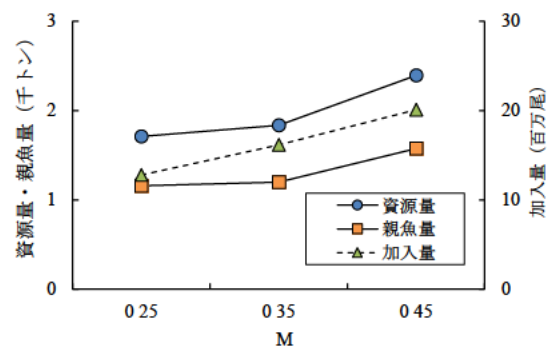
図 12. M と 2018 年資源量、親魚量、 加入量の関係
