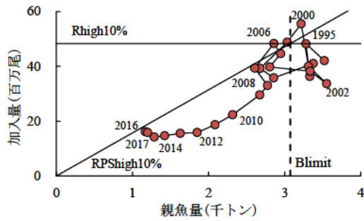
図 13. 親魚量と加入量（1 歳魚）の関係
