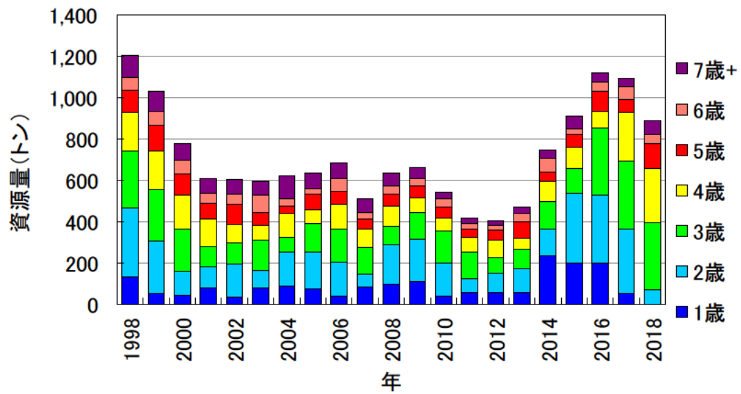
補足図 4-6. 標準化 CPUE によってチューニングした VPA によって求めた資源量
