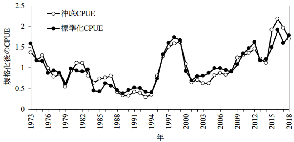
補足図 4-5. 沖底 CPUE と標準化 CPUE の時系列変化 それぞれ平均値で除すことで規格化した。
